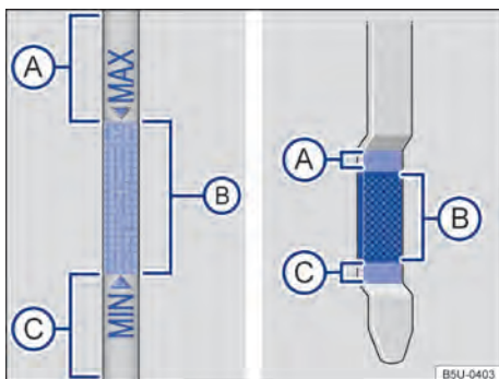
Fig. 173 Vareta de medição do óleo com marcas de nível do óleo do motor.
