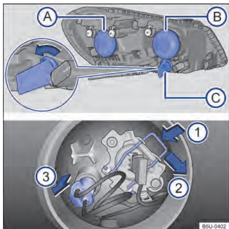
Fig. 154 No compartimento do motor: vista traseira do farol dianteiro com cobertura de borracha (lado esquerdo da ilustração) - A farol baixo, B farol alto e luz de posição, e C indicador de direção. Vista traseira do farol dianteiro sem a cobertura de borracha (lado direito da ilustração): 1 mola de travamento da lâmpada incandescente do farol e 2 luz de posição.
