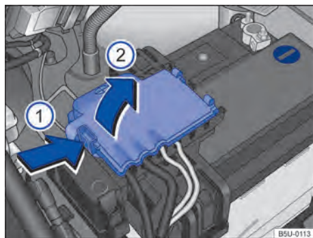
Fig. 122 Compartimento do motor: acesso ao terminal positivo da bateria.
