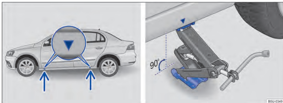
Fig. 143 Pontos de apoio do macaco e macaco posicionado no lado esquerdo traseiro do veículo.
