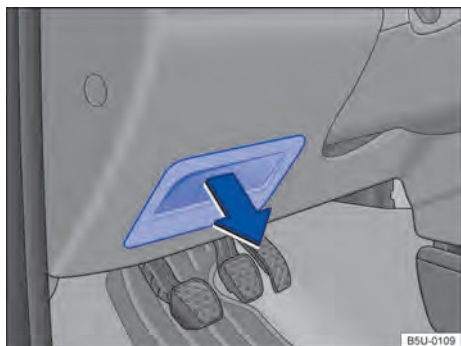
Fig. 116 No lado do condutor no painel de instrumentos: cobertura da caixa de fusíveis.
