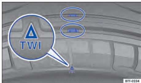
Fig. 137 Perfil do pneu: indicadores de desgaste.
