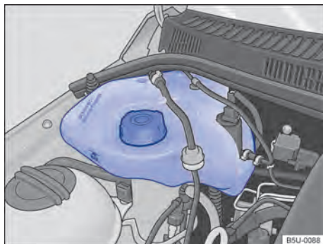
Fig. 132 No compartimento do motor: reservatório de gasolina para o sistema de partida a frio.
