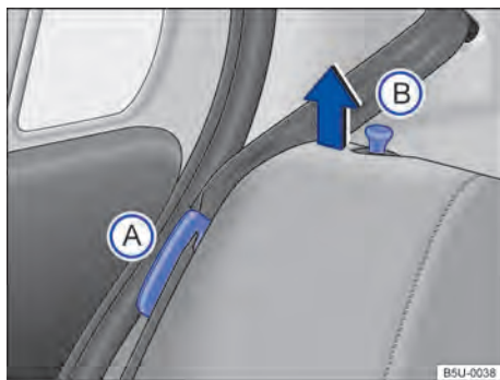
Fig. 57 Banco traseiro: posicionador do cinto de segurança (A) e pino de destravamento do encosto (B).
