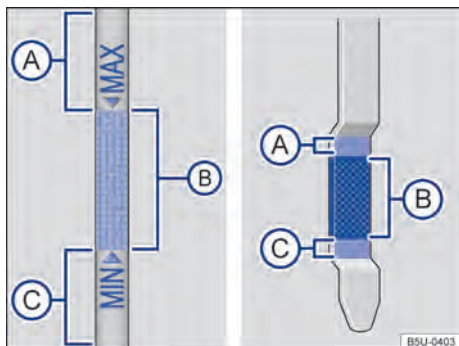
Fig. 127 Vareta de medição do óleo com marcas de nível do óleo do motor.
