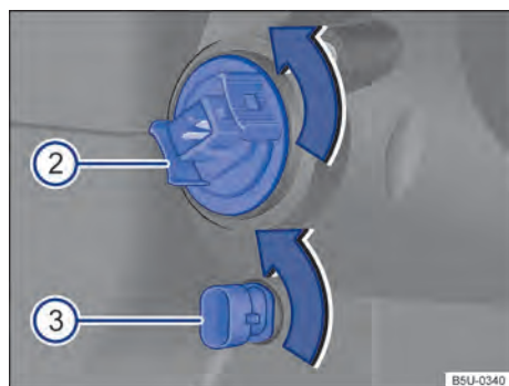
Fig. 109 No compartimento do motor: vista traseira do farol dianteiro (2) indicadores de direção e (3) luz de posição.
