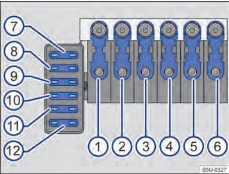
Fig. 119 Caixa de fusíveis.
