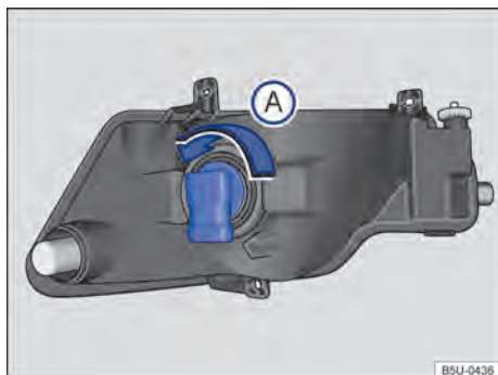
Fig. 110 Atrás do para-choque dianteiro: acesso à lâmpada incandescente do farol de neblina.
