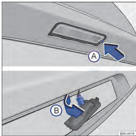
Fig. 115 No para-choque traseiro: remover a lanterna da placa de licença e o soquete da lâmpada.
