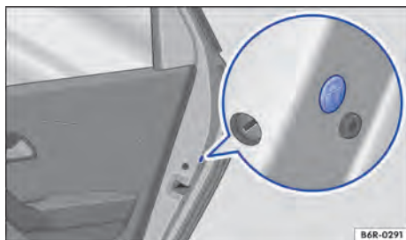
Fig. 49 Na porta traseira: travamento de emergência, coberto por uma vedação de borracha.
