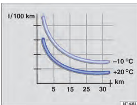
Fig. 80 Consumo de combustível em l/100 km em 2 temperaturas ambiente diferentes.
