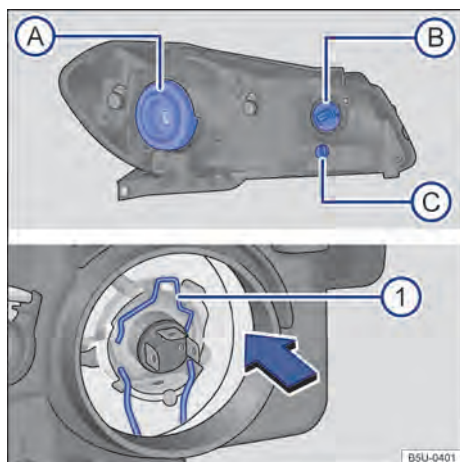
Fig. 108 No compartimento do motor: vista traseira do farol dianteiro com cobertura de borracha (lado esquerdo da ilustração) - (A) farol baixo / alto, (B) indicadores de direção e (C) luz de posição. Vista traseira do farol dianteiro sem a cobertura de borracha (lado direito da ilustração): (1) mola de travamento da lâmpada incandescente do farol baixo / alto.
