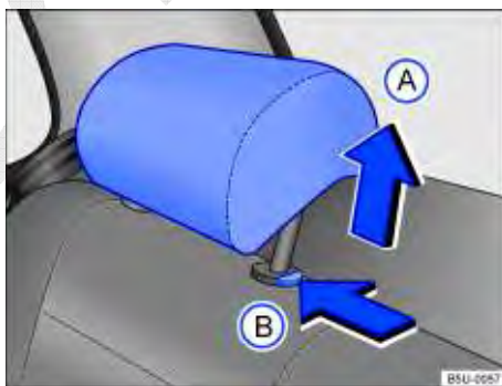
Fig. 43 Desinstalar o apoio para cabeça traseiro.
