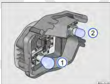
Fig. 186 No suporte das lâmpadas: localização das lâmpadas.
