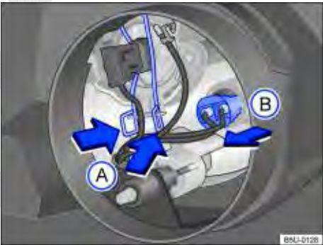
Fig. 179 Acesso à lâmpada incandescente do farol alto / luz de posição.
