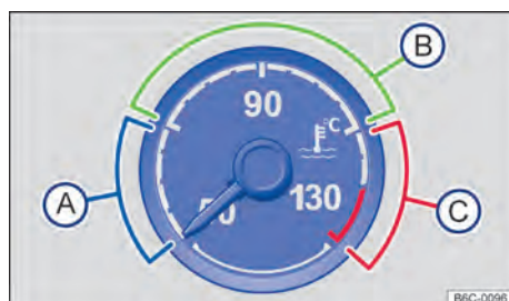
Fig. 14 Indicador de temperatura do líquido de arrefecimento do motor no instrumento combinado analógico: (A) área fria; (B) área normal; (C) área de advertência.
