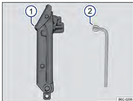
Fig. 159 Componentes das ferramentas de bordo.
