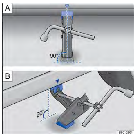
Fig. 202 Pontos de apoio do macaco e macaco posicionado no lado esquerdo traseiro do veículo.
