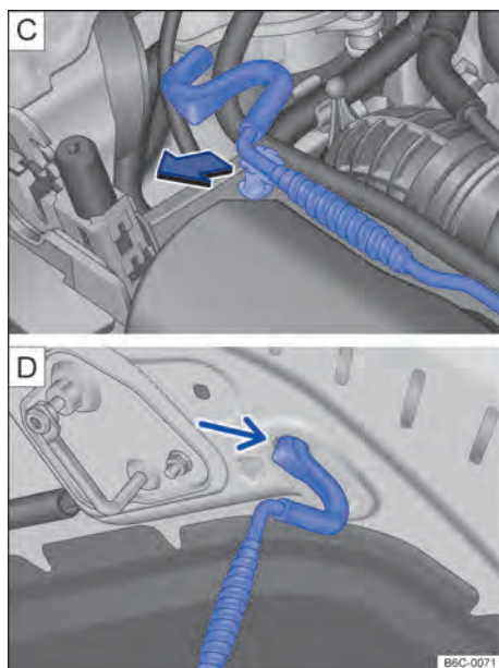
Fig. 183 [C] Haste de sustentação da tampa do compartimento do motor. [D] Tampa do compartimento do motor apoiada na haste de sustentação.
