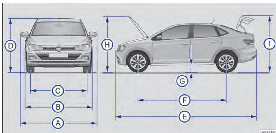
Fig. 208 Dimensões.
