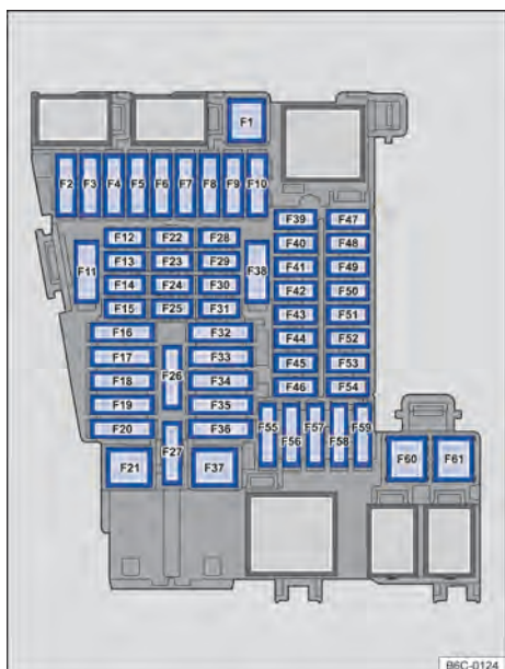
Fig. 174 No painel de instrumentos: disposição dos fusíveis.
