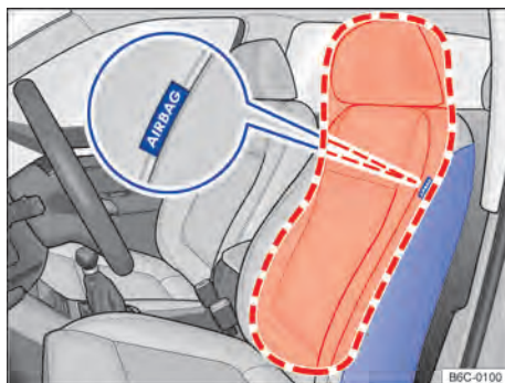
Fig. 39 Lateralmente no banco dianteiro: localização de instalação e área de expansão dos airbags laterais.
