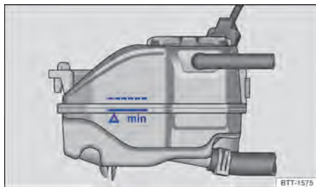
Fig. 188 No compartimento do motor: marcação no reservatório de expansão do líquido de arrefecimento do motor.
