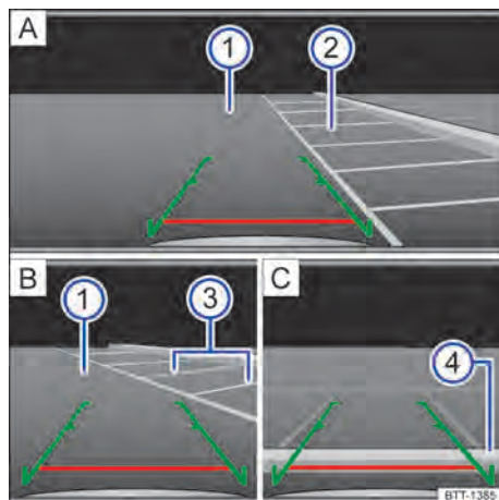
Fig. 99 Exibição do display do sistema do rádio: estacionar com a câmera de marcha a ré.
