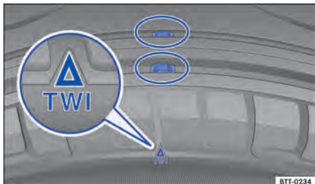
Fig. 196 Perfil do pneu: indicadores de desgaste.
