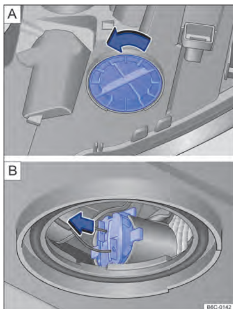
Fig. 164 Farol dianteiro, por baixo: cobertura do indicador de direção.
