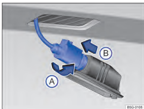
Fig. 172 Lanterna da placa de licença: desinstalar o suporte da lâmpada.
