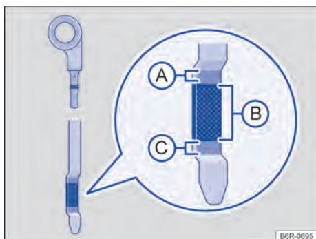
Fig. 186 Vareta de medição do óleo com marcas de nível do óleo do motor.
