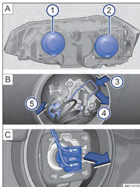
Fig. 163 No compartimento do motor: ❶ farol alto e luz de posição e ❷ farol baixo.
