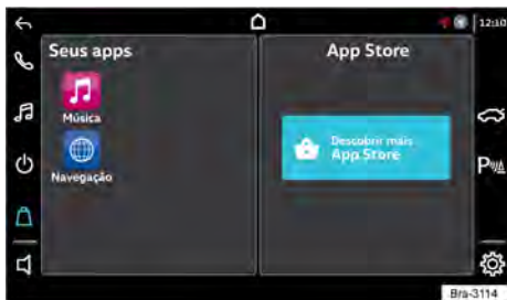
Fig. 144 App-store.
