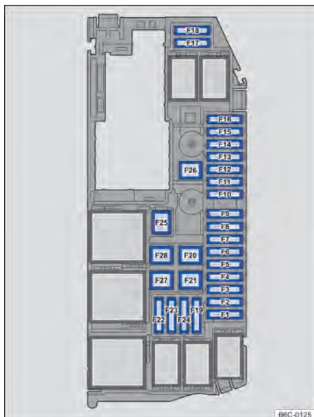
Fig. 177 No compartimento do motor: disposição dos fusíveis.
