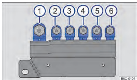
Fig. 178 No compartimento do motor em cima da bateria: disposição dos fusíveis.
