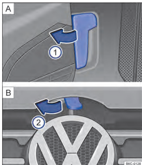
Fig. 183 [A] Alavanca de destravamento da tampa do compartimento do motor na área para os pés do lado do condutor. [B] Alavanca de destravamento na parte interna da tampa do compartimento do motor.
