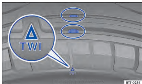
Fig. 197 Perfil do pneu: indicadores de desgaste.
