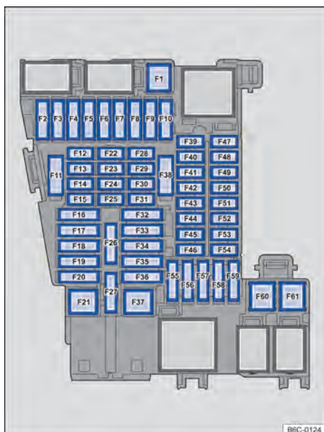
Fig. 175 No painel de instrumentos: disposição dos fusíveis.
