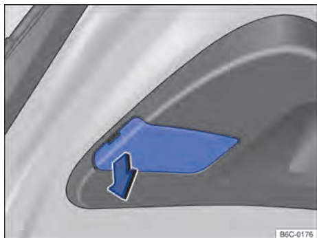
Fig. 170 Na tampa traseira: desmontar a cobertura da lanterna traseira.
