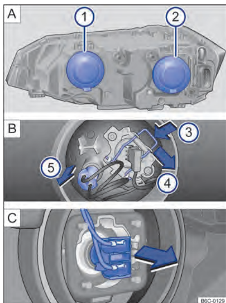
Fig. 164 No compartimento do motor: ⓘ farol alto e luz de posição e ⓘ farol baixo. ►
