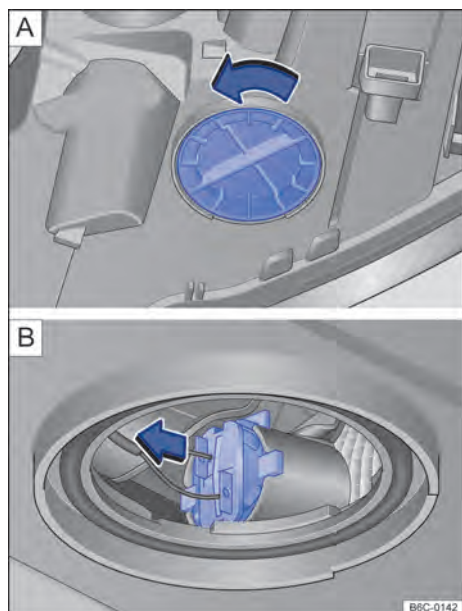
Fig. 165 Farol dianteiro, por baixo: cobertura do indicador de direção.
