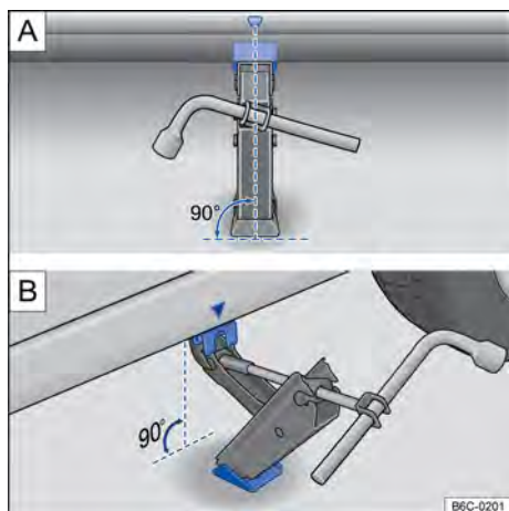
Fig. 203 Pontos de apoio do macaco e macaco posicionado no lado esquerdo traseiro do veículo.
