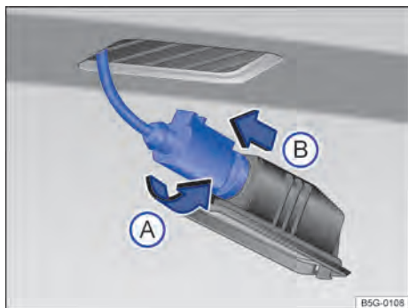
Fig. 173 Lanterna da placa de licença: desinstalar o suporte da lâmpada.
