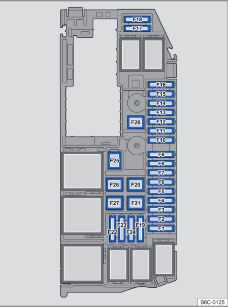
Fig. 142 No compartimento do motor: disposição dos fusíveis.
