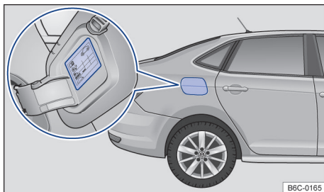
Fig. 160 Na parte interna da portinhola do tanque de combustível: etiqueta com a pressão dos pneus.
