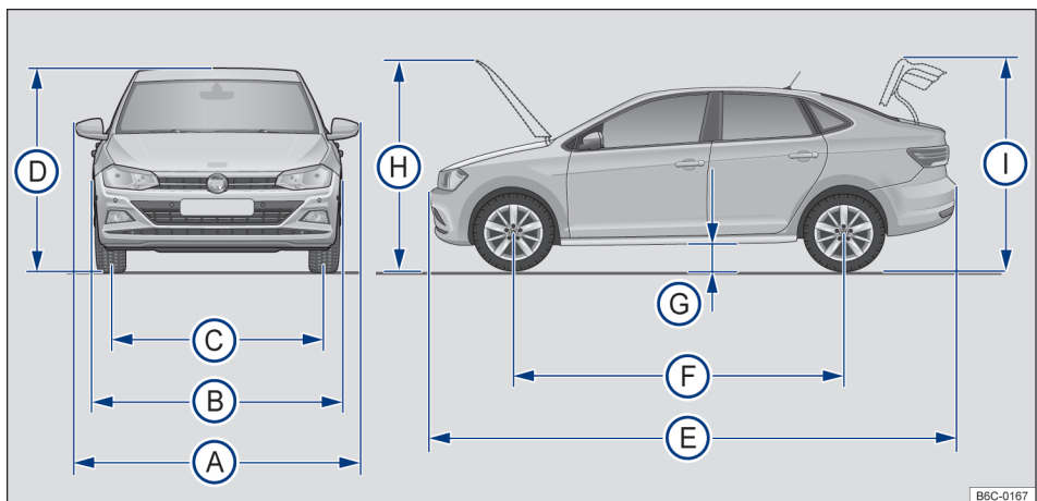
Fig. 176 Dimensões.
