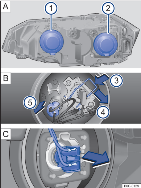
Fig. 129 No compartimento do motor: ⓘ farol alto e luz de posição e ⓘ farol baixo.
