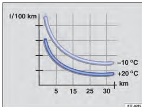
Fig. 77 Consumo de combustível em l/100 km em 2 temperaturas ambiente diferentes.
