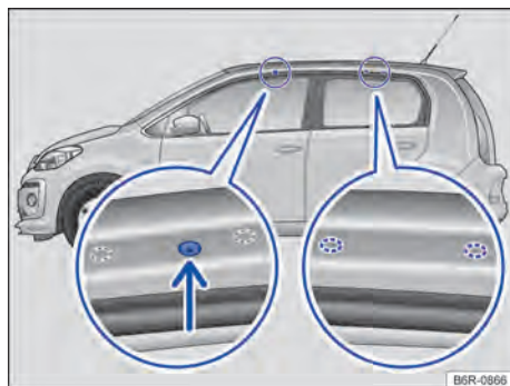
Fig. 106 Veículos sem bagageiro do teto: Pontos de fixação dos suportes de base do bagageiro do teto (ambos os lados).
