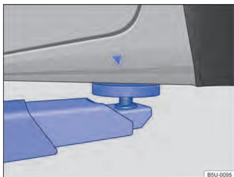
Fig. 154 Pontos de apoio traseiros para a suspensão com plataforma elevatória ou com macaco.
