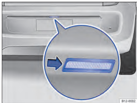
Fig. 119 No para-choque traseiro: remover a lanterna da placa de licença.
