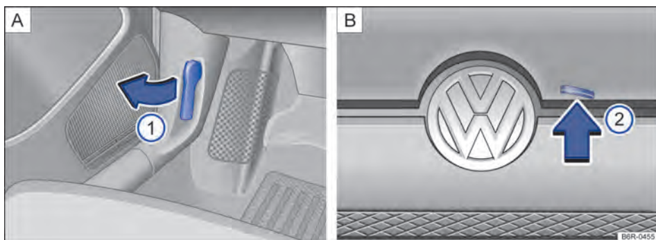
Fig. 130 A: alavanca de destravamento na área para os pés do lado do condutor. B: alavanca de destravamento na parte interna da tampa do compartimento do motor.
