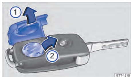
Fig. 45 Chave do veículo com comando remoto: substituir a bateria.
