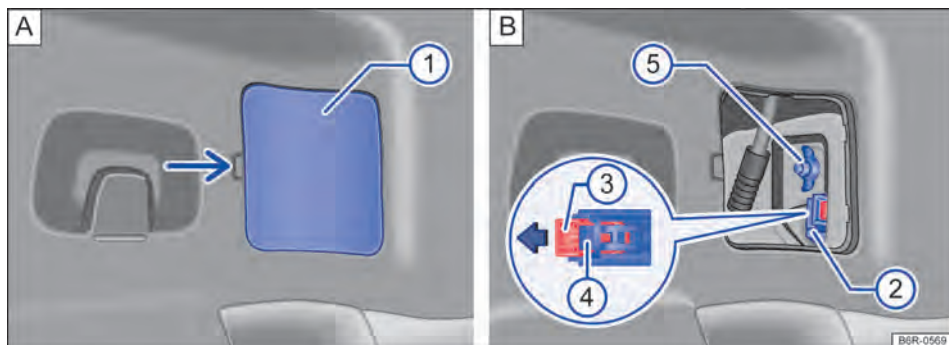
Fig. 117 Lateralmente no compartimento de bagagem: A: desinstalar a cobertura, B: remover a lanterna traseira.
