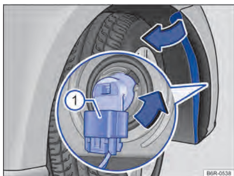
Fig. 116 Substituir a lâmpada incandescente do farol.
