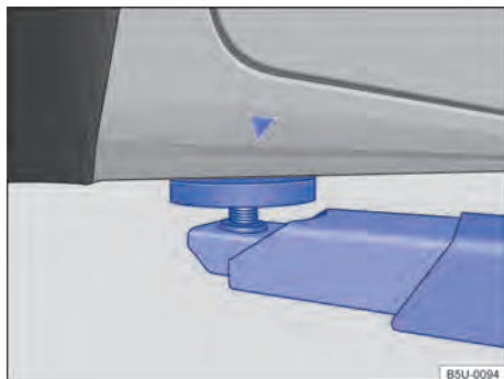
Fig. 153 Pontos de apoio dianteiros para a suspensão com plataforma elevatória ou com macaco.
