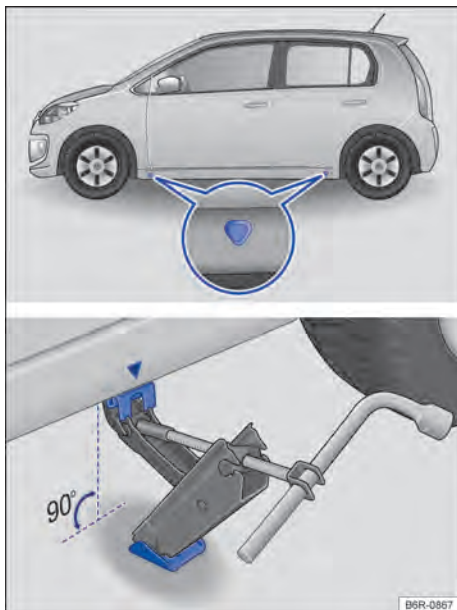
Fig. 150 Pontos de apoio do macaco e macaco posicionado no lado esquerdo traseiro do veículo.
