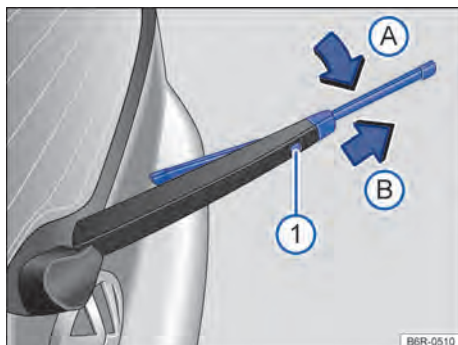
Fig. 113 Substituir a palheta do limpador do vidro traseiro.
