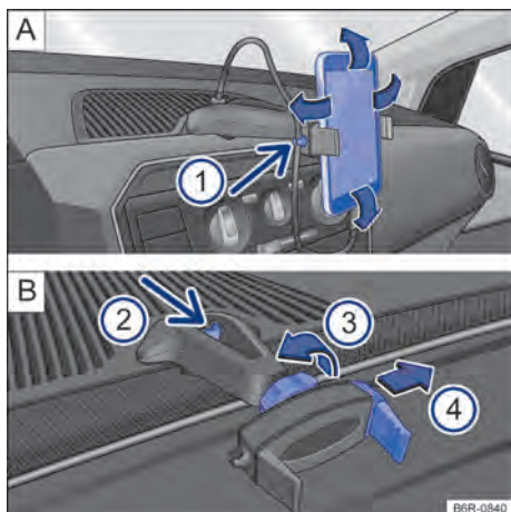
Fig. 151 No console central: suporte para telefone celular e ajustes.
