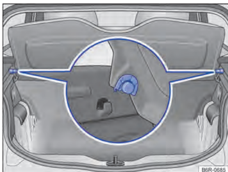
Fig. 102 No compartimento de bagagem: remover e instalar a cobertura do compartimento de bagagem. ➤
