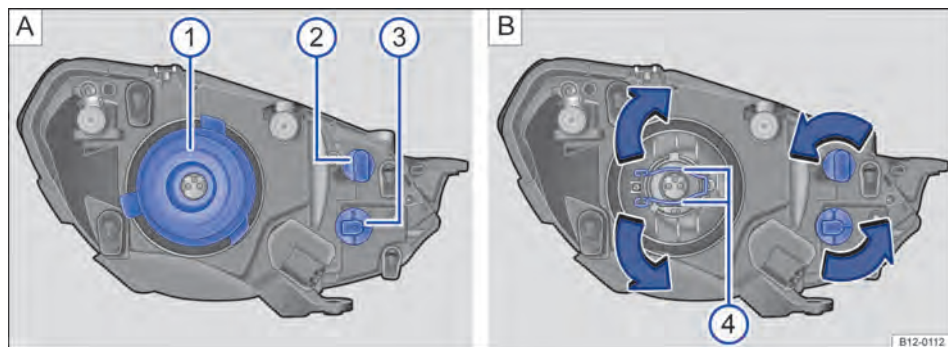
Fig. 114 No compartimento do motor: vista traseira do farol dianteiro esquerdo com cobertura de borracha: ❶ farol baixo e farol alto, ❷ luz de posição e/ou luz de condução diurna, ❸ indicadores de direção e trava de proteção ❹.
