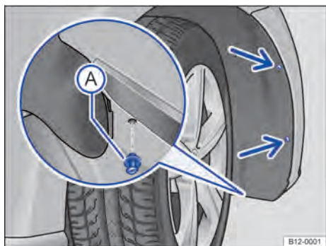
Fig. 115 Na caixa da roda dianteira direita: remover os parafusos de fixação (setas) e remover o rebite de expansão (A).
