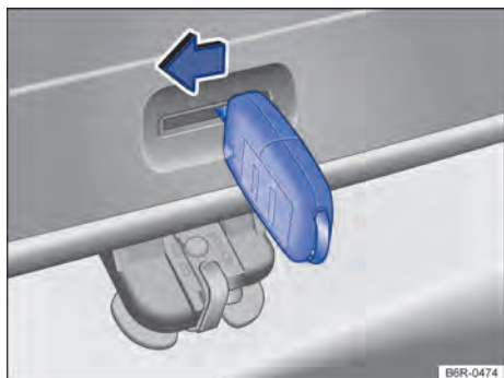
Fig. 55 Do lado de dentro do compartimento de bagagem: destravamento de emergência da tampa traseira.
