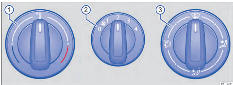
Fig. 73 No console central: comandos do sistema de ventilação e aquecimento. ▶
