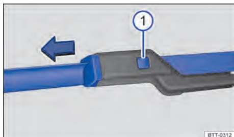
Fig. 112 Substituir as palhetas dos limpadores do para-brisa.
