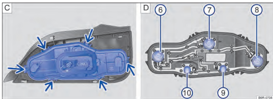
Fig. 118 Lanterna traseira: C: desinstalar o suporte da lâmpada, D: desinstalar a lâmpada incandescente.
