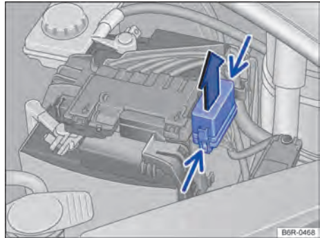
Fig. 122 No compartimento do motor: retirar cobertura da caixa de fusíveis.
