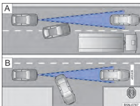
Fig. 161 A Mudança de faixa de um veículo. B Veículo virando ou parando.
