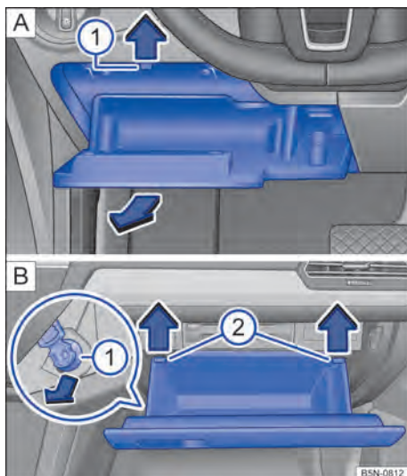
Fig. 239 Cobertura da caixa de fusíveis no painel de instrumentos: A veículos com direção à esquerda, à esquerda ao lado do volante. B veículos com direção à direita, no lado passageiro dianteiro.
