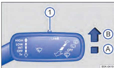
Fig. 113 Na alavanca dos limpadores do para-brisa à direita da coluna de direção: ajustar o sensor de chuva e de luz ①.
