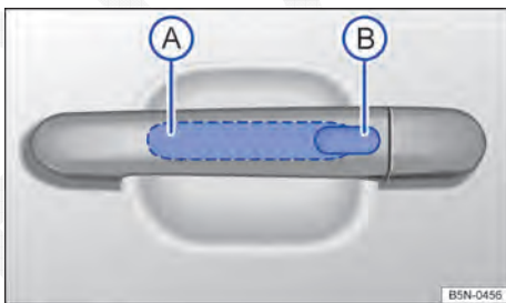
Fig. 30 Sistema de travamento e de partida Keyless Access sem chave: superfície do sensor (A) para destravar na parte interna da maçaneta da porta e superfície do sensor (B) para travamento na parte externa da maçaneta da porta.
