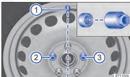
Fig. 233 Troca de roda: Válvula do pneu ① e locais de instalação do parafuso de roda antifurto ② ou ③.
