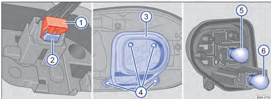
Fig. 249 Lanterna traseira desinstalada: desinstalar o suporte de lâmpadas e trocar as lâmpadas da lanterna traseira e da lanterna de freio ⑤ ou a lâmpada do indicador de direção ⑥.
