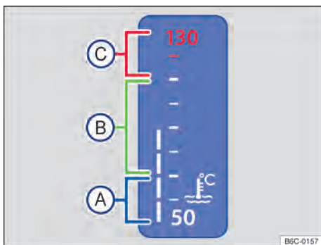
Fig. 16 Indicador de temperatura do líquido de arrefecimento do motor no instrumento combinado digital (variante 1): (A) área fria; (B) área normal; (C) área de alerta.
