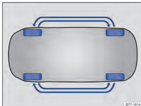
Fig. 213 Esquema para a troca das rodas.
