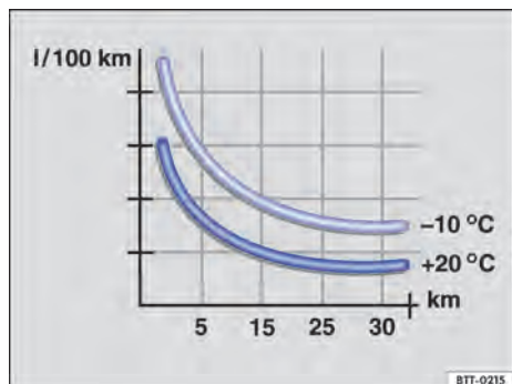
Fig. 91 Consumo de combustível em l/100 km em 2 temperaturas ambiente diferentes.
