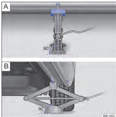
Fig. 222 Pontos de apoio do macaco e macaco posicionado no lado esquerdo traseiro do veículo.
