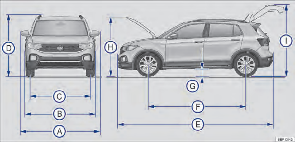
Fig. 228 Dimensões.
