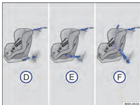
Fig. 43 No banco traseiro: as figuras D e E mostram o princípio da fixação do sistema de retenção para crianças nos olhais de retenção inferiores e com o cinto de fixação superior. A figura F mostra a fixação do sistema de retenção para crianças com o cinto de segurança do veículo e com o cinto de fixação superior.
