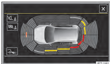
Fig. 102 Indicação no sistema do rádio: modo de tela cheia. As áreas registradas dependem da versão do veículo.
