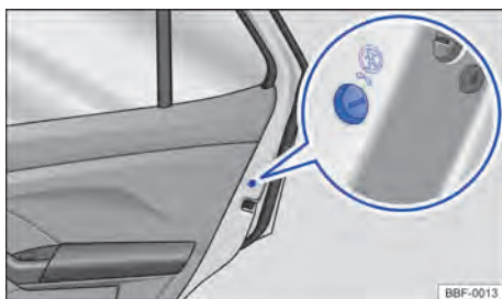
Fig. 45 Na porta traseira (lado direito): localização da trava de segurança para crianças.
