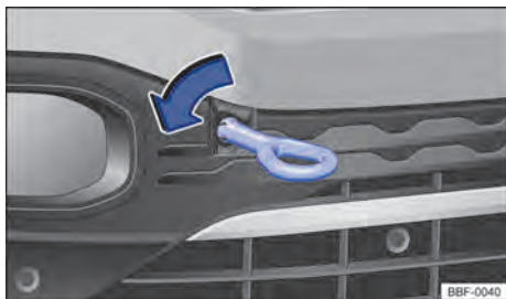
Fig. 153 No para-choque dianteiro à direita: rosquear a argola de reboque.
