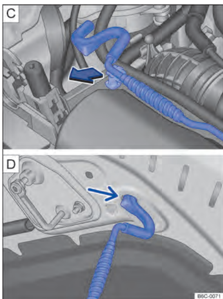
Fig. 155 [C] Haste de sustentação da tampa do compartimento do motor. [D] Tampa do compartimento do motor apoiada na haste de sustentação.
