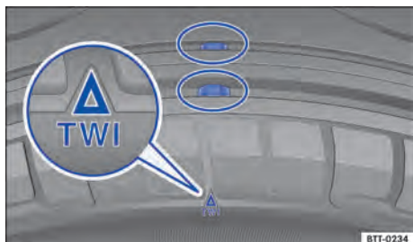
Fig. 168 Perfil do pneu: indicadores de desgaste.
