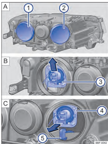
Fig. 139 No compartimento do motor: ① farol baixo e ② farol alto e luz de posição.
