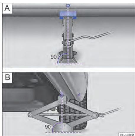
Fig. 175 Pontos de apoio do macaco e macaco posicionado no lado esquerdo traseiro do veículo.
