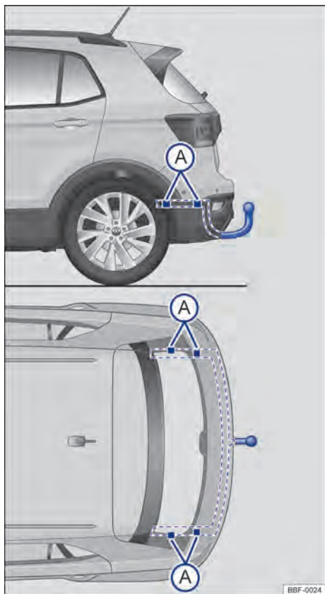
Fig. 131 Pontos de fixação para instalar um dispositivo de reboque posteriormente.
