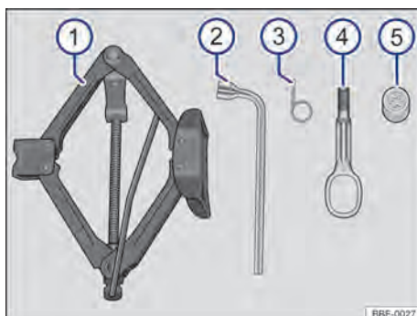
Fig. 135 Componentes das ferramentas de bordo.
