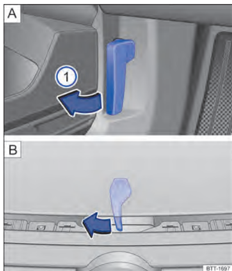
Fig. 154 [A] Alavanca de destravamento da tampa do compartimento do motor na área para os pés do lado do condutor. [B] Alavanca de destravamento na parte interna da tampa do compartimento do motor.
