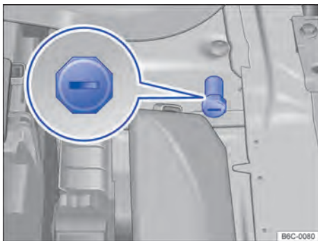
Fig. 150 No compartimento do motor: ponto de auxílio à partida (ponto de aterramento).
