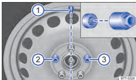
Fig. 173 Troca de roda: válvula do pneu ① e posição de montagem do parafuso da roda antifurto ② ou ③.
