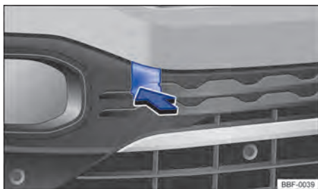
Fig. 152 No para-choque dianteiro à direita: soltar e remover a cobertura.
