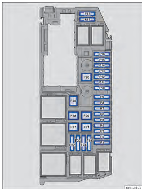
Fig. 146 No compartimento do motor: disposição dos fusíveis.
