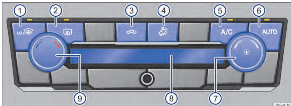
Fig. 86 Comandos do Climatronic.
