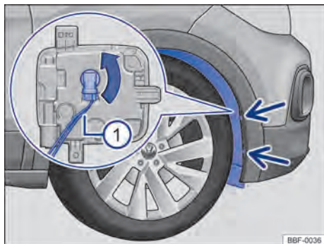
Fig. 140 Na caixa de roda dianteira: acesso à lâmpada incandescente do farol de neblina.
