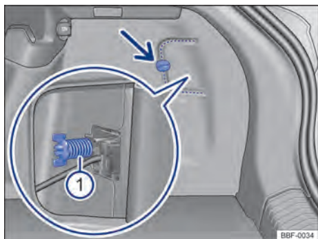
Fig. 141 No compartimento de bagagem: desinstalar cobertura e retirar o parafuso borboleta ❶ (lupa).
