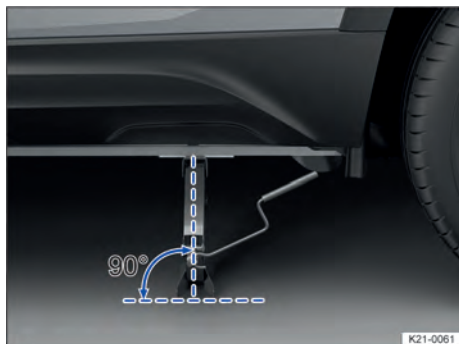
Fig. 183 Alinhamento correto do macaco.
