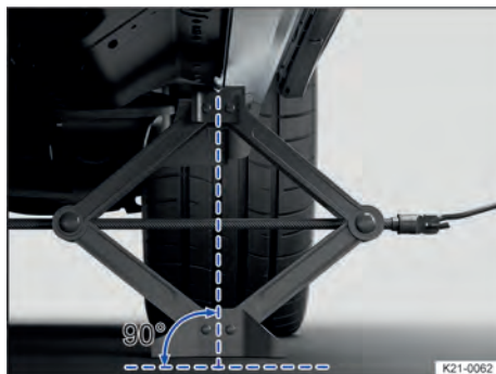
Fig. 184 Atrás, do lado esquerdo do veículo: macaco posicionado.
