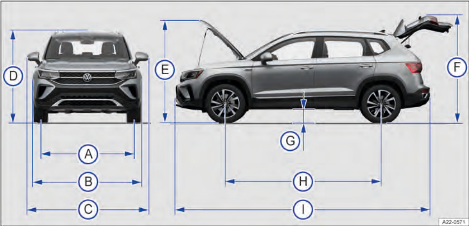
Fig. 265 Dimensões do veículo.
