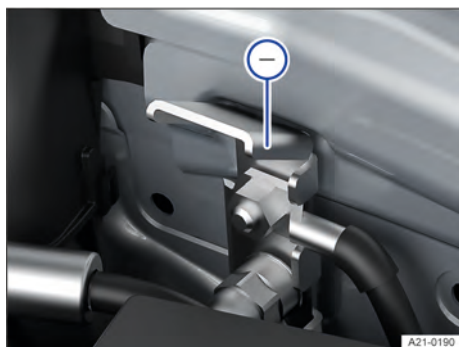
Fig. 152 No compartimento dianteiro: ponto de auxílio à partida de massa.
