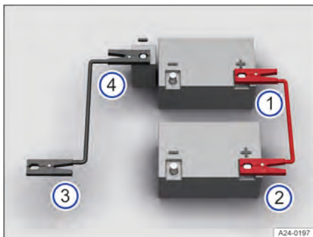
Fig. 153 Esquema para conexão dos cabos auxiliares de partida.
