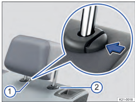
Fig. 62 Desinstalar o apoio para cabeça traseiro (representação esquemática).
