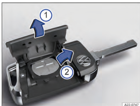
Fig. 39 Chave do veículo: trocar a pilha-botão (representação esquemática).
