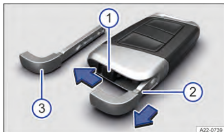
Fig. 38 Chave do veículo: destravamento da chave de emergência (representação esquemática).
