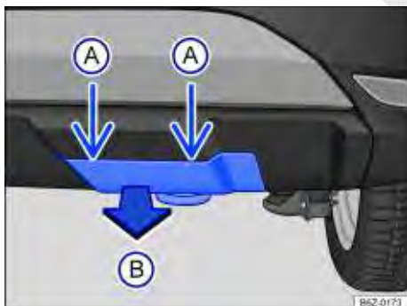
Fig. 192 No para-choque traseiro à direita: argola de reboque traseira - para-choque com cobertura removível.
