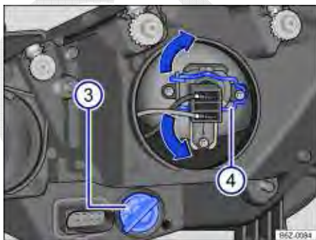
Fig. 175 No compartimento do motor: vista traseira do farol dianteiro direito sem cobertura de borracha: (3) indicadores de direção e (4) farol baixo.
