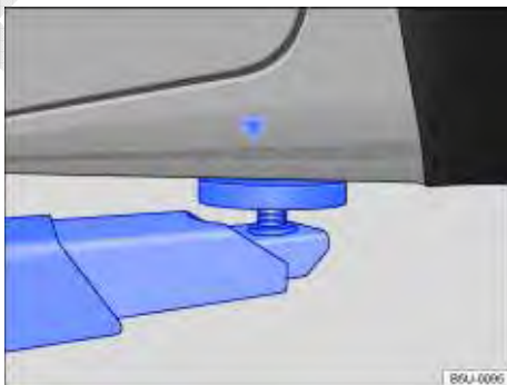
Fig. 146 Pontos de apoio traseiros para a suspensão com plataforma elevatória ou com macaco.
