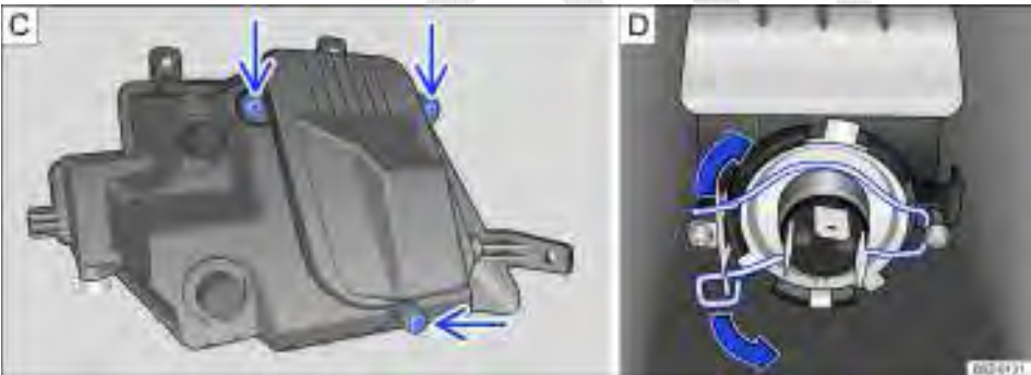
Fig. 178 No para-choque dianteiro: (C) retirar os parafusos da cobertura da lâmpada e (D) lâmpada do farol de neblina.
