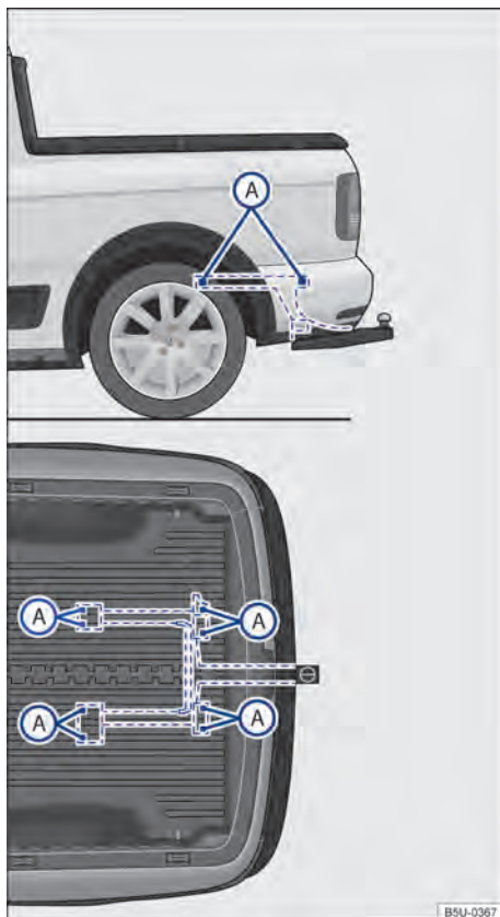
Fig. 167 Pontos de fixação para instalar um dispositivo de reboque posteriormente.
