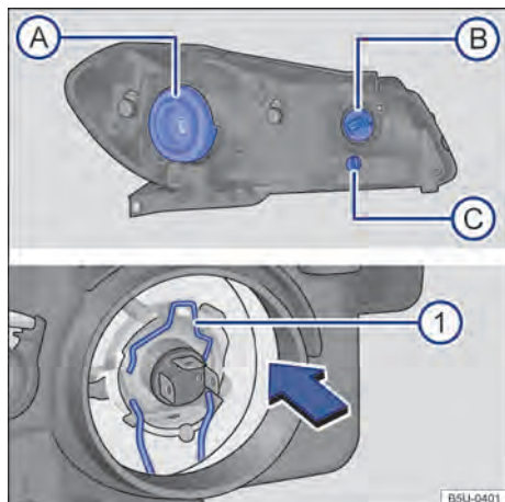
Fig. 178 No compartimento do motor: vista traseira do farol dianteiro com cobertura de borracha (lado esquerdo da ilustração) - A farol baixo / alto, B indicadores de direção e C luz de posição. Vista traseira do farol dianteiro sem a cobertura de borracha (lado direito da ilustração): 1 mola de travamento da lâmpada incandescente do farol baixo / alto.
