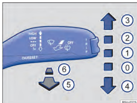
Fig. 70 Comandar os limpadores / lavadores do para-brisa.
