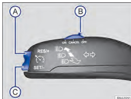
Fig. 91 À esquerda na coluna da direção: alavanca com interruptor e botões de comando do GRA.
