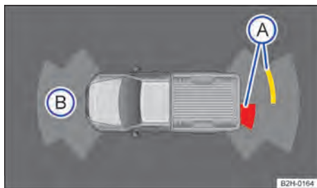
Fig. 95 Exibição do display do controle de distância de estacionamento (display colorido): (A) obstáculo reconhecido no segmento. (B) área examinada à frente do veículo.
