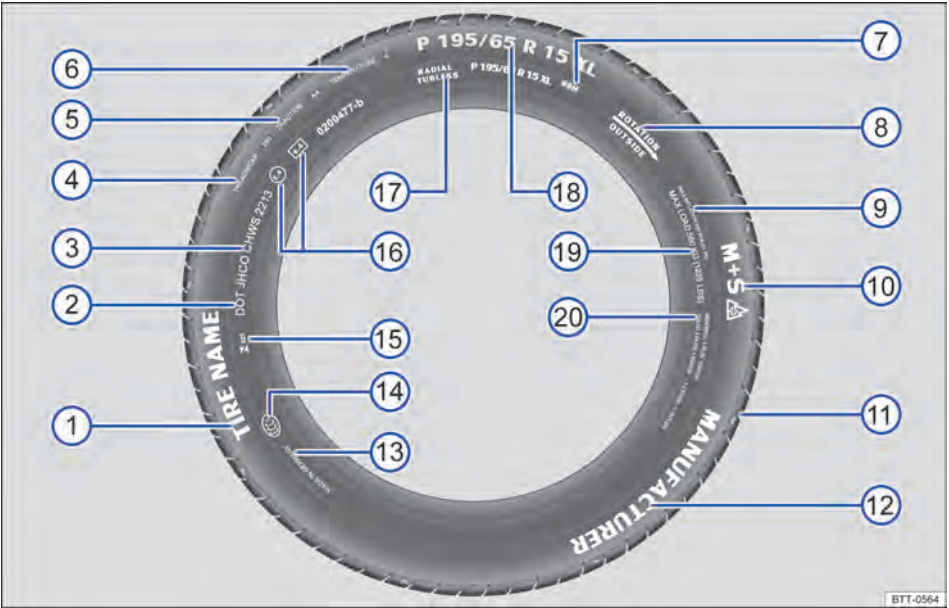
Fig. 215 Inscrição dos pneus internacional (exemplo).
