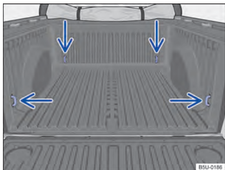
Fig. 161 Compartimento de carga: olhais de amarração.
