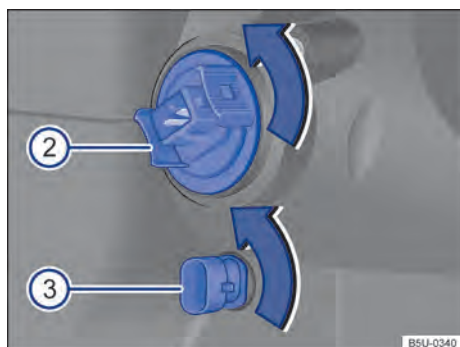
Fig. 179 No compartimento do motor: vista traseira do farol dianteiro 2 indicadores de direção e 3 luz de posição.
