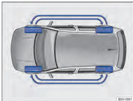
Fig. 210 Esquema para a troca das rodas.
