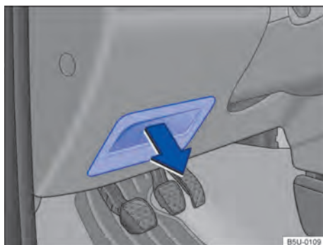
Fig. 191 No lado do condutor no painel de instrumentos: cobertura da caixa de fusíveis.
