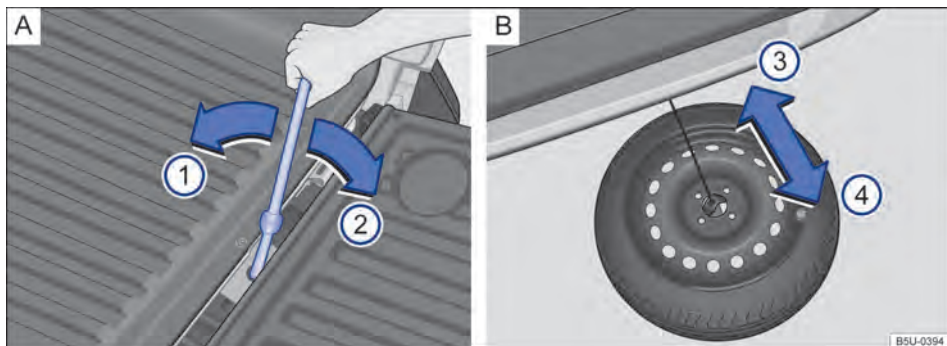
Fig. 213 [A] No compartimento de carga: acesso a roda de emergência. [B] Sob o veículo: roda de emergência totalmente no piso e retirada de baixo do veículo.
