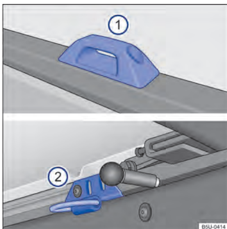
Fig. 162 No compartimento de carga: suportes fixos ① para veículos sem capota marítima e ② para veículos com capota marítima.
