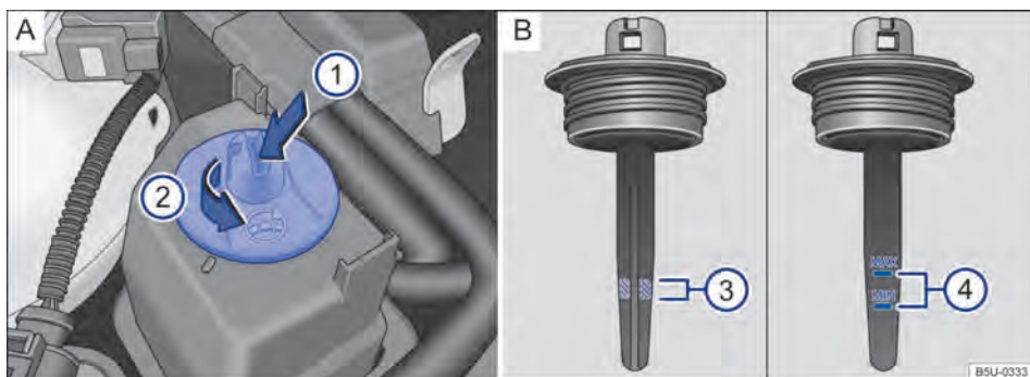
Fig. 88 No compartimento do motor (variante 1): A Reservatório do fluido da direção hidráulica. B Marcações para controle do nível do fluido da direção hidráulica.
