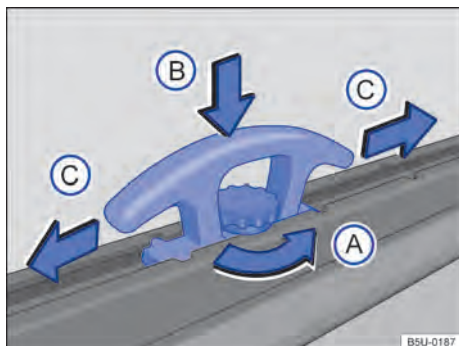
Fig. 163 No compartimento de carga: suporte deslizante para veículos sem capota marítima.
