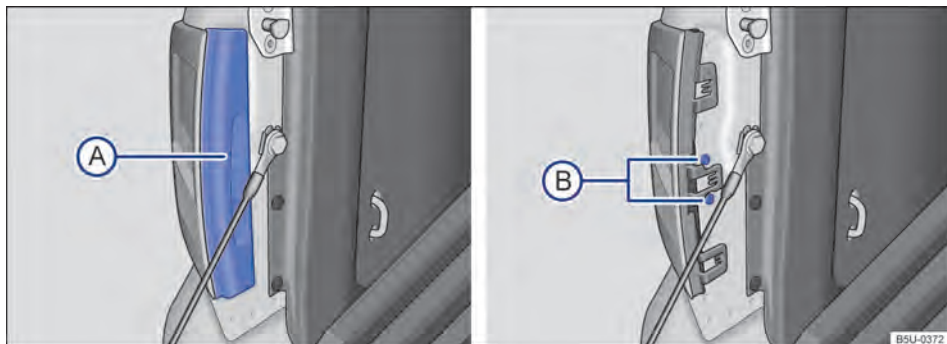
Fig. 185 No compartimento de carga: A desinstalar cobertura, B retirar os parafusos de fixação. ►
