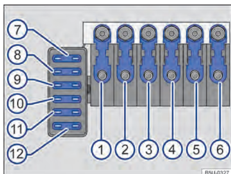
Fig. 194 Caixa de fusíveis.
