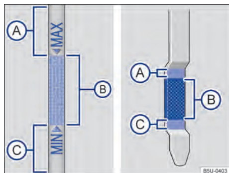
Fig. 202 Vareta de medição do óleo com marcas de nível do óleo do motor.
