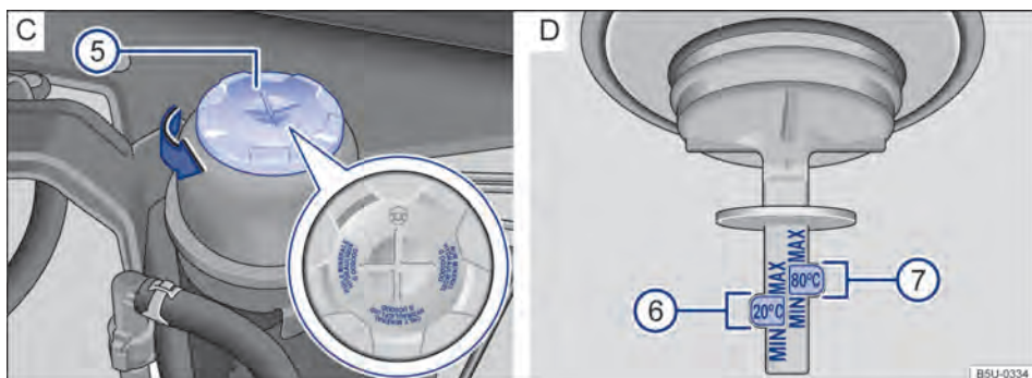
Fig. 89 No compartimento do motor (variante 2): C Reservatório do fluido da direção hidráulica. D Marcações para controle do nível do fluido da direção hidráulica.
