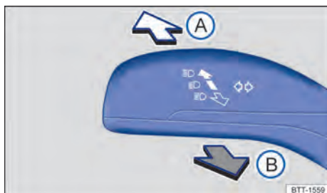
Fig. 67 À esquerda na coluna de direção: alavanca dos indicadores de direção e do farol alto.
