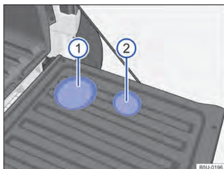
Fig. 109 No revestimento da tampa do compartimento de carga: ① porta-garrafas e ② porta-copos. ▶
