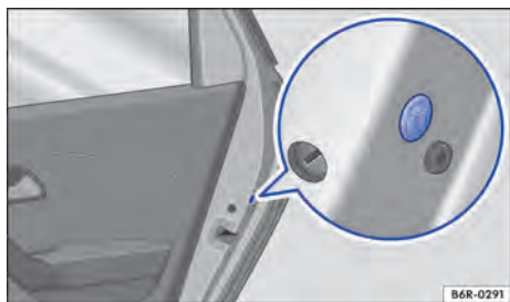
Fig. 45 Na parte dianteira da porta direita: travamento de emergência, coberto por uma vedação de borracha.
