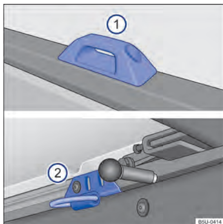
Fig. 164 No compartimento de carga: suportes fixos ① para veículos sem capota marítima e ② para veículos com capota marítima.
