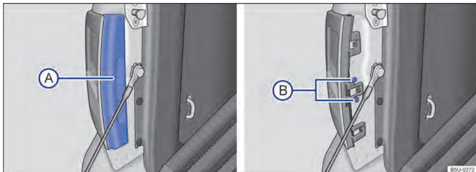
Fig. 187 No compartimento de carga: (A) desinstalar cobertura, (B) retirar os parafusos de fixação. ►
