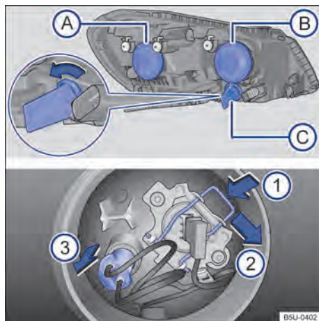
Fig. 182 No compartimento do motor: vista traseira do farol dianteiro com cobertura de borracha (lado esquerdo da ilustração) - (A) farol baixo, (B) farol alto e luz de posição, e (C) indicador de direção. Vista traseira do farol dianteiro sem a cobertura de borracha (lado direito da ilustração): ① mola de travamento da lâmpada incandescente do farol e ② luz de posição.
