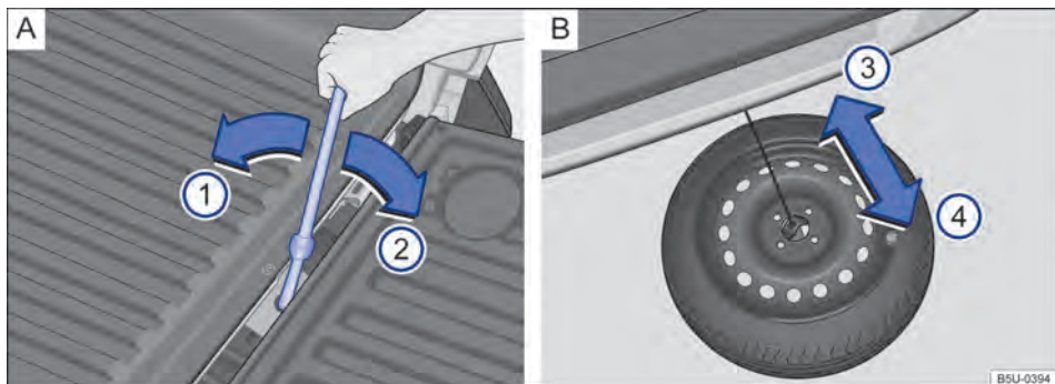
Fig. 215 [A] No compartimento de carga: acesso a roda de emergência. [B] Sob o veículo: roda de emergência totalmente no piso e retirada de baixo do veículo.
