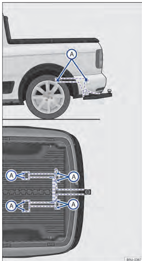
Fig. 169 Pontos de fixação para instalar um dispositivo de reboque posteriormente.
