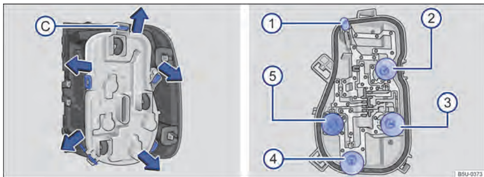
Fig. 188 Lanterna traseira: (C) desinstalar o suporte das lâmpadas e (1), (2), (3), (4) e (5) desinstalar as lâmpadas.
