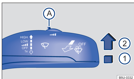
Fig. 84 Alavanca dos limpadores do para-brisa: regular a sensibilidade do sensor de chuva (A).
