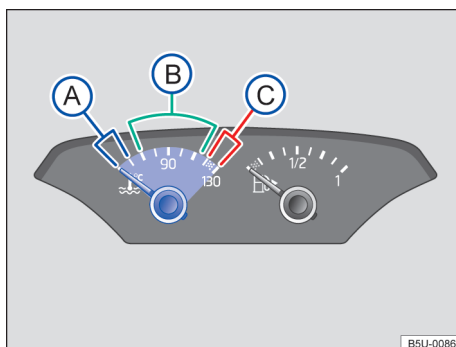
Fig. 22 Indicador de temperatura do líquido de arrefecimento do motor no instrumento combinado: (A) área fria; (B) área normal; (C) área de alerta.
