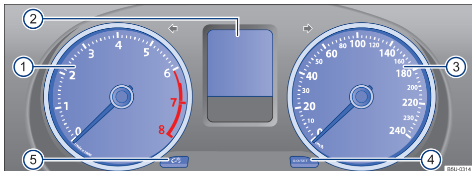
Fig. 13 Instrumento combinado no painel de instrumentos (variante 1).
