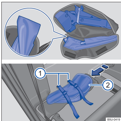
Fig. 151 Atrás do encosto do banco do passageiro: ① cintas de fixação da bolsa das ferramentas de bordo e ② bolsa das ferramentas de bordo.
