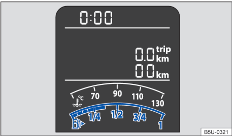
Fig. 17 No display do instrumento combinado: indicador do nível de combustível (variante 1).
