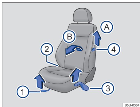
Fig. 73 No banco dianteiro: comandos.
