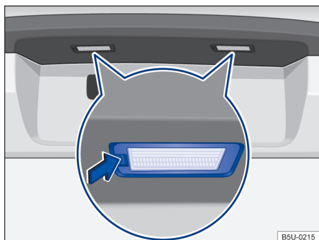
Fig. 166 No para-choque traseiro: remover a lanterna da placa de licença.
