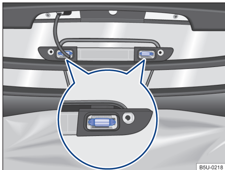
Fig. 169 Lanterna de freio elevada: remover a lâmpada incandescente da iluminação do compartimento de carga.
