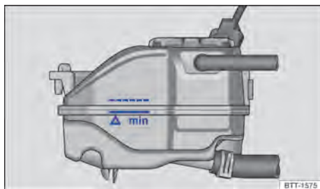
Fig. 190 No compartimento do motor: marcação no reservatório de expansão do líquido de arrefecimento do motor.
