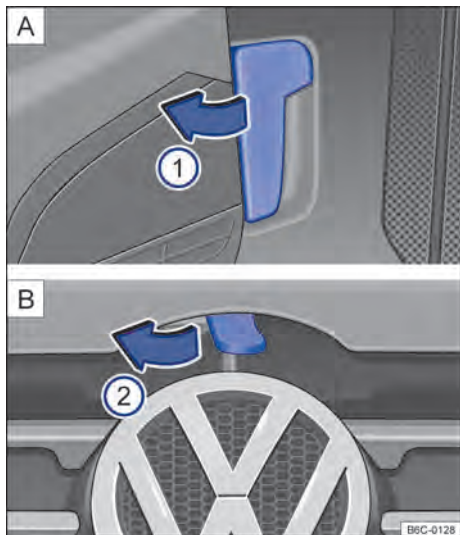
Fig. 184 A) Alavanca de destravamento da tampa do compartimento do motor na área para os pés do lado do condutor. B) Alavanca de destravamento na parte interna da tampa do compartimento do motor.
