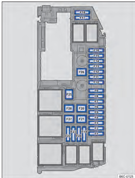
Fig. 178 No compartimento do motor: disposição dos fusíveis.
