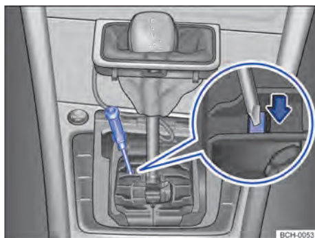
Fig. 97 Desinstalar a cobertura da alavanca seletora e destravar o bloqueio da alavanca seletora emergencialmente.
