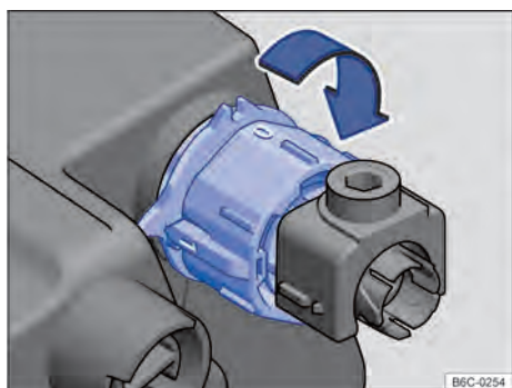
Fig. 75 No compartimento do motor: interruptor de regulagem de alcance do farol.
