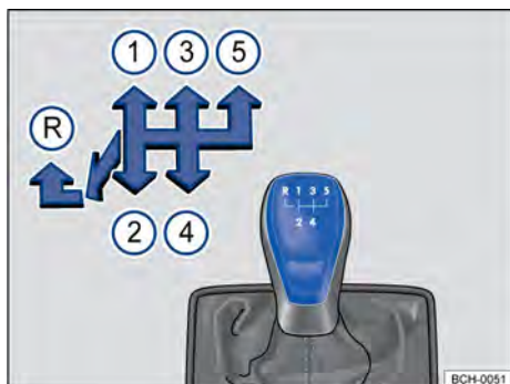
Fig. 93 Esquema de troca de marchas da transmissão manual de 5 marchas.
