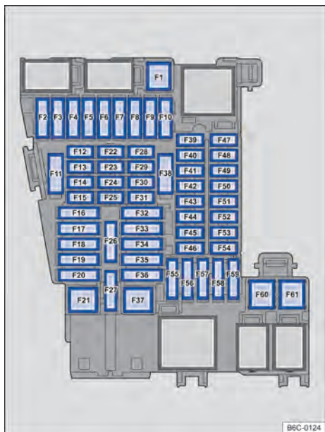
Fig. 176 No painel de instrumentos: disposição dos fusíveis.
