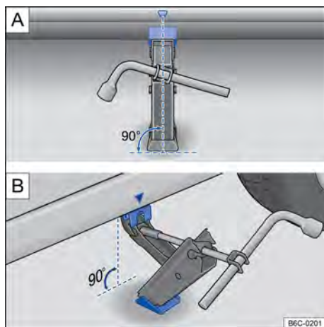
Fig. 205 Pontos de apoio do macaco e macaco posicionado no lado esquerdo traseiro do veículo.
