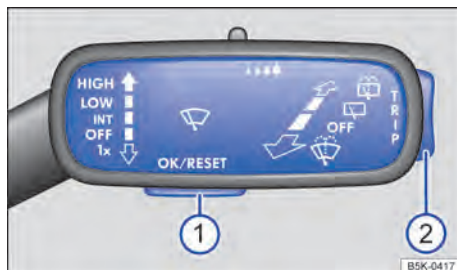
Fig. 19 Veículos sem volante multifunções: botão ① na alavanca dos limpadores dos vidros para confirmação dos itens de menu e chave ② para alternar entre os menus.
