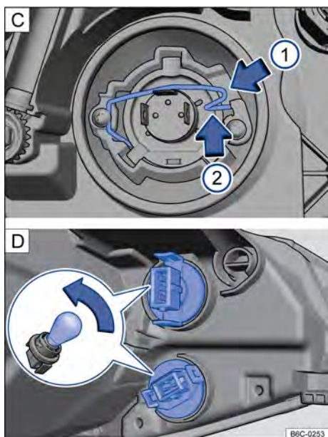
Fig. 170 No compartimento do motor: cobertura do indicador de direção do farol alto e baixo.
