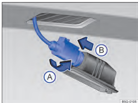
Fig. 174 Lanterna da placa de licença: desinstalar o suporte da lâmpada.
