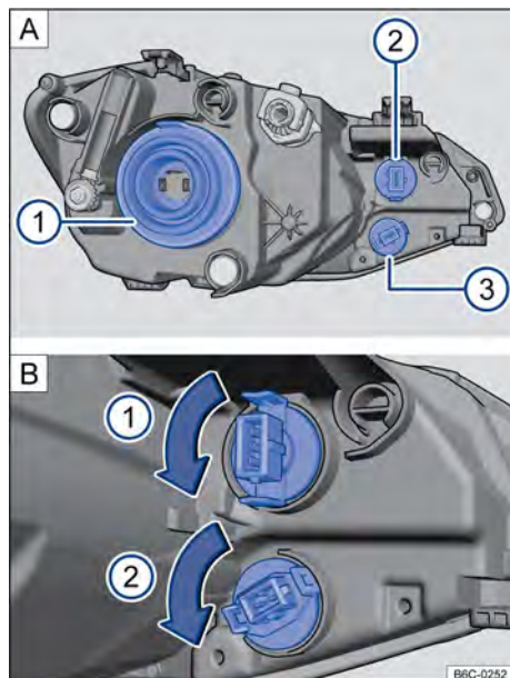
Fig. 169 No compartimento do motor: farol dianteiro. ① Luz de rodagem diurna e luz de posição e ② Indicadora de direção.
