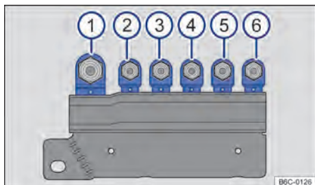
Fig. 179 No compartimento do motor em cima da bateria: disposição dos fusíveis.
