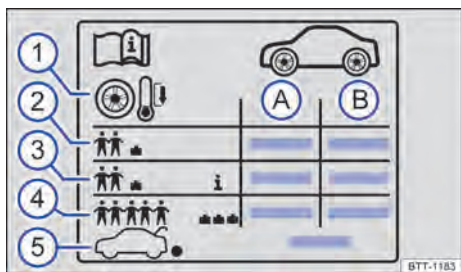
Fig. 196 Etiqueta com as pressões dos pneus.
