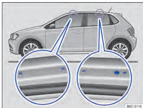
Fig. 159 Pontos de fixação dos suportes de base do bagageiro do teto (ambos os lados).
