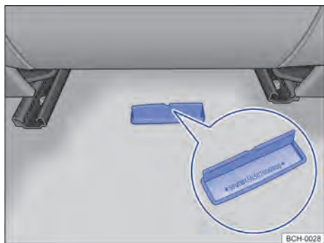
Fig. 209 Em frente ao banco do passageiro traseiro no assoalho direito: número de identificação do veículo (número do chassi).
