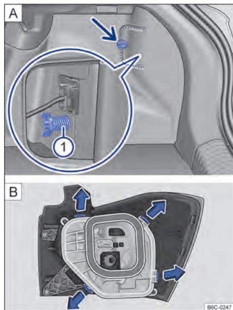
Fig. 171 (A) No compartimento de bagagem: desinstalar cobertura e retirar o parafuso borboleta (1) (lupa). (B) Lanterna traseira: desinstalar o suporte das lâmpadas.
