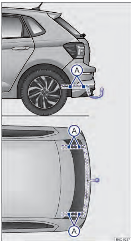
Fig. 160 Pontos de fixação para instalar um dispositivo de reboque posteriormente.
