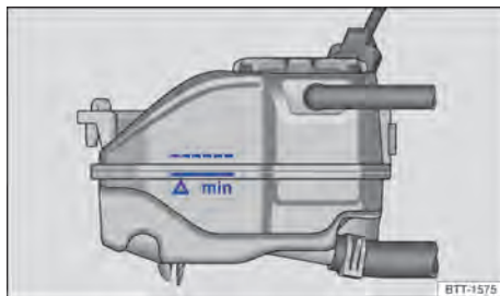
Fig. 187 No compartimento do motor: marcação no reservatório de expansão do líquido de arrefecimento do motor.
