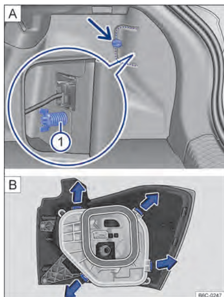
Fig. 168 (A) No compartimento de bagagem: desinstalar cobertura e retirar o parafuso borboleta ⓘ (lupa). (B) Lanterna traseira: desinstalar o suporte das lâmpadas.
