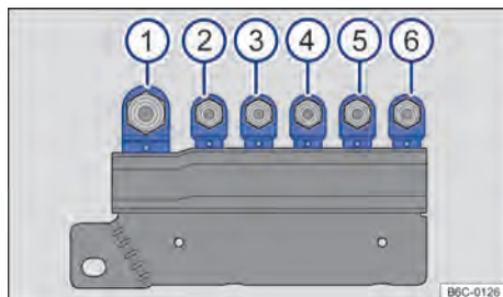
Fig. 176 No compartimento do motor em cima da bateria: disposição dos fusíveis.
