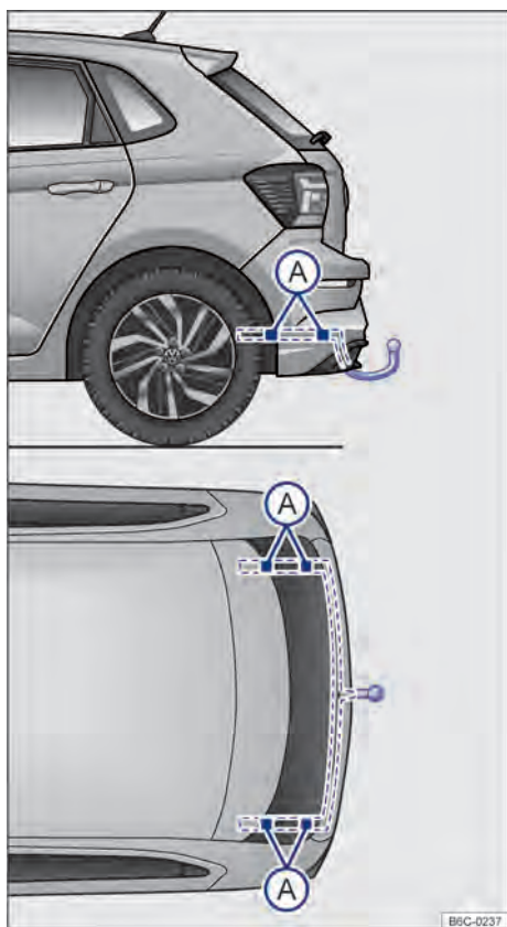
Fig. 158 Pontos de fixação para instalar um dispositivo de reboque posteriormente.
