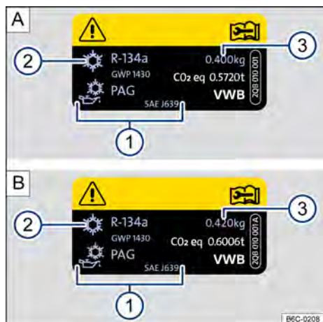
Fig. 209 [A]: informações do ar-condicionado - motor 1.0L. [B]: informações do ar-condicionado - motor 1.0L TSI, motor 1.4L TSI e motor 1.6L.
