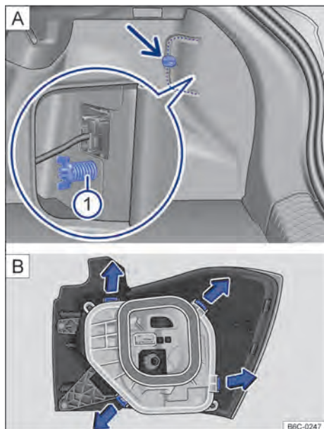
Fig. 169 (A) No compartimento de bagagem: desinstalar cobertura e retirar o parafuso borboleta (lupa). (B) Lanterna traseira: desinstalar o suporte das lâmpadas.
