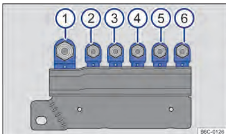
Fig. 177 No compartimento do motor em cima da bateria: disposição dos fusíveis.
