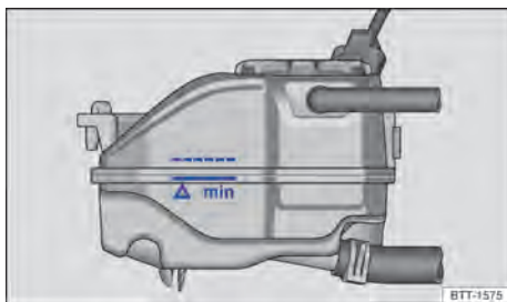
Fig. 188 No compartimento do motor: marcação no reservatório de expansão do líquido de arrefecimento do motor.
