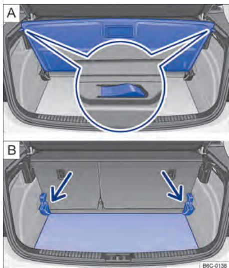
Fig. 154 No compartimento de bagagem: ajustar a altura do assoalho do compartimento de bagagem.
