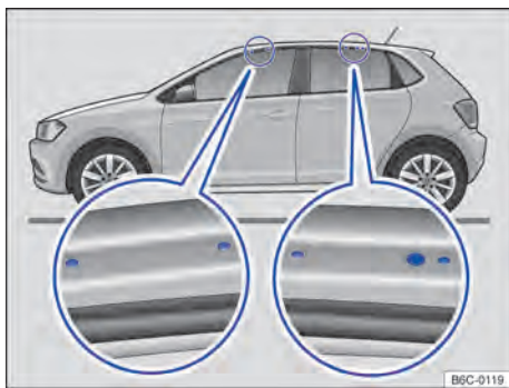
Fig. 157 Pontos de fixação dos suportes de base do bagageiro do teto (ambos os lados).
