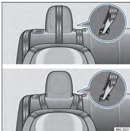
Fig. 46 No encosto do banco traseiro: A ) posição do cadarço do cinto de segurança no caso de apoios para cabeça não ajustáveis com cinto individual Top Tether, B ) posição do cadarço do cinto de segurança no caso de apoios para cabeça não ajustáveis com cinto Top Tether em forma de V.
