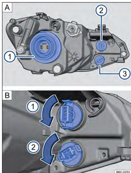
Fig. 167 No compartimento do motor: farol dianteiro. ① Luz de rodagem diurna e luz de posição e ② Indicadora de direção.
