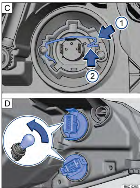
Fig. 168 No compartimento do motor: cobertura do indicador de direção do farol alto e baixo.
