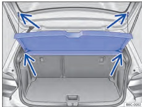
Fig. 152 No compartimento de bagagem: remover e instalar a cobertura do compartimento de bagagem.
