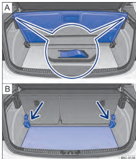
Fig. 152 No compartimento de bagagem: ajustar a altura do assoalho do compartimento de bagagem.
