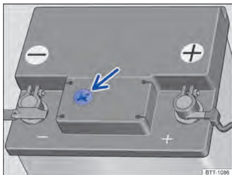
Fig. 191 No compartimento do motor: exemplo de posição do visor no lado superior da bateria do veículo.
