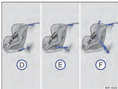
Fig. 41 No banco traseiro: as figuras D e E mostram o princípio da fixação do sistema de retenção para crianças nos olhalos de retenção inferiores e com o cinto de fixação superior. A figura F mostra a fixação do sistema de retenção para crianças com o cinto de segurança do veículo e com o cinto de fixação superior.
