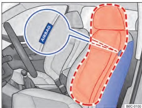
Fig. 39 Lateralmente no banco dianteiro: localização de instalação e área de expansão dos airbags laterais.
