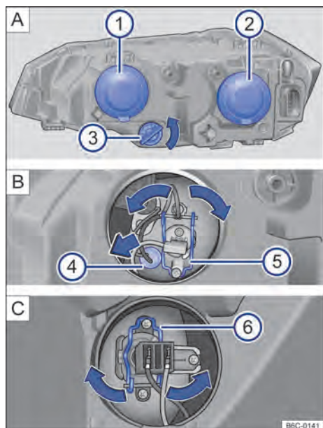
Fig. 167 No compartimento do motor: 1) farol alto e luz de posição, 2) farol baixo e 3) indicador de direção.
