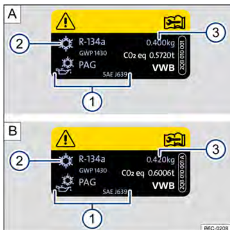
Fig. 207 [A]: informações do ar-condicionado - motor 1.0L. [B]: informações do ar-condicionado - motor 1.0L TSI, motor 1.4L TSI e motor 1.6L.
