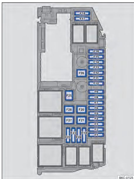
Fig. 174 No compartimento do motor: disposição dos fusíveis.
