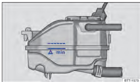
Fig. 186 No compartimento do motor: marcação no reservatório de expansão do líquido de arrefecimento do motor.
