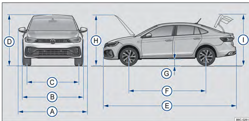
Fig. 207 Dimensões.
