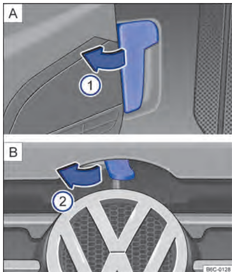
Fig. 180 [A] Alavanca de destravamento da tampa do compartimento do motor na área para os pés do lado do condutor. [B] Alavanca de destravamento na parte interna da tampa do compartimento do motor. ►
