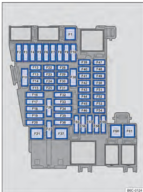
Fig. 172 No painel de instrumentos: disposição dos fusíveis.
