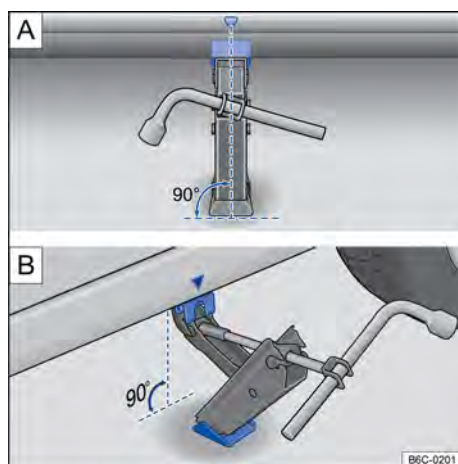
Fig. 200 Pontos de apoio do macaco e macaco posicionado no lado esquerdo traseiro do veículo.
