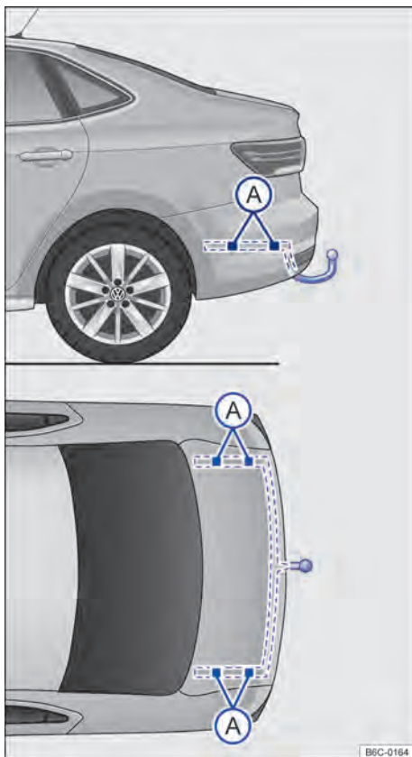
Fig. 162 Pontos de fixação para instalar um dispositivo de reboque posteriormente.
