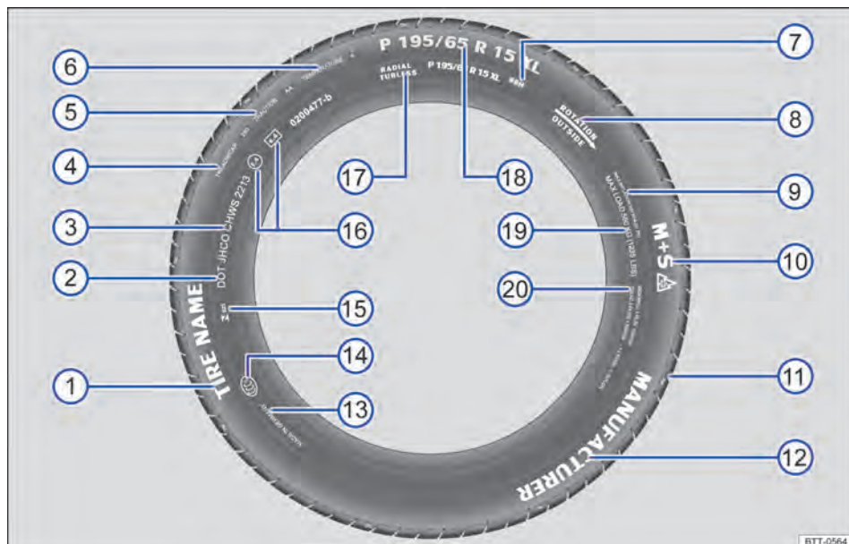
Fig. 195 Inscrição dos pneus internacional (exemplo).
