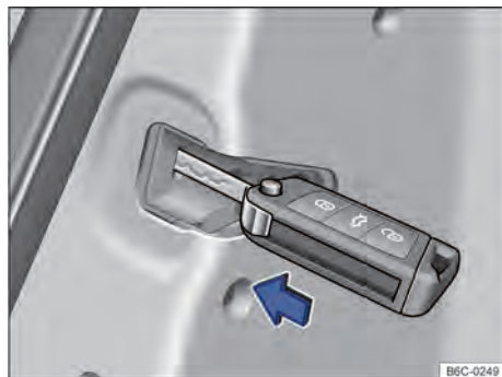
Fig. 59 Nas portas, dianteira direita e traseiras: travamento de emergência do veículo com a haste metálica da chave.
