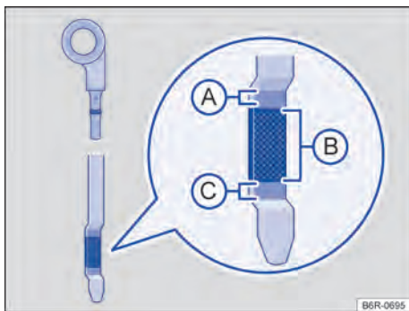
Fig. 184 Vareta de medição do óleo com marcas de nível do óleo do motor.
