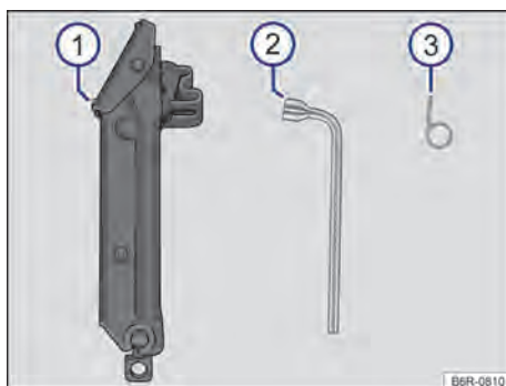
Fig. 166 Componentes das ferramentas de bordo.
