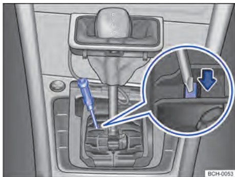
Fig. 95 Desinstalar a cobertura da alavanca seletora e destravar o bloqueio da alavanca seletora emergencialmente.
