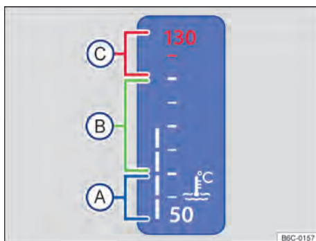
Fig. 13 Indicador de temperatura do líquido de arrefecimento do motor no instrumento combinado digital (variante 1): (A) área fria; (B) área normal; (C) área de advertência.
