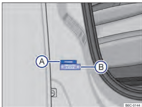
Fig. 205 Na área inferior da coluna da porta dianteira direita: etiqueta com número de identificação do veículo parcial (VIS) (A) e placa do ano de fabricação (B).
