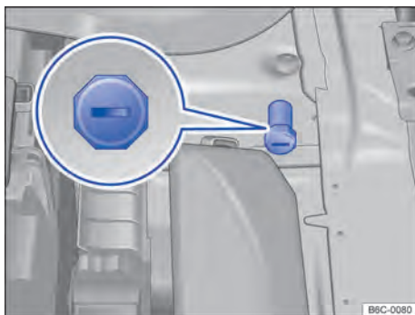
Fig. 178 No compartimento do motor: ponto de auxílio à partida (ponto de aterramento).
