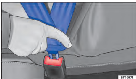
Fig. 29 Introduzir a lingueta do cinto de segurança no fecho do cinto de segurança.
