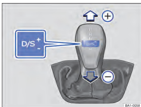
Fig. 93 Alavanca seletora na posição Tiptronic.
