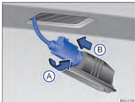
Fig. 170 Lanterna da placa de licença: desinstalar o suporte da lâmpada.
