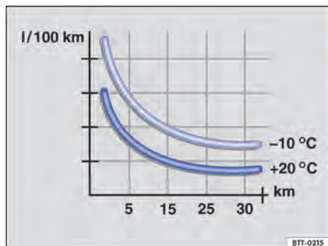
Fig. 87 Consumo de combustível em l/100 km em 2 temperaturas ambiente diferentes.
