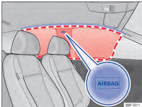
Fig. 40 No lado esquerdo do veículo: local de instalação e área de expansão do airbag para cabeça.
