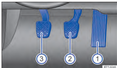
Fig. 84 Na área para os pés: pedais em veículos com transmissão manual.
