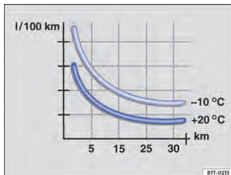
Fig. 92 Consumo de combustível em l/100 km em 2 temperaturas ambiente diferentes.
