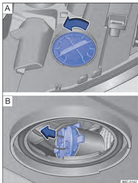
Fig. 135 Farol dianteiro, por baixo: cobertura do indicador de direção.
