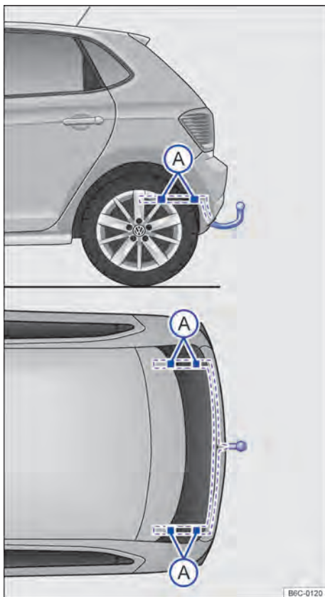
Fig. 125 Pontos de fixação para instalar um dispositivo de reboque posteriormente.
