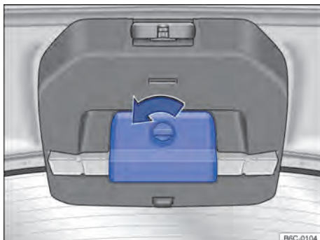
Fig. 53 Na tampa do compartimento de bagagem: suporte para o triângulo de segurança.
