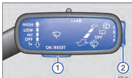
Fig. 22 Veículos sem volante multifunções: botão ① na alavanca dos limpadores dos vidros para confirmação dos itens de menu e chave ② para alternar entre os menus.
