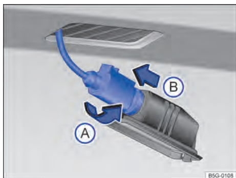
Fig. 141 Lanterna da placa de licença: desinstalar o suporte da lâmpada.
