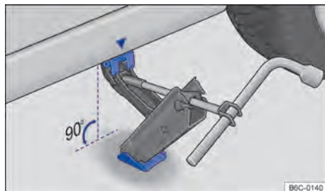
Fig. 171 Pontos de apoio do macaco e macaco posicionado no lado esquerdo traseiro do veículo.
