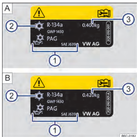
Fig. 177 [A]: informações do ar-condicionado - motor 1.0L. [B]: informações do ar-condicionado - motor 1.0L TSI, motor 1.4L TSI e motor 1.6L.
