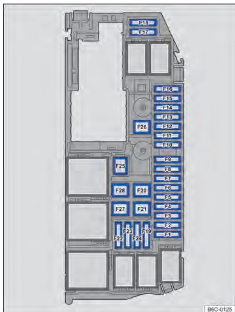
Fig. 145 No compartimento do motor: disposição dos fusíveis.
