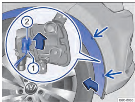
Fig. 137 Na caixa de roda dianteira: acesso à lâmpada incandescente do farol de neblina.
