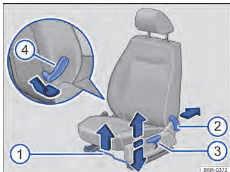
Fig. 69 No banco dianteiro: comandos.
