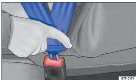
Fig. 35 Introduzir a lingueta do cinto de segurança no fecho do cinto de segurança.
