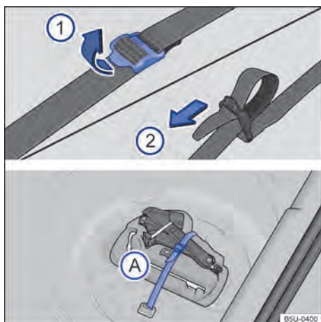
Fig. 128 No compartimento de bagagem: cinta de fixação da caixa de ferramentas e caixa de ferramentas de bordo.
