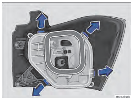
Fig. 139 Lanterna traseira: desinstalar o suporte das lâmpadas
