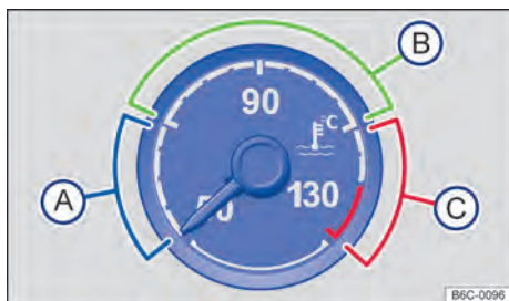
Fig. 18 Indicador de temperatura do líquido de arrefecimento do motor no instrumento combinado analógico (variante 2): (A) área fria; (B) área normal; (C) área de alerta.
