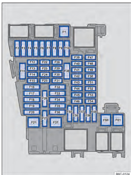
Fig. 143 No painel de instrumentos: disposição dos fusíveis.
