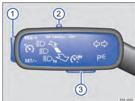
Fig. 104 À esquerda na coluna de direção: alavanca com interruptor e botões de comando do GRA.
