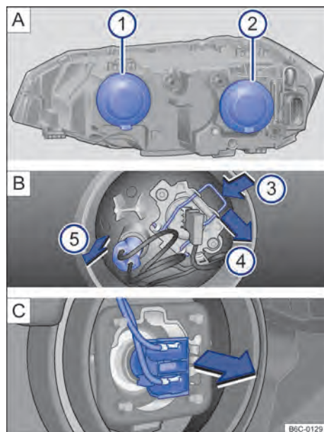
Fig. 134 No compartimento do motor: ⓘ farol alto e luz de posição e ⓘ farol baixo. ►
