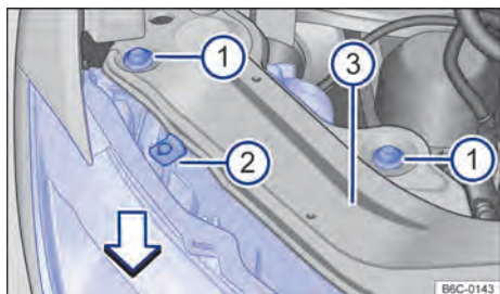
Fig. 133 No compartimento do motor: parafusos de fixação do farol dianteiro.
