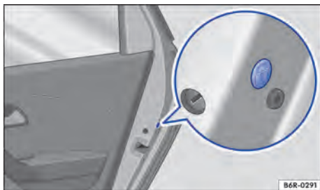
Fig. 62 Na porta traseira: travamento de emergência, coberto por uma vedação de borracha.
