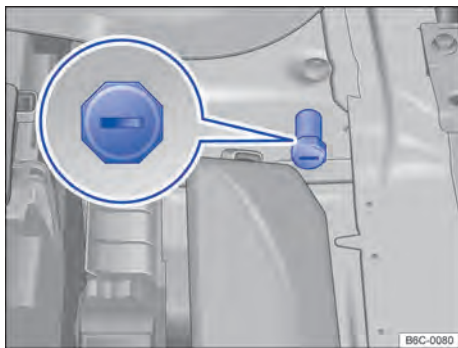
Fig. 182 No compartimento do motor: ponto de auxílio à partida (ponto de aterramento).
