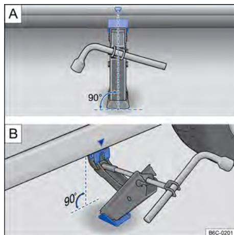
Fig. 204 Pontos de apoio do macaco e macaco posicionado no lado esquerdo traseiro do veículo.
