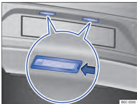
Fig. 190 No para-choque traseiro: lanterna da placa de licença.
