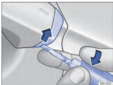
Fig. 58 Maçaneta da porta do condutor: levantar a capa de cobertura.
