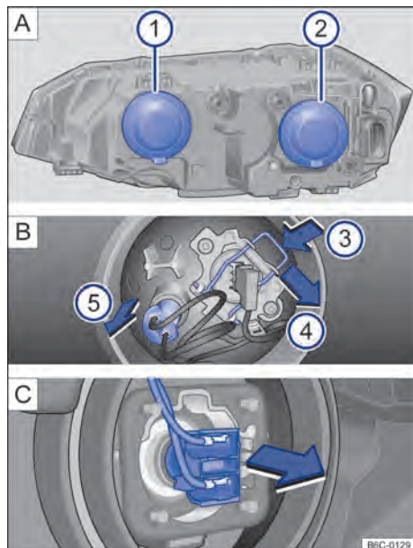
Fig. 184 No compartimento do motor: ① farol alto e luz de posição e ② farol baixo.
