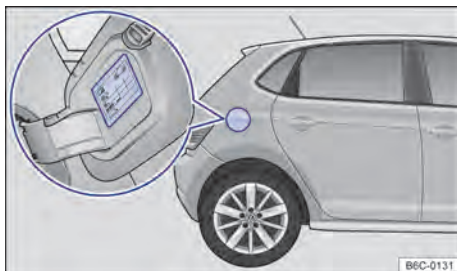
Fig. 214 Na parte interna da portinhola do tanque de combustível: etiqueta com a pressão dos pneus.
