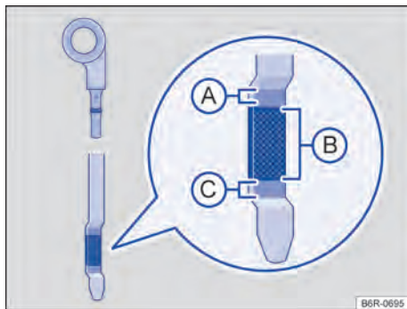
Fig. 205 Vareta de medição do óleo com marcas de nível do óleo do motor.
