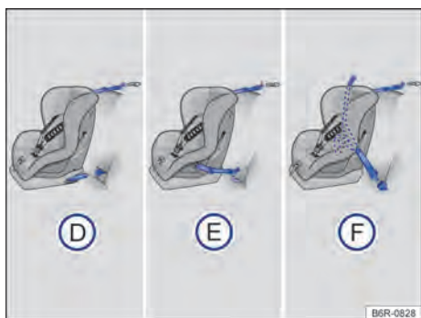
Fig. 44 No banco traseiro: as figuras D e E mostram o princípio da fixação do sistema de retenção para crianças nos olhais de retenção inferiores e com o cinto de fixação superior. A figura F mostra a fixação do sistema de retenção para crianças com o cinto de segurança do veículo e com o cinto de fixação superior.
