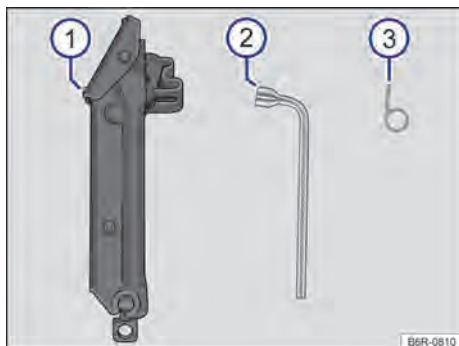
Fig. 179 Componentes das ferramentas de bordo.
