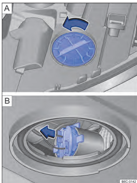
Fig. 185 Farol dianteiro, por baixo: cobertura do indicador de direção.
