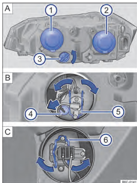
Fig. 186 No compartimento do motor: ① farol alto e luz de posição, ② farol baixo e ③ indicador de direção.
