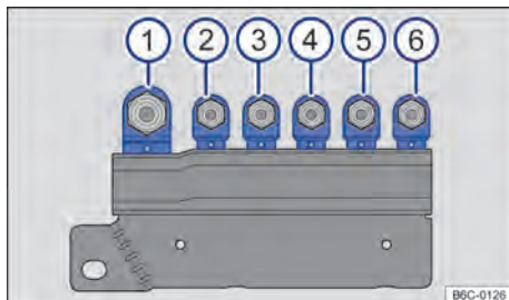
Fig. 196 No compartimento do motor em cima da bateria: disposição dos fusíveis.
