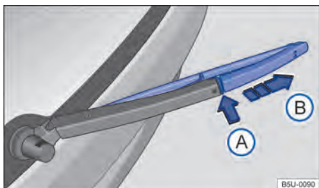
Fig. 182 Substituir a palheta do limpador do vidro traseiro.
