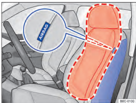
Fig. 42 Lateralmente no banco dianteiro: localização de instalação e área de expansão dos airbags laterais.
