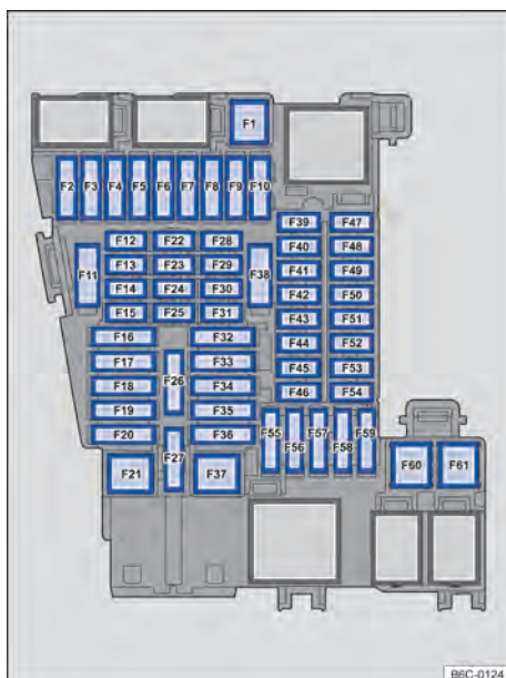
Fig. 193 No painel de instrumentos: disposição dos fusíveis.
