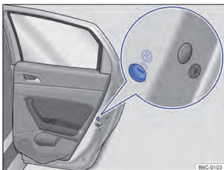
Fig. 48 Na porta traseira (lado direito): localização da trava de segurança para crianças.
