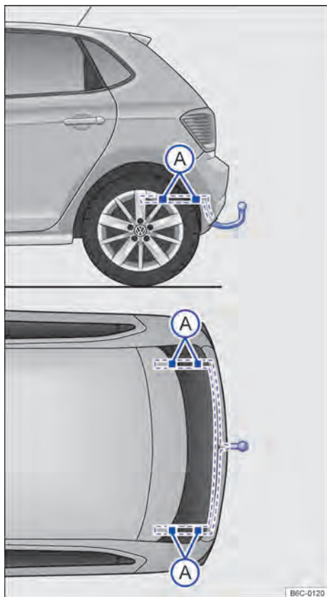
Fig. 175 Pontos de fixação para instalar um dispositivo de reboque posteriormente.
