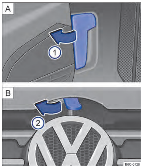
Fig. 201 [A] Alavanca de destravamento da tampa do compartimento do motor na área para os pés do lado do condutor. [B] Alavanca de destravamento na parte interna da tampa do compartimento do motor. ►
