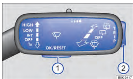
Fig. 19 Veículos sem volante multifunções: botão ① na alavanca dos limpadores dos vidros para confirmação dos itens de menu e chave ② para alternar entre os menus.
