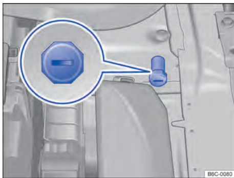
Fig. 199 No compartimento do motor: ponto de auxílio à partida (ponto de aterramento).
