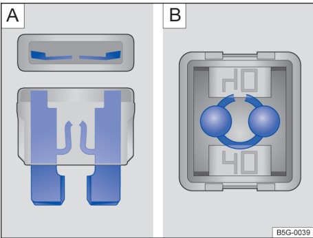
Fig. 144 Fusível queimado: A) fusível plano, B) fusível de bloqueio.
