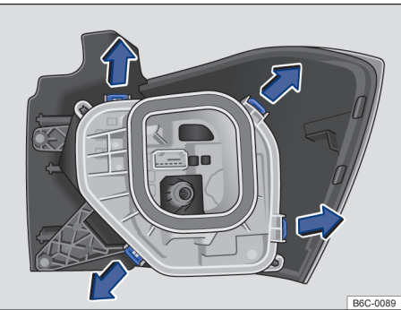
Fig. 136 Lanterna traseira: desinstalar o suporte das lâmpadas
