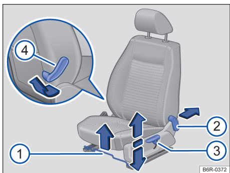
Fig. 66 No banco dianteiro: comandos.
