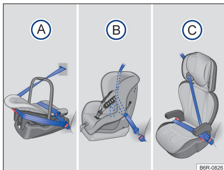
Fig. 42 As ilustrações (A), (B) e (C) mostram a fixação do sistema de retenção para crianças apenas com o cinto de segurança do veículo.
