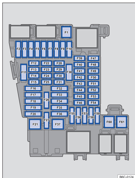
Fig. 141 No painel de instrumentos: disposição dos fusíveis.
