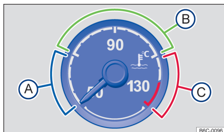
Fig. 17 Indicador de temperatura do líquido de arrefecimento do motor no instrumento combinado analógico (variante 2): (A) área fria; (B) área normal; (C) área de alerta.
