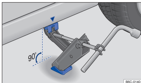
Fig. 168 Pontos de apoio do macaco e macaco posicionado no lado esquerdo traseiro do veículo.
