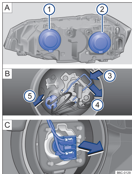
Fig. 131 No compartimento do motor: ① farol alto e luz de posição e ② farol baixo.
