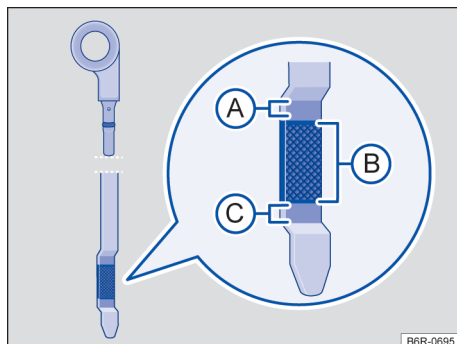
Fig. 151 Vareta de medição do óleo com marcas de nível do óleo do motor.
