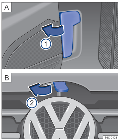
Fig. 147 [A] Alavanca de destravamento da tampa do compartimento do motor na área para os pés do lado do condutor. [B] Alavanca de destravamento na parte interna da tampa do compartimento do motor. ►
