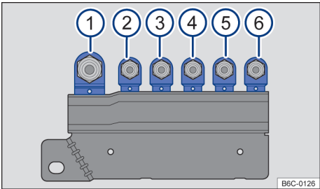
Fig. 143 No compartimento do motor em cima da bateria: disposição dos fusíveis.
