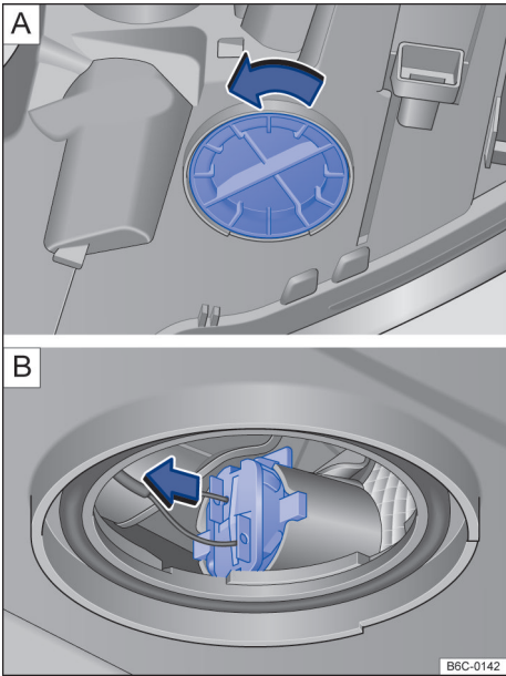
Fig. 132 Farol dianteiro, por baixo: cobertura do indicador de direção.
