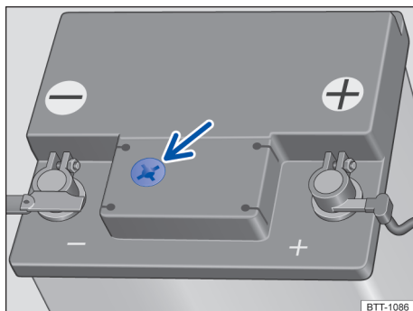
Fig. 156 No compartimento do motor: exemplo de posição do visor no lado superior da bateria do veículo.
