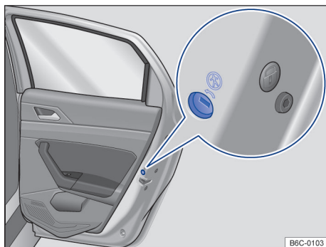
Fig. 47 Na porta traseira (lado direito): localização da trava de segurança para crianças.
