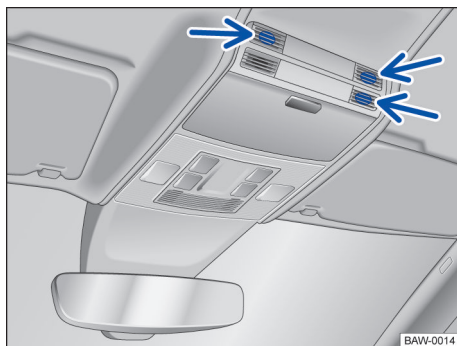
Fig. 57 No consola do teto: sensores de monitoramento do interior do veículo (setas).
