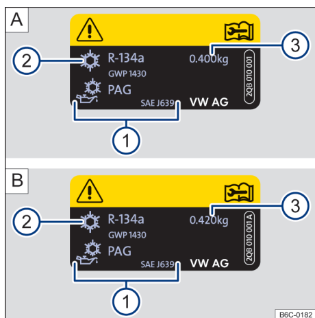
Fig. 175 A: informações do ar-condicionado - motor 1.0L. B: informações do ar-condicionado - motor 1.0L TSI e motor 1.6L.
