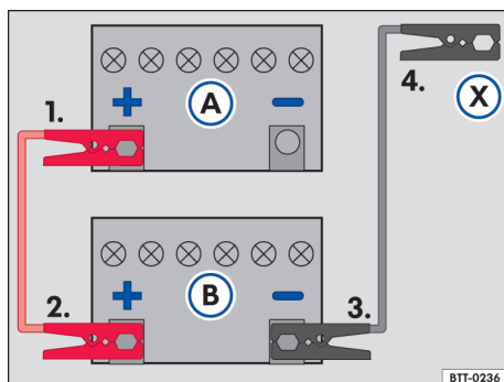
Fig. 146 Esquema para a conexão dos cabos auxiliares de partida: bateria do veículo descarregada (A) e bateria do veículo fornecedora de corrente (B).
