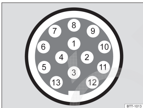
Fig. 136 Representação esquemática: disposição dos pinos da tomada do reboque.
