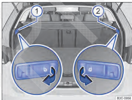
Fig. 112 No compartimento de bagagem: alavanca de destravamento à distância para a parte esquerda ① e para a parte direita ② do encosto do banco traseiro.
