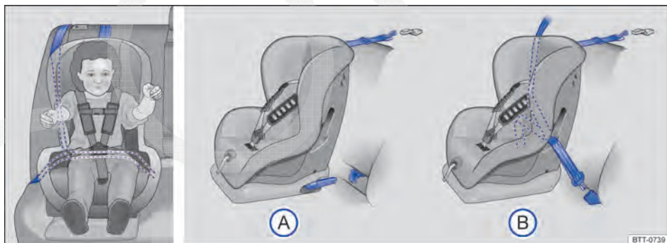
Fig. 85 Nos bancos traseiros: a figura A mostra o princípio da fixação do sistema de retenção para crianças nos olhais de retenção inferiores e com o cinto de fixação superior. A figura B mostra a fixação do sistema de retenção para crianças com o cinto de segurança do veículo.
