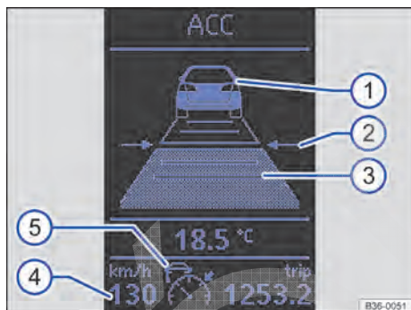
Fig. 194 No display do instrumento combinado: ACC ativado, veículo adiante reconhecido, distância regulada.
