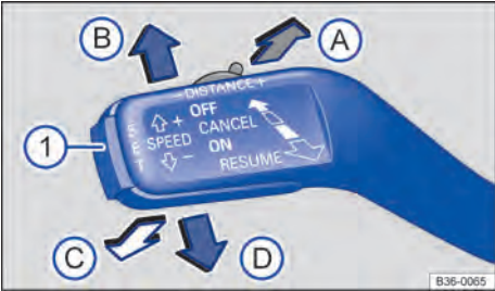
Fig. 196 Alavanca de operação ACC à esquerda na coluna de direção: regular a velocidade.
