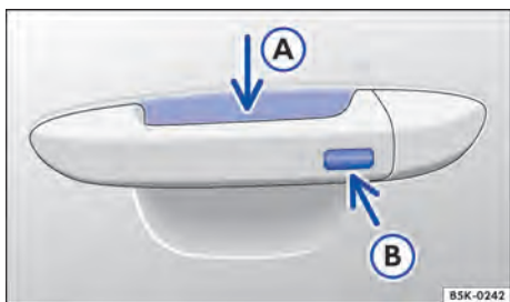
Fig. 30 Sistema de travamento e de partida Keyless Access sem chave: superfície dos sensores (A) para destravamento na parte interna da maçaneta da porta e superfície dos sensores (B) para travamento na parte externa da maçaneta da porta.
