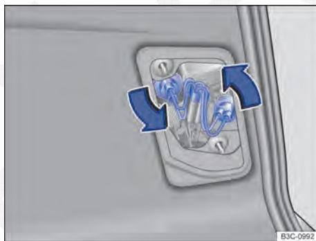
Fig. 256 Na tampa do compartimento de bagagem: desinstalar as lâmpadas incandescentes.
