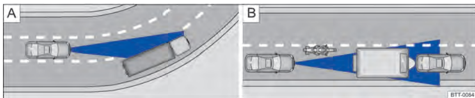
Fig. 175 A: veículo na área de uma curva. B: motocicleta à frente fora da área de alcance do sensor do radar.
