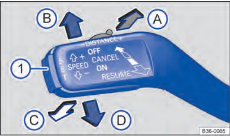
Fig. 172 Alavanca de operação ACC à esquerda na coluna de direção: regular a velocidade.
