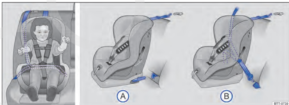
Fig. 78 Nos bancos traseiros: a figura A mostra o princípio da fixação do sistema de retenção para crianças nos olhais de retenção inferiores e com o cinto de fixação superior. A figura B mostra a fixação do sistema de retenção para crianças com o cinto de segurança do veículo.
