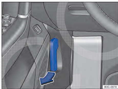
Fig. 198 Na área para os pés no lado do condutor: alavanca de destravamento da tampa do compartimento do motor.
