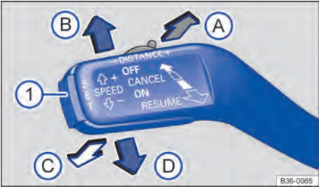
Fig. 174 Alavanca de operação ACC à esquerda na coluna de direção: regular a velocidade.
