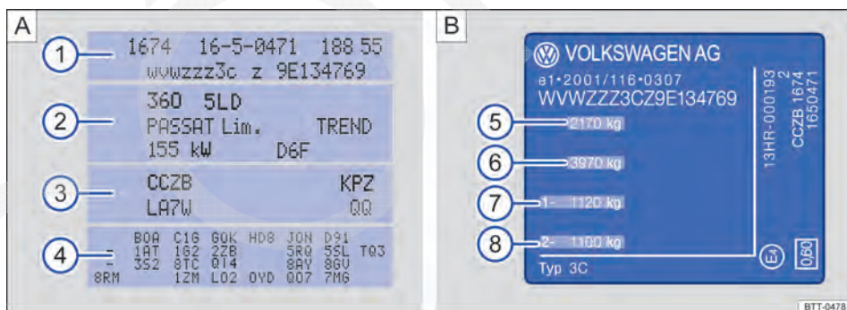
Fig. 17 (A) Etiqueta de dados do veículo: na imagem de exemplo, com o código do motor CCZB ③. (B) Plaqueta de identificação.
