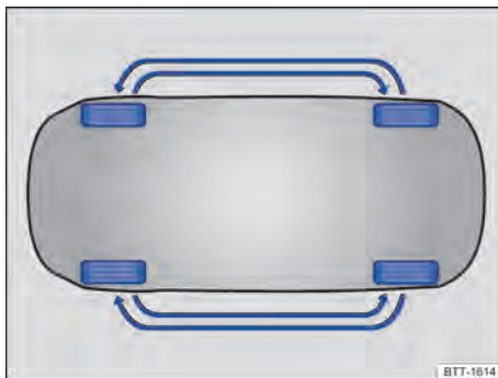
Fig. 186 Esquema para a troca das rodas.
