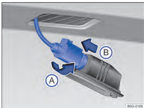
Fig. 166 Lanterna da placa de licença: desinstalar o suporte da lâmpada.
