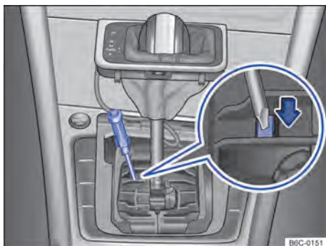
Fig. 91 Desinstalar a cobertura da alavanca seletora e destravar o bloqueio da alavanca seletora emergencialmente.
