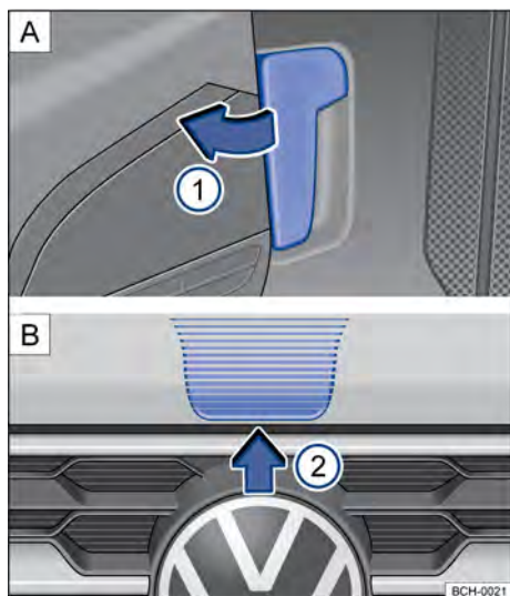
Fig. 175 [A] Alavanca de destravamento da tampa do compartimento do motor na área para os pés do lado do condutor. [B] Alavanca de destravamento na parte interna da tampa do compartimento do motor.
