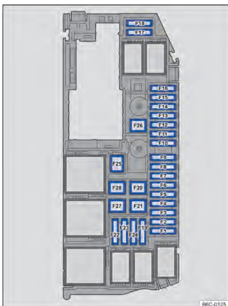
Fig. 170 No compartimento do motor: disposição dos fusíveis.
