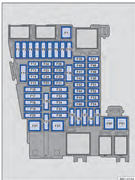
Fig. 168 No painel de instrumentos: disposição dos fusíveis.
