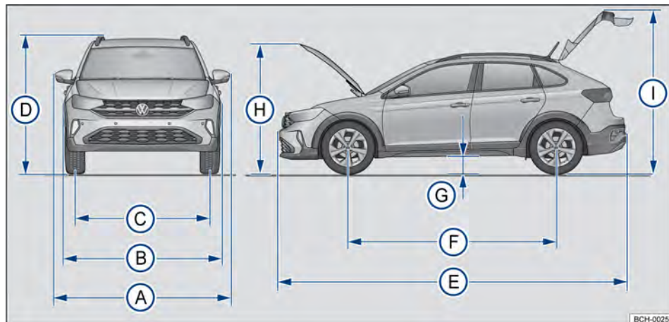
Fig. 200 Dimensões.
