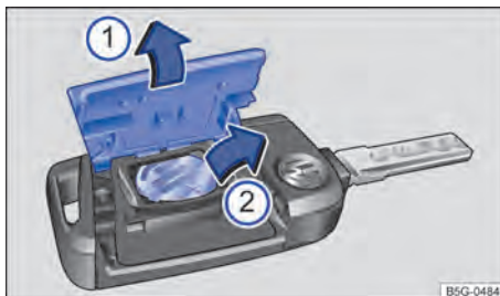
Fig. 49 Chave do veículo: substituir a bateria.
