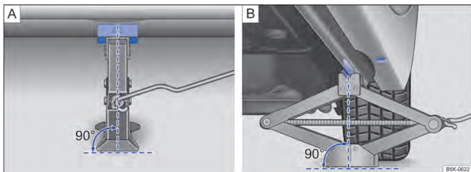
Fig. 247 Macaco posicionado no lado esquerdo traseiro do veículo.
