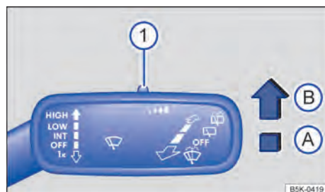
Fig. 101 Na alavanca dos limpadores dos vidros à direita da coluna de direção: ajustar o sensor de chuva e de luz ①.
