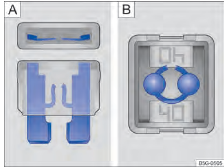
Fig. 214 Fusível queimado: A) fusível plano, B) fusível de bloqueio.
