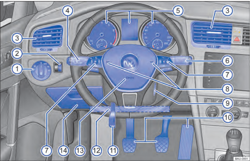
Fig. 8 Vista geral do lado do condutor.
