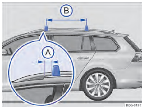
Fig. 191 Longarina do bagageiro do teto: fixação das barras de suporte (Golf Variant).
