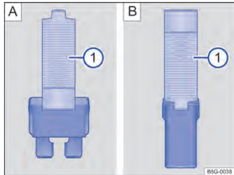
Fig. 215 Retirar ou colocar o fusível com a pinça de plástico: A) fusível plano, B) fusível de bloqueio.
