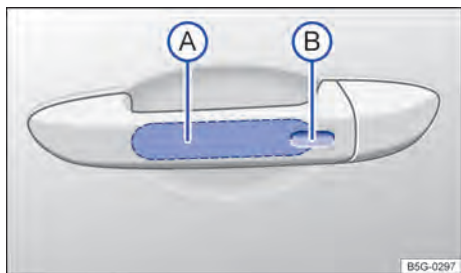
Fig. 65 Sistema de travamento e de partida Keyless Access sem chave: superfície do sensor (A) para destravamento na parte interna da maçaneta da porta e superfície do sensor (B) para travamento na parte externa da maçaneta da porta.
