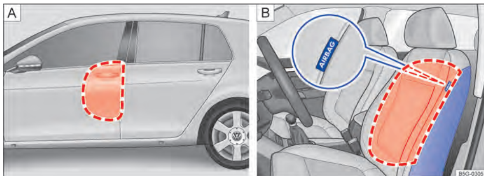
Fig. 44 A No lado esquerdo do veículo: áreas de expansão do airbag lateral. B Lateralmente no banco dianteiro: local de instalação e área de expansão dos airbags laterais.
