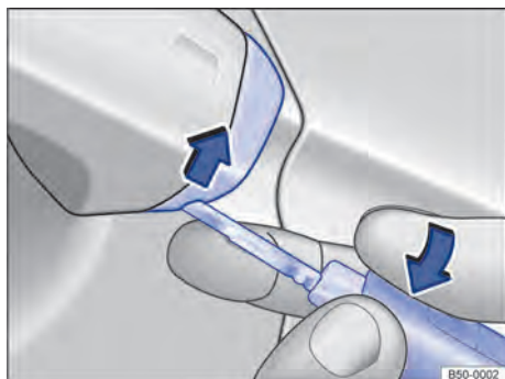
Fig. 70 Maçaneta da porta do condutor: levantar a capa de cobertura.
