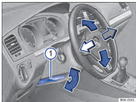
Fig. 79 Embaixo do volante no revestimento da coluna de direção: alavanca de ajuste mecânico da posição do volante.
