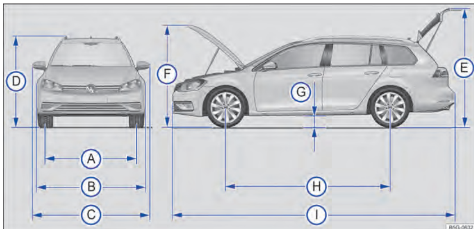
Fig. 257 Dimensões.
