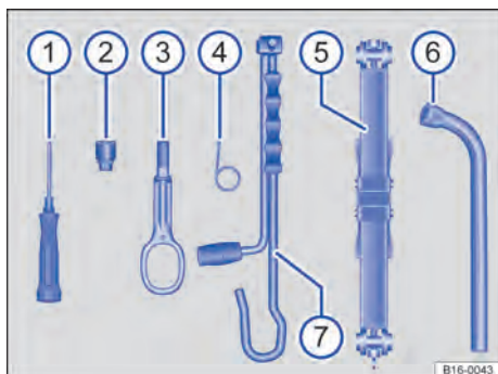
Fig. 196 Componentes das ferramentas de bordo.
