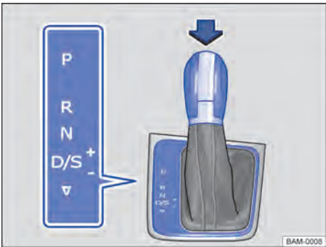
Fig. 123 Alavanca seletora da transmissão automática com botão bloqueador (seta).
