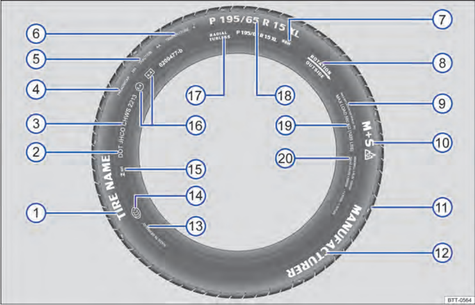
Fig. 237 Inscrição internacional dos pneus.
