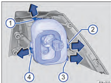
Fig. 201 Lanterna traseira da carroceria: desinstalar o suporte da lâmpada. Tiras de travamento (1) a (4).
