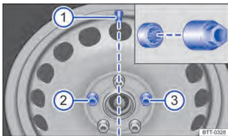
Fig. 243 Troca de roda: válvula do pneu ① e posições de montagem do parafuso de roda antifurto ② ou ③.
