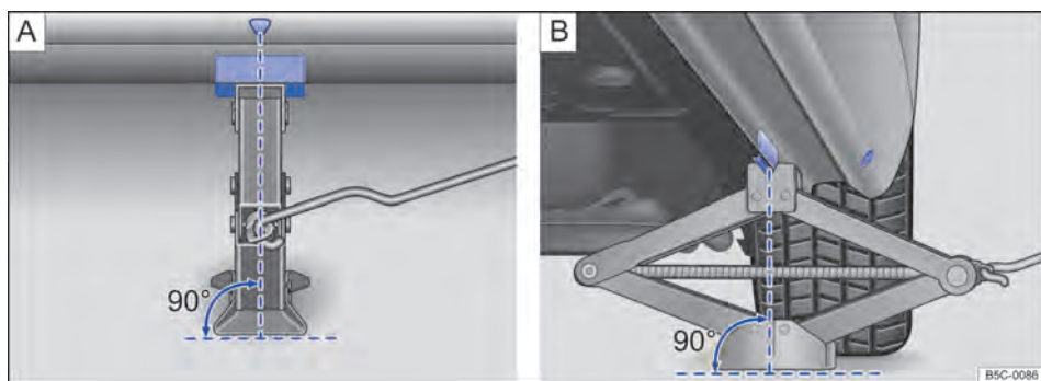
Fig. 245 Macaco posicionado no lado esquerdo traseiro do veículo.
