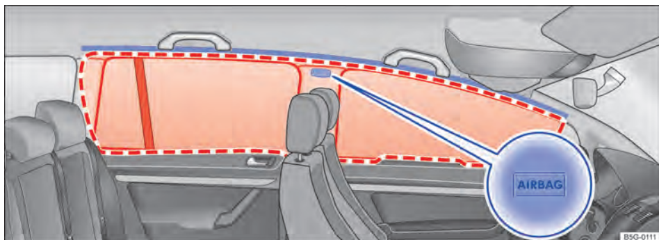
Fig. 46 No lado esquerdo do veículo: local de instalação e área de expansão do airbag para cabeça (Golf Variant).
