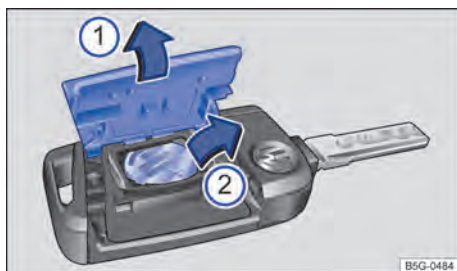
Fig. 61 Chave do veículo: substituir a pilha botão.
