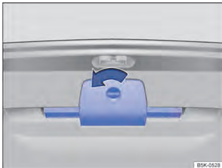
Fig. 56 Na tampa do compartimento de bagagem: suporte para o triângulo de segurança.
