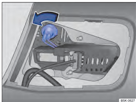
Fig. 209 Na tampa do compartimento de bagagem: remover o suporte da lâmpada.
