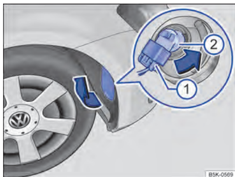
Fig. 199 No protetor da caixa de roda dianteiro direito: substituir a lâmpada incandescente no farol.
