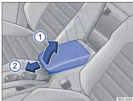
Fig. 90 Descansa-braço central dianteiro.
