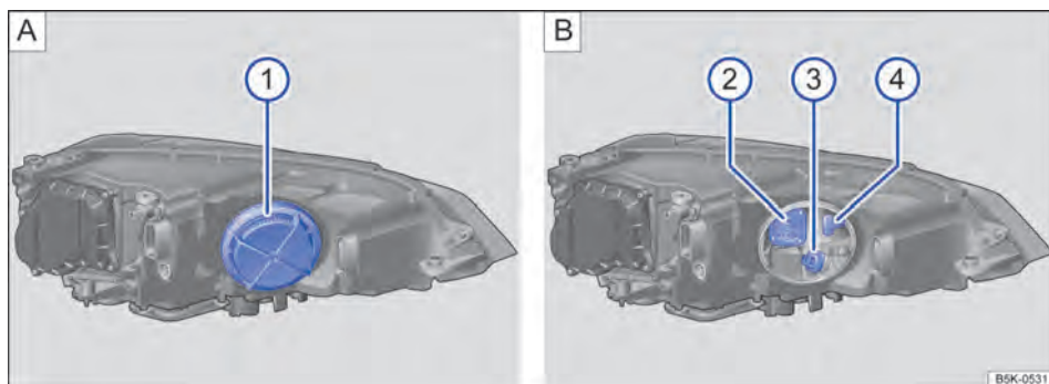
Fig. 198 No compartimento do motor: ① cobertura no farol dianteiro esquerdo, ② farol de conversão, ③ indicadores de direção, ④ luz de posição e farol de rodagem diurna.
