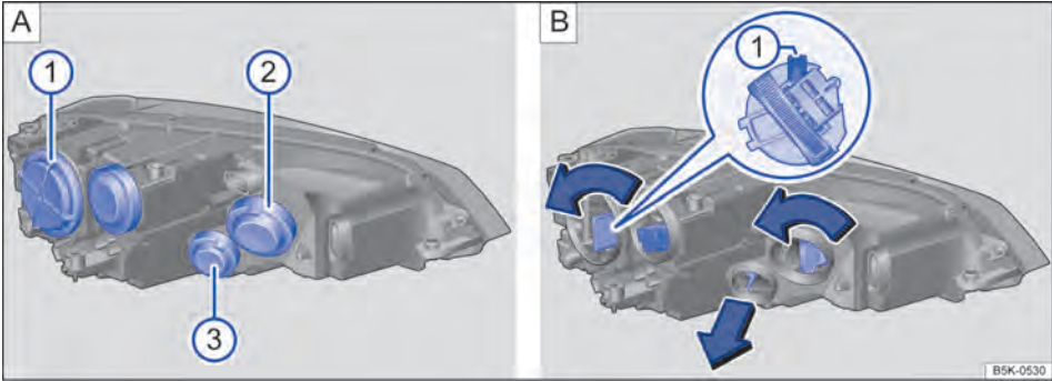
Fig. 197 No compartimento do motor: coberturas do farol dianteiro esquerdo. 1 farol baixo, 2 farol alto e luz de posição, bem como farol de rodagem diurna, 3 indicador de direção.
