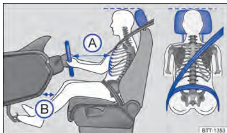
Fig. 27 Distância correta do condutor em relação ao volante, posição correta do cadarço do cinto de segurança e ajuste correto do apoio para cabeça.
