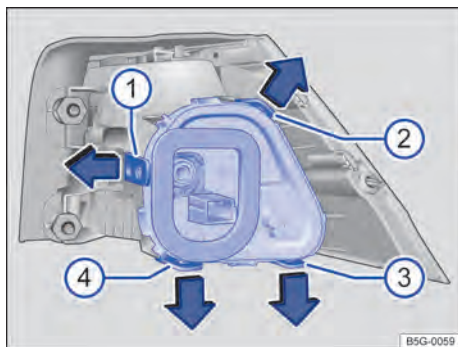
Fig. 203 Lanterna traseira da carroceria: desinstalar o suporte da lâmpada. Tiras de travamento ① a ④.
