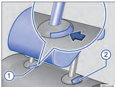
Fig. 89 Desinstalar o apoio para cabeça traseiro.
