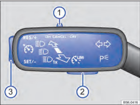
Fig. 149 À esquerda na coluna de direção: interruptores e botões para comandar o GRA.
