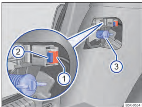
Fig. 225 Lateralmente no compartimento de bagagem: desinstalar a lanterna traseira.
