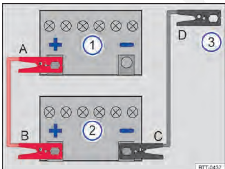
Fig. 230 Esquema para a conexão dos cabos auxiliares de partida em veículos auxiliares de partida sem sistema Start-Stop: bateria do veículo 12 V descarregada ① e bateria do veículo 12 V fornecedora de corrente ②.
