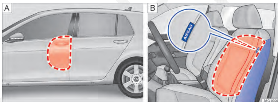
Fig. 70 A No lado esquerdo do veículo: áreas de expansão do airbag lateral. B Lateralmente no banco dianteiro: local de instalação e área de expansão dos airbags laterais.
