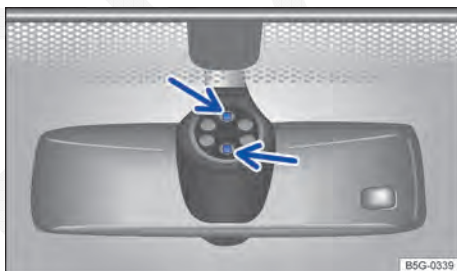
Fig. 87 No para-brisa acima do espelho retrovisor interno: superfície sensível do sensor de chuva e de luz.
