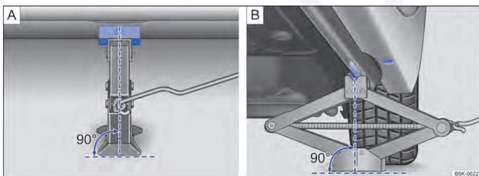
Fig. 211 Macaco posicionado no lado esquerdo traseiro do veículo.
