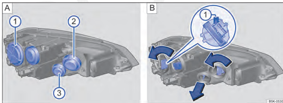
Fig. 218 No compartimento do motor: coberturas do farol dianteiro esquerdo. ❶ farol baixo, ❷ farol alto e luz de posição, bem como farol de rodagem diurna, ❸ indicador de direção.
