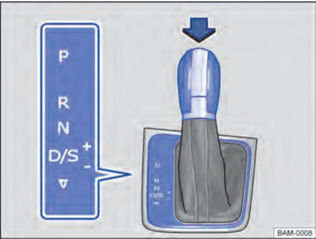
Fig. 124 Alavanca seletora da transmissão automática com botão bloqueador (seta).
