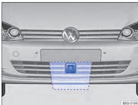
Fig. 157 Área que deve ficar livre ao redor do sensor do radar.
