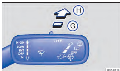
Fig. 84 À direita da coluna de direção: comandar o limpador do vidro traseiro.
