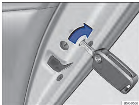
Fig. 197 Na parte dianteira da porta traseira direita: travamento de emergência do veículo com a chave do veículo.
