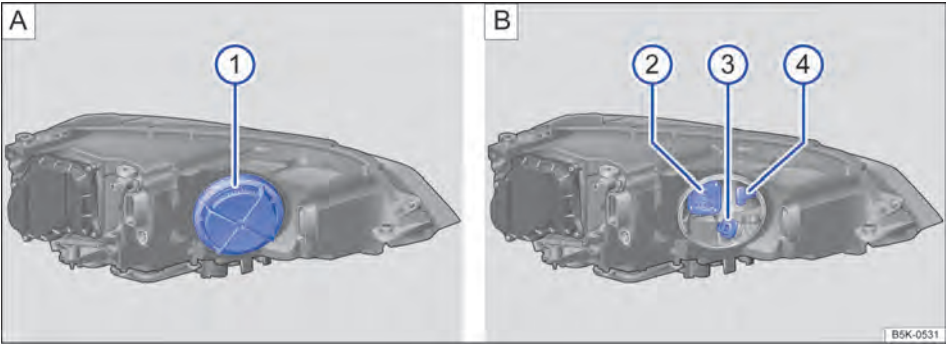
Fig. 219 No compartimento do motor: ① cobertura no farol dianteiro esquerdo, ② farol de conversão, ③ indicadores de direção, ④ luz de posição e farol de rodagem diurna.
