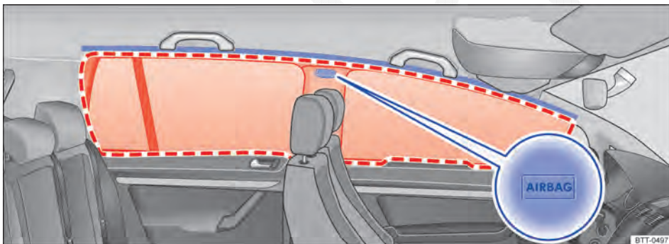
Fig. 71 No lado esquerdo do veículo: local de instalação e área de expansão do airbag para cabeça.
