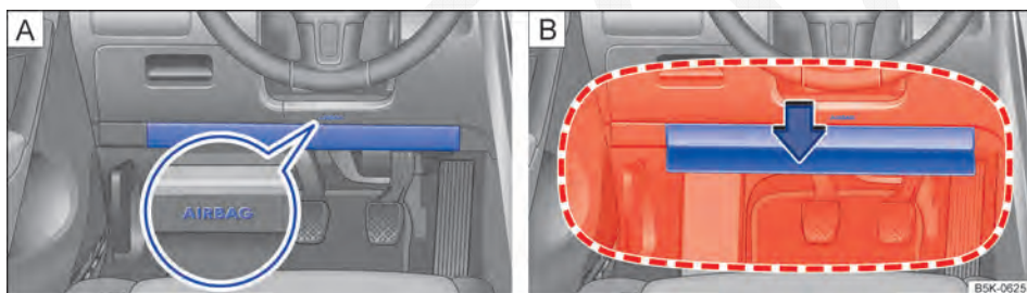
Fig. 72 No lado do condutor: A local de instalação e B área de expansão do airbag para joelhos.
