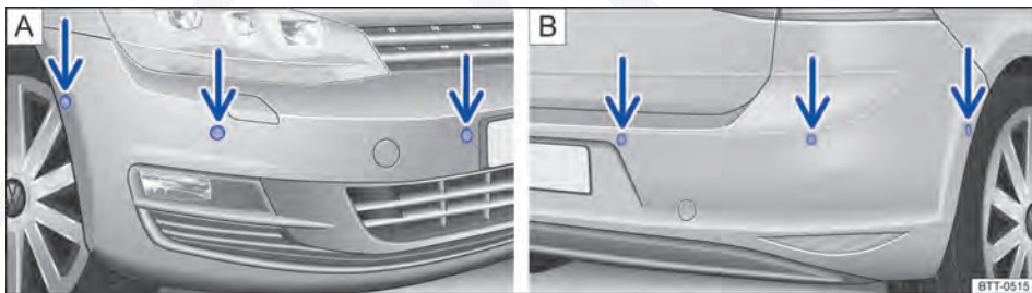
Fig. 135 Nos para-choques dianteiro e traseiro: sensores de ultrassom do Park Pilot nos arredores do veículo.
