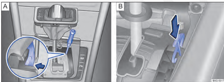
Fig. 201 Embaixo da cobertura do quadro da alavanca seletora: destravar o bloqueio da alavanca seletora emergencialmente (variante A) e (variante B).
