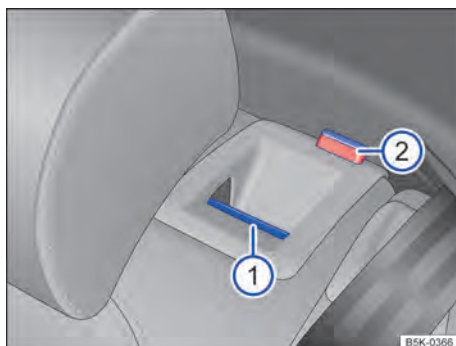
Fig. 92 No encosto do banco traseiro: botão de destravamento ①, marcação vermelha ②.
