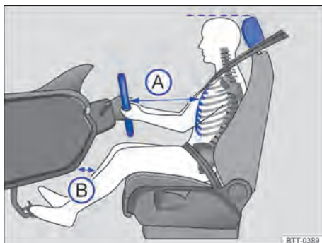
Fig. 40 A distância correta (A) entre o condutor e o volante deve ser de, no mínimo, 25 cm. Na área dos joelhos, a distância (B) ao painel de instrumentos deve ser, no mínimo, 10 cm.
