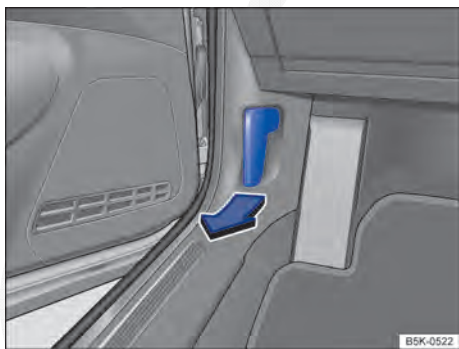
Fig. 173 No área para os pés no lado do condutor: alavanca de destravamento da tampa do compartimento do motor.
