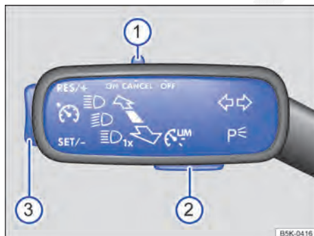
Fig. 152 À esquerda na coluna de direção: interruptores e botões para comandar o limitador de velocidade.
