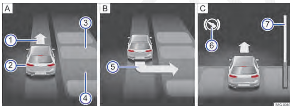
Fig. 146 No display do instrumento combinado: entrar na vaga de estacionamento transversalmente à pista. A Procurar vaga transversal, B posição em relação à entrada na vaga de estacionamento, C manobrar.
