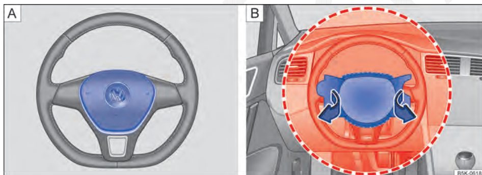
Fig. 67 [A] Local de instalação e [B] área de expansão do airbag frontal do condutor.
