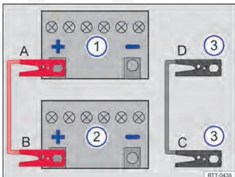
Fig. 231 Esquema para a conexão dos cabos auxiliares de partida em veículos auxiliares de partida com sistema Start-Stop: bateria do veículo 12 V descarregada ① e bateria do veículo 12 V fornecedora de corrente ②.
