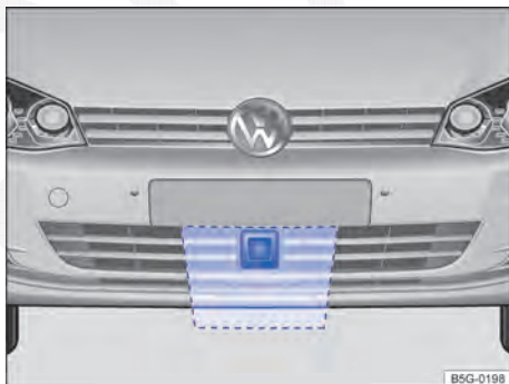
Fig. 164 Área que deve ficar livre ao redor do sensor do radar.
