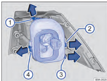
Fig. 226 Lanterna traseira na carroceria: desinstalar o suporte da lâmpada. Tiras de travamento ① bis ④.
