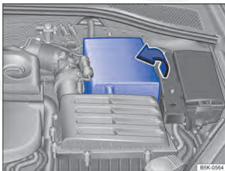
Fig. 180 No compartimento do motor: rebater para fora a capa da bateria do veículo 12 V.
