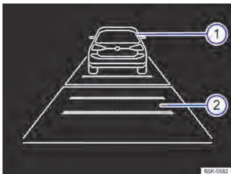
Fig. 154 No display do instrumento combinado: ACC não ativo temporariamente, veículo à frente reconhecido, distância temporal regulada.
