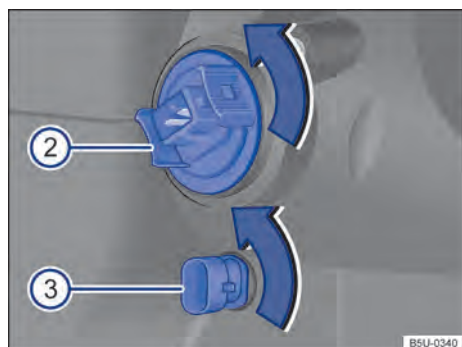
Fig. 153 No compartimento do motor: vista traseira do farol dianteiro (2) indicadores de direção e (3) luz de posição.
