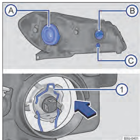
Fig. 152 No compartimento do motor: vista traseira do farol dianteiro com cobertura de borracha (lado esquerdo da ilustração) - (A) farol baixo / alto, (B) indicadores de direção e (C) luz de posição. Vista traseira do farol dianteiro sem a cobertura de borracha (lado direito da ilustração): (1) mola de travamento da lâmpada incandescente do farol baixo / alto.
