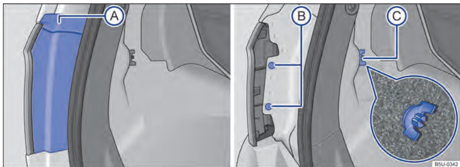
Fig. 157 No compartimento de bagagem: A desinstalar cobertura, B retirar os dois parafusos de fixação e C retirar o parafuso borboleta (lupa).
