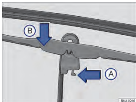
Fig. 148 Substituir as palhetas dos limpadores do para-brisa.
