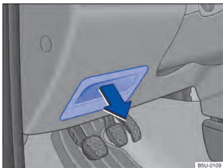
Fig. 161 No lado do condutor no painel de instrumentos: cobertura da caixa de fusíveis.
