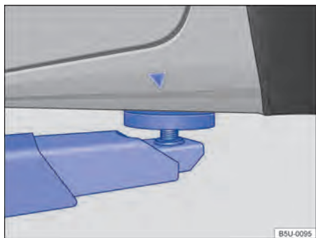
Fig. 192 Pontos de apoio traseiros para a suspensão com plataforma elevatória ou com macaco.
