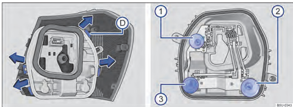
Fig. 158 Lanterna traseira: D desinstalar o suporte das lâmpadas e 1 , 2 e 3 desinstalar as lâmpadas.
