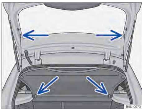
Fig. 142 No compartimento de bagagem: remover e instalar a cobertura do compartimento de bagagem. ▶
