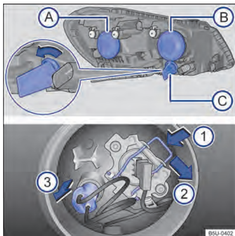
Fig. 154 No compartimento do motor: vista traseira do farol dianteiro com cobertura de borracha (lado esquerdo da ilustração) - (A) farol baixo, (B) farol alto e luz de posição, e (C) indicador de direção. Vista traseira do farol dianteiro sem a cobertura de borracha (lado direito da ilustração): 1 mola de travamento da lâmpada incandescente do farol e 2 luz de posição.
