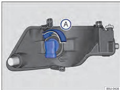
Fig. 156 Atrás do para-choque dianteiro: acesso à lâmpada incandescente do farol de neblina.
