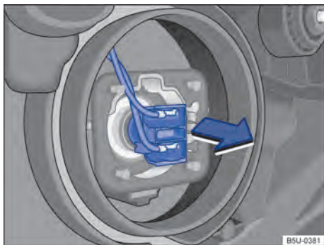
Fig. 155 Acesso à lâmpada incandescente do farol baixo.
