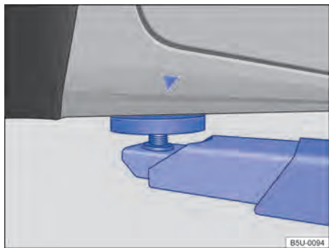
Fig. 191 Pontos de apoio dianteiros para a suspensão com plataforma elevatória ou com macaco.
