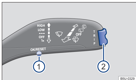
Fig. 17 Veículos sem volante multifunções: tecla ① na alavanca dos limpadores dos vidros para confirmação dos itens de menu e chave ② para alternar entre os menus.
