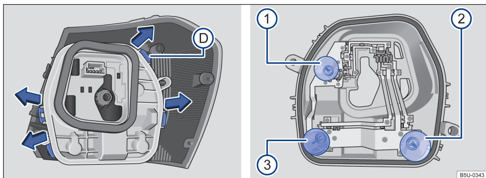
Fig. 113 Lanterna traseira: D) desinstalar o suporte das lâmpadas e ❶, ❷ e ❸ desinstalar as lâmpadas.
