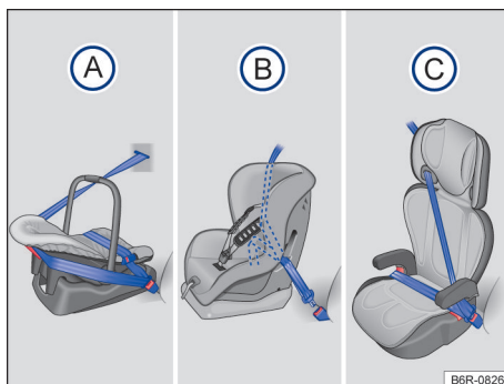
Fig. 35 As ilustrações A, B e C mostram a fixação do sistema de retenção para crianças apenas com o cinto de segurança do veículo.
