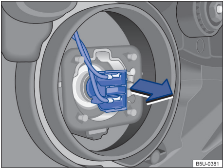
Fig. 110 Acesso à lâmpada incandescente do farol baixo.
