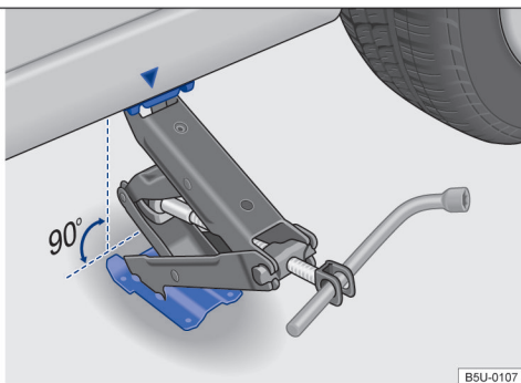
Fig. 143 Pontos de apoio do macaco e macaco posicionado no lado esquerdo traseiro do veículo.
