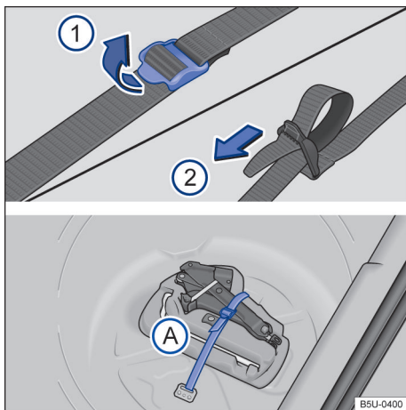
Fig. 103 No compartimento de bagagem: cinto de fixação da caixa de ferramentas e caixa de ferramentas de bordo.
