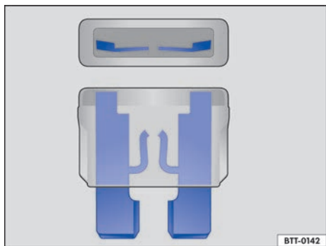
Fig. 165 Representação de um fusível queimado.
