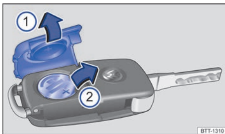
Fig. 45 Chave do veículo com comando remoto: 1 Abrir a tampa do alojamento da bateria. 2 Remover a bateria.
