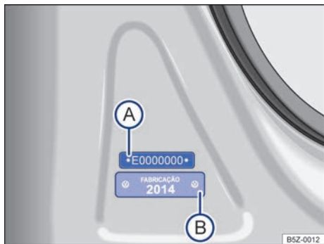
Fig. 201 Na coluna da porta dianteira direita: etiqueta com o número de identificação do veículo parcial (A) e etiqueta de identificação do ano de fabricação (B).
