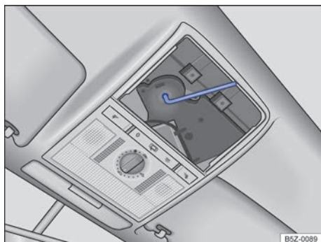
Fig. 59 Parafuso sextavado para fechamento do teto solar.
