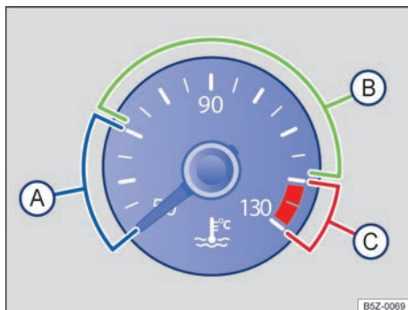
Fig. 14 Indicador de temperatura do líquido de arrefecimento do motor no instrumento combinado: (A) área fria; (B) área normal; (C) área de alerta.
