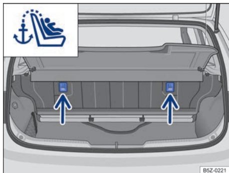
Fig. 37 Olhalis de retenção para o cinto de fixação superior no lado de trás do banco traseiro.
