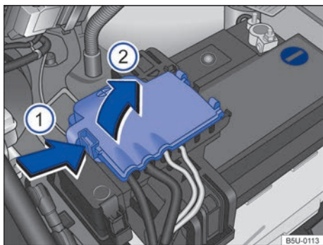
Fig. 167 Compartimento do motor: acesso ao terminal positivo da bateria.
