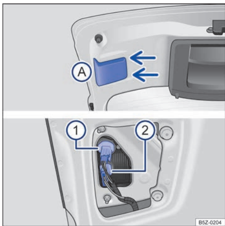
Fig. 158 Lanterna traseira: (A) desinstalar a cobertura e (1) e (2) desinstalar as lâmpadas.
