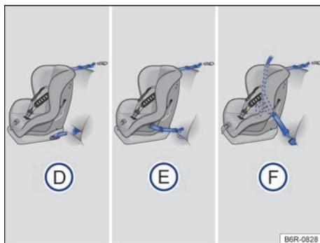
Fig. 35 No banco traseiro: (D) e (E) mostram o princípio da fixação do sistema de retenção para crianças nos olhais de retenção inferiores e com o cinto de fixação superior. A figura (F) mostra a fixação do sistema de retenção para crianças com o cinto de segurança do veículo e com o cinto de fixação superior.
