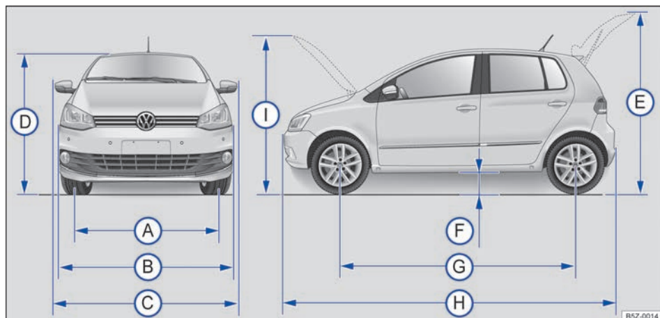
Fig. 204 Dimensões.
