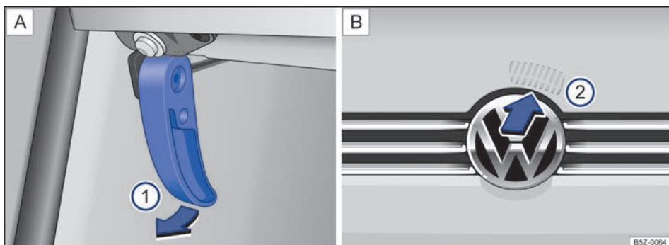
Fig. 175 A: alavanca de destravamento na área para os pés do lado do condutor ①. B: alavanca de destravamento na parte interna da tampa do compartimento do motor ②.
