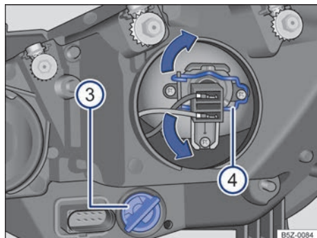
Fig. 152 No compartimento do motor: vista traseira do farol dianteiro direito sem cobertura de borracha: 3 indicadores de direção e 4 farol baixo.
