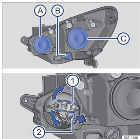
Fig. 151 No compartimento do motor: vista traseira do farol dianteiro direito com cobertura de borracha (esquerda): A farol alto e luz de posição, B indicadores de direção e C farol baixo. Vista traseira do farol dianteiro direito sem cobertura de borracha (direita): 1 farol alto, 2 luz de posição.
