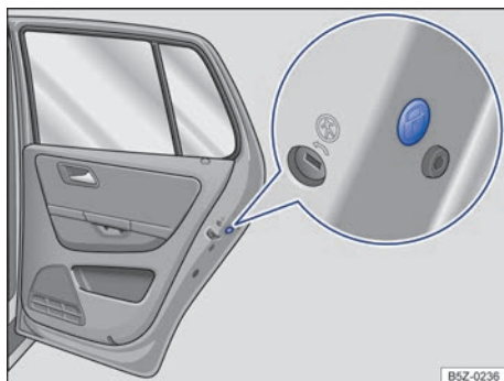
Fig. 52 Na porta traseira: travamento de emergência, coberto por uma vedação de borracha.
