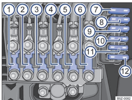
Fig. 164 Caixa de fusíveis.
