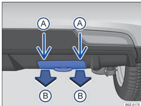
Fig. 174 No para-choque traseiro à direita: argola de reboque traseira - para-choque com cobertura removível. ▶
