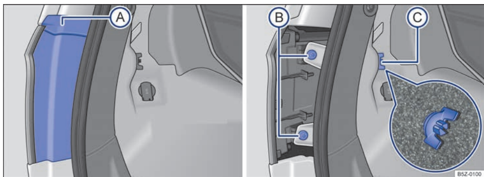
Fig. 156 Lateralmente no compartimento de bagagem: A desinstalar a cobertura, B retirar os dois parafusos e C retirar o parafuso borboleta (lupa).
