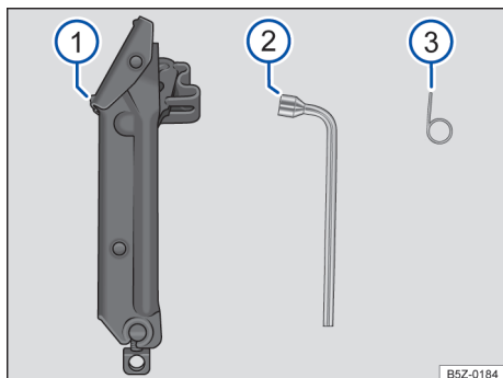
Fig. 114 Representação esquemática: componentes das ferramentas de bordo.
