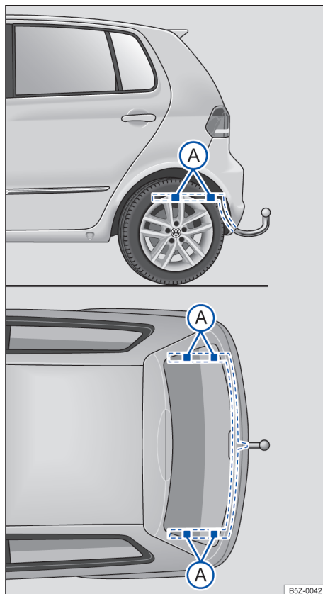
Fig. 110 Pontos de fixação para instalar um dispositivo de reboque posteriormente.
