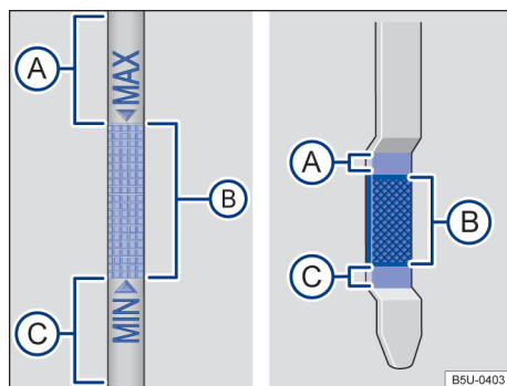
Fig. 145 Vareta de medição do óleo com marcas de nível do óleo do motor.
