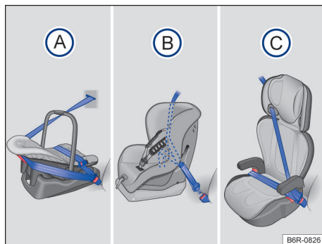
Fig. 35 As ilustrações A, B e C mostram a fixação do sistema de retenção para crianças apenas com o cinto de segurança do veículo.
