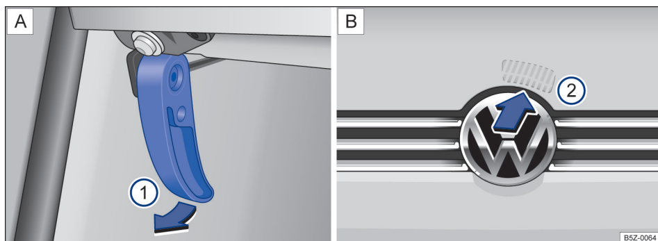
Fig. 142 A: alavanca de destravamento na área para os pés do lado do condutor (1). B: alavanca de destravamento na parte interna da tampa do compartimento do motor (2).
