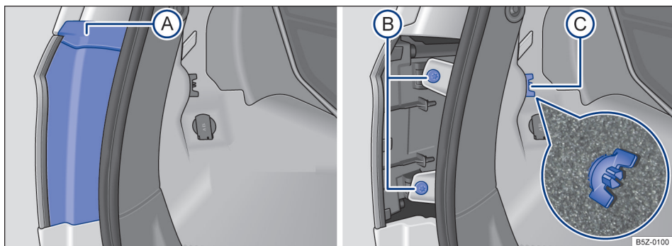
Fig. 123 Lateralmente no compartimento de bagagem: A desinstalar a cobertura, B retirar os dois parafusos e C retirar o parafuso borboleta (lupa).
