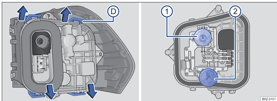
Fig. 124 Lanterna traseira: D desinstalar o suporte das lâmpadas e 1 e 2 desinstalar as lâmpadas incandescentes.
