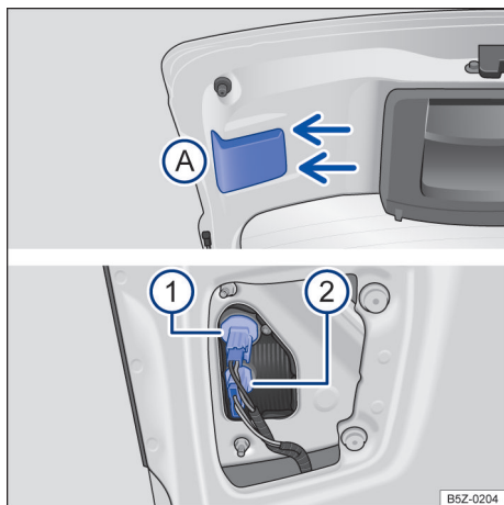
Fig. 125 Lanterna traseira: (A) desinstalar a cobertura e ❶ e ❷ desinstalar as lâmpadas.
