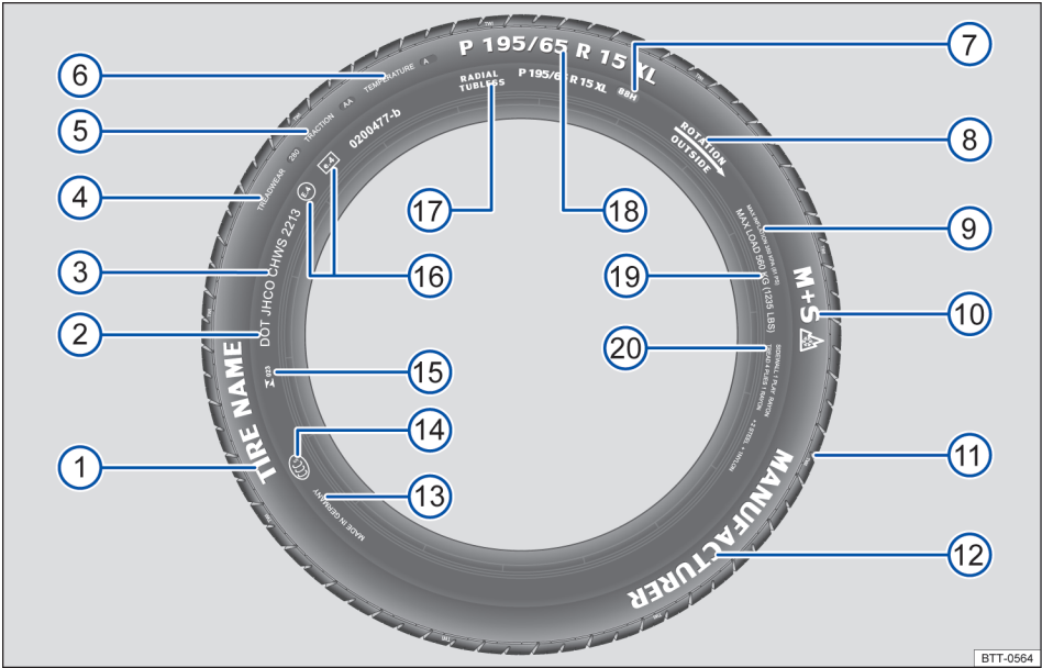
Fig. 158 Inscrição dos pneus internacional (exemplo).
