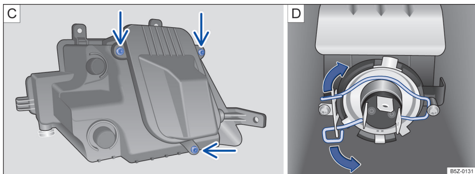
Fig. 122 No para-choque dianteiro: (C) retirar os parafusos da cobertura da lâmpada e (D) lâmpada do farol de neblina.
