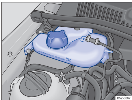
Fig. 151 No compartimento do motor: reservatório de gasolina para o sistema de partida a frio para motores 1.6 (válido somente para o motor CCRA).
