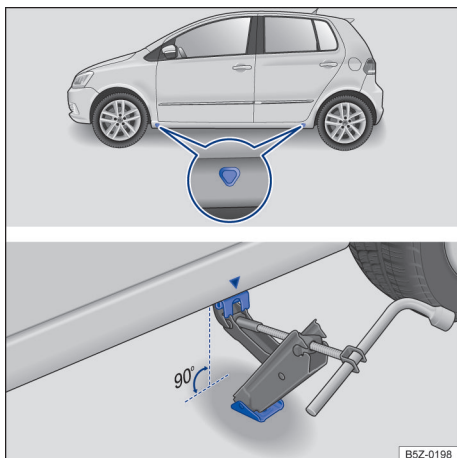
Fig. 162 Pontos de apoio do macaco e macaco posicionado no lado esquerdo traseiro do veículo.
