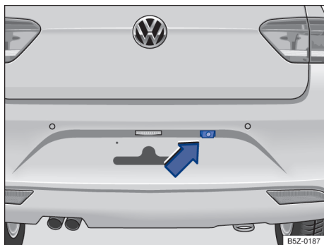
Fig. 93 No para-choque traseiro: local de instalação do assistente de condução em marcha a ré.
