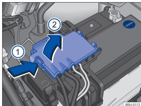
Fig. 134 Compartimento do motor: acesso ao terminal positivo da bateria.
