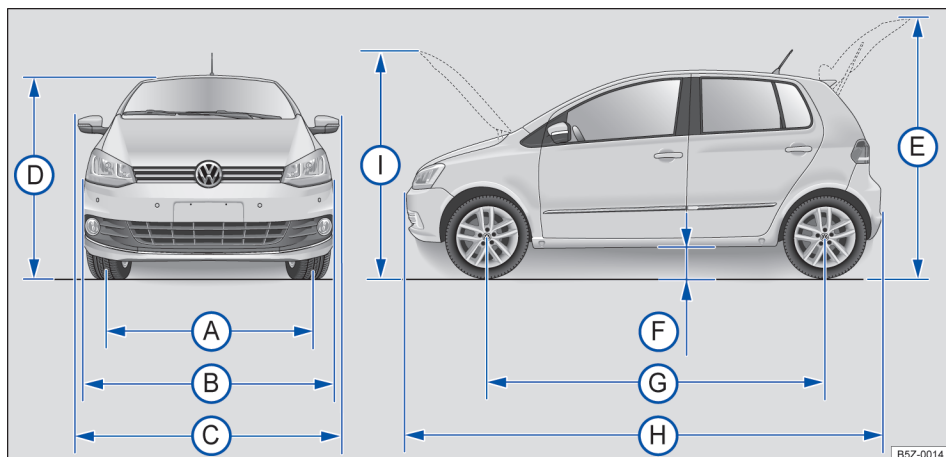
Fig. 171 Dimensões.
