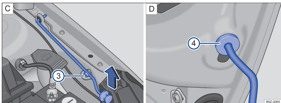
Fig. 143 C: haste de sustentação da tampa do compartimento do motor (3). D: tampa do motor protegida com a haste de sustentação da tampa (4).
