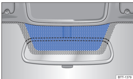
Fig. 75 Para-brisa reticulado com janela de comunicação (superfície azul).
