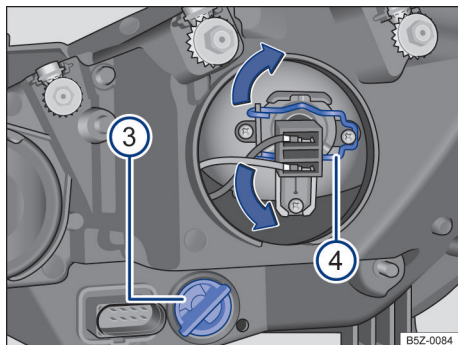
Fig. 119 No compartimento do motor: vista traseira do farol dianteiro direito sem cobertura de borracha: (3) indicadores de direção e (4) farol baixo.
