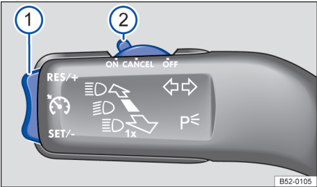
Fig. 88 À esquerda na coluna da direção: alavanca de operação do GRA.
