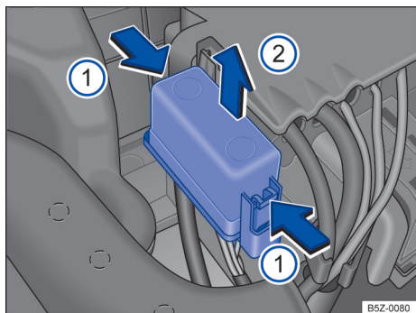
Fig. 129 No compartimento do motor: retirar cobertura da caixa de fusíveis.
