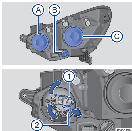
Fig. 118 No compartimento do motor: vista traseira do farol dianteiro direito com cobertura de borracha (esquerda): (A) farol alto e luz de posição, (B) indicadores de direção e (C) farol baixo. Vista traseira do farol dianteiro direito sem cobertura de borracha (direita): (1) farol alto, (2) luz de posição.
