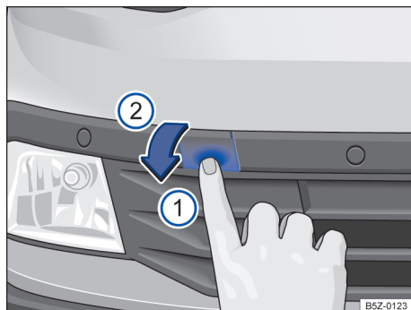
Fig. 138 No para-choque dianteiro à direita: soltar e remover a cobertura.
