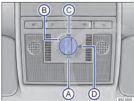
Fig. 59 No revestimento do teto: interruptor rotativo do teto solar.
