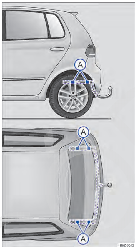
Fig. 128 Pontos de fixação para instalar um dispositivo de reboque posteriormente.
