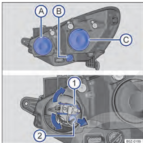
Fig. 136 No compartimento do motor: vista traseira do farol dianteiro direito com cobertura de borracha (esquerda): (A) farol alto e luz de posição, (B) indicadores de direção e (C) farol baixo. Vista traseira do farol dianteiro direito sem cobertura de borracha (direita): (1) farol alto, (2) luz de posição.
