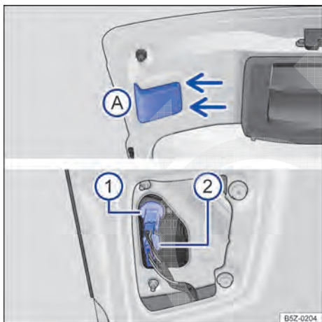
Fig. 143 Lanterna traseira: A desinstalar a cobertura e 1 e 2 desinstalar as lâmpadas.
