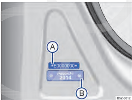
Fig. 187 Na coluna da porta dianteira direita: etiqueta com o número de identificação do veículo parcial (A) e etiqueta de identificação do ano de fabricação (B).
