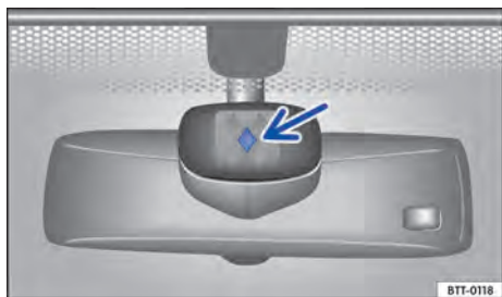
Fig. 76 No para-brisa: superfície sensível do sensor de chuva.
