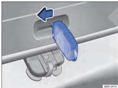
Fig. 57 Do lado de dentro do compartimento de bagagem: destravamento de emergência da tampa traseira.
