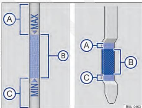
Fig. 164 Vareta de medição do óleo com marcas de nível do óleo do motor.
