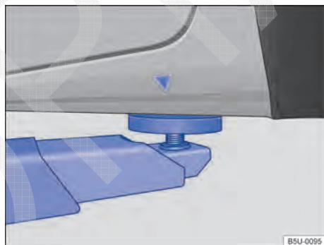
Fig. 184 Pontos de apoio traseiros para a suspensão com plataforma elevatória ou com macaco.
