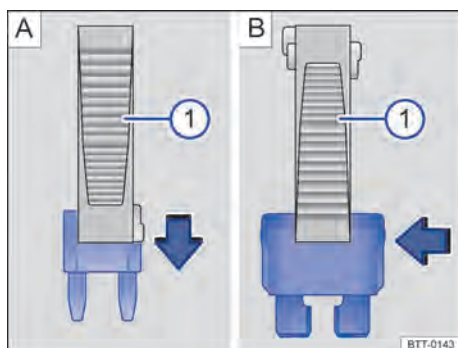
Fig. 152 Remover ou instalar um fusível com a garra da pinça de plástico ①.
