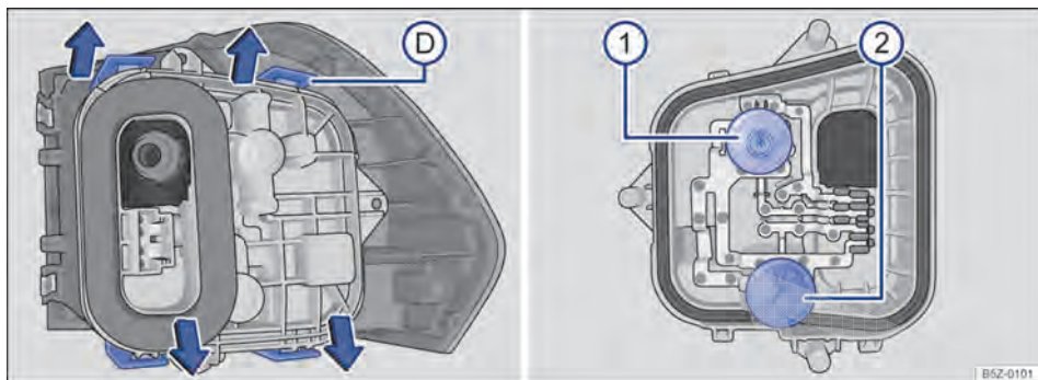
Fig. 142 Lanterna traseira: D desinstalar o suporte das lâmpadas e 1 e 2 desinstalar as lâmpadas incandescentes.
