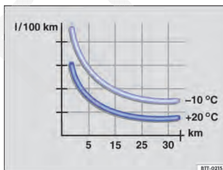
Fig. 91 Consumo de combustível em l/100 km em 2 temperaturas ambiente diferentes.
