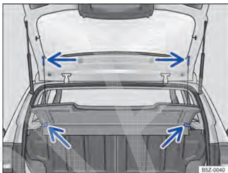
Fig. 125 No compartimento de bagagem: remover e instalar a cobertura do compartimento de bagagem.
