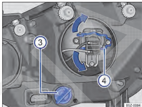
Fig. 137 No compartimento do motor: vista traseira do farol dianteiro direito sem cobertura de borracha: (3) indicadores de direção e (4) farol baixo.
