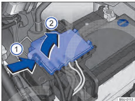
Fig. 153 Compartimento do motor: acesso ao terminal positivo da bateria.
