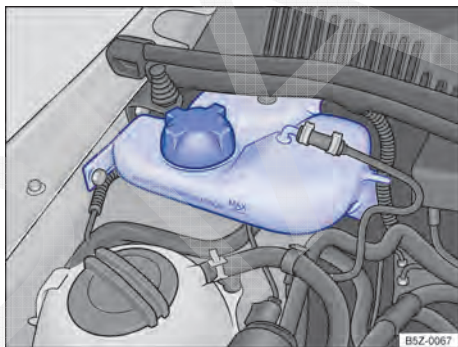
Fig. 170 No compartimento do motor: reservatório de gasolina para o sistema de partida a frio para motores 1.6 (válido somente para o motor CCRA).
