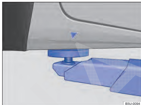
Fig. 183 Pontos de apoio dianteiros para a suspensão com plataforma elevatória ou com macaco.
