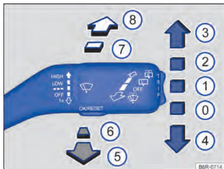
Fig. 74 Comandar os limpadores / lavadores do para-brisa e o limpador / lavador do vidro traseiro.
