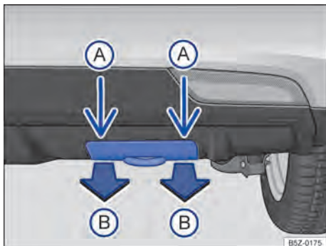
Fig. 160 No para-choque traseiro à direita: argola de reboque traseira - para-choque com cobertura removível. ►
