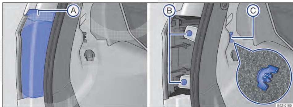
Fig. 141 Lateralmente no compartimento de bagagem: (A) desinstalar a cobertura, (B) retirar os dois parafusos e (C) retirar o parafuso borboleta (lupa).
