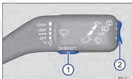
Fig. 38 Veículos sem volante multifunções: tecla 1 na alavanca dos limpadores dos vidros para confirmação dos itens de menu e chave 2 para alternar entre os menus.
