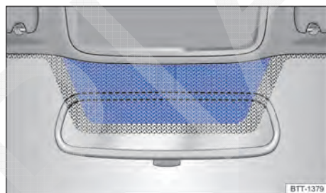
Fig. 82 Para-brisa reticulado com janela de comunicação (superfície azul).
