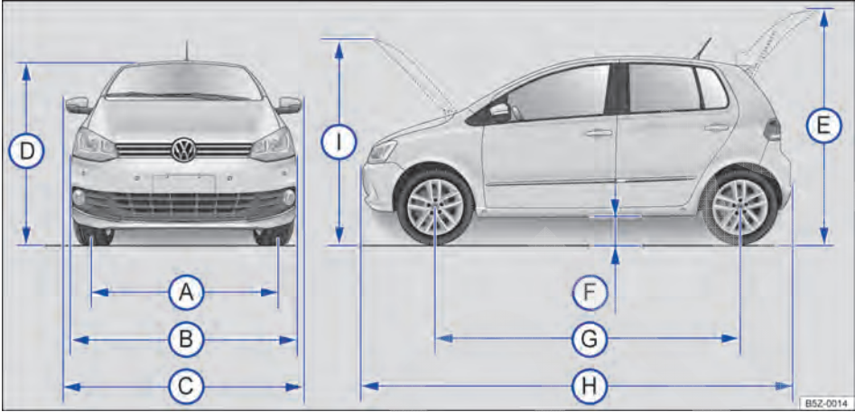
Fig. 190 Dimensões.
