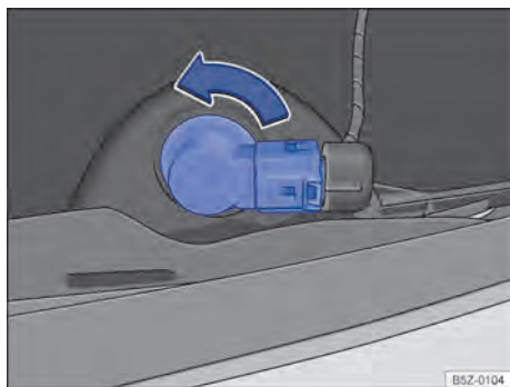
Fig. 144 Atrás do para-choque traseiro: acesso à lâmpada incandescente da lanterna de neblina (somente lado esquerdo).
