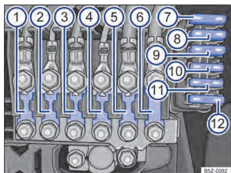
Fig. 150 Caixa de fusíveis.
