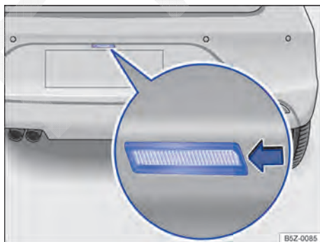
Fig. 145 No para-choque traseiro: remover a lanterna da placa de licença.
