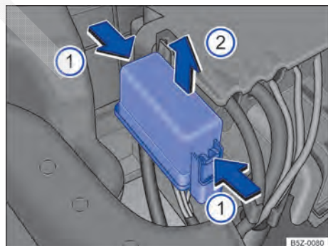
Fig. 148 No compartimento do motor: retirar cobertura da caixa de fusíveis.
