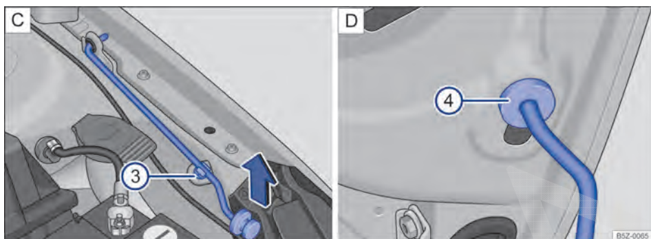
Fig. 162 C: haste de sustentação da tampa do compartimento do motor (3). D: tampa do motor protegida com a haste de sustentação da tampa (4).
