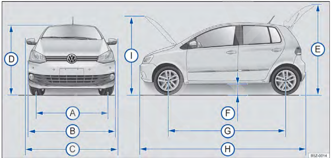
Fig. 19 Dimensões.
