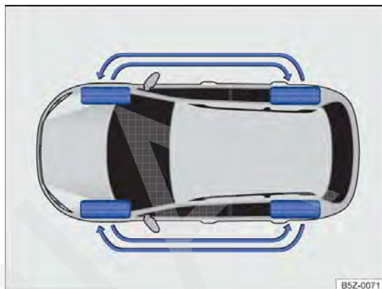
Fig. 140 Esquema para a troca das rodas.
