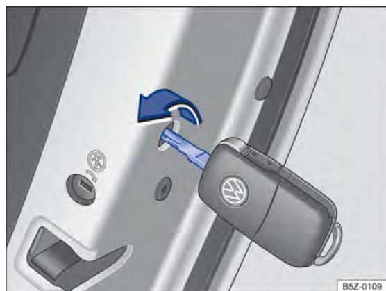
Fig. 156 Travação de emergência do veículo com a chave do veículo.
