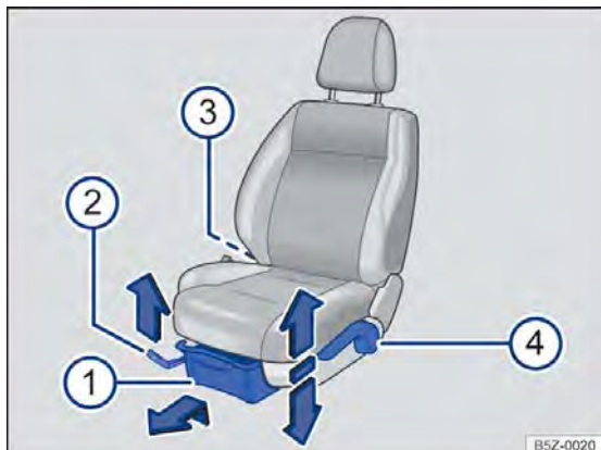
Fig. 37 Comandos do banco dianteiro esquerdo.
