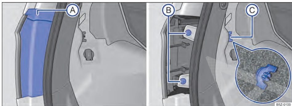
Fig. 177 Lateralmente no compartimento de bagagem: (A) desinstalar a cobertura, (B) retirar os dois parafusos e (C) retirar o parafuso borboleta (lupa).
