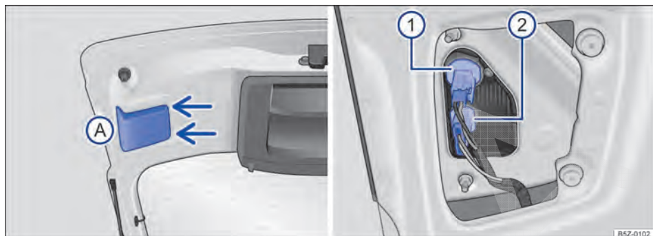
Fig. 179 Lanterna traseira: A desinstalar a cobertura e ① e ② desinstalar as lâmpadas.
