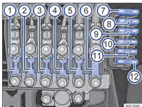
Fig. 171 Caixa de fusíveis.
