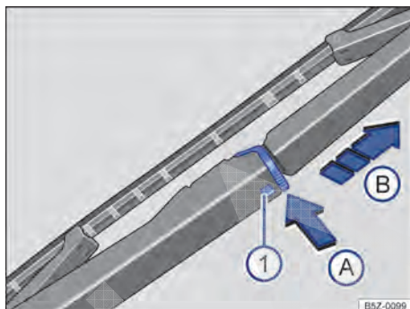
Fig. 137 Substituir a palheta do limpador do vidro traseiro.
