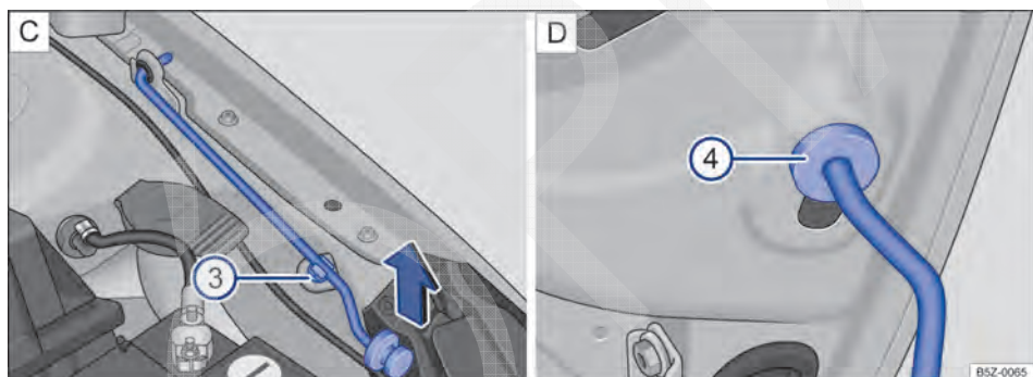
Fig. 126 C: haste de sustentação da tampa do compartimento do motor (3). D: tampa do motor protegida com a haste de sustentação da tampa (4).
