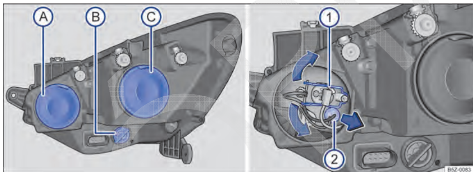
Fig. 172 No compartimento do motor: vista traseira do farol dianteiro direito com cobertura de borracha (esquerda): (A) farol alto e luz de posição, (B) indicadores de direção e (C) farol baixo. Vista traseira do farol dianteiro direito sem cobertura de borracha (direita): ① farol alto, ② luz de posição
