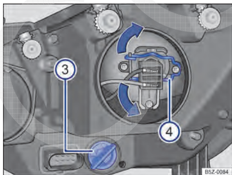
Fig. 173 No compartimento do motor: vista traseira do farol dianteiro direito sem cobertura de borracha: ③ indicadores de direção e ④ farol baixo.
