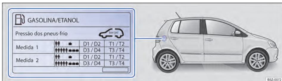
Fig. 140 Na parte interna da portinhola do tanque de combustível: etiqueta com a pressão dos pneus.
