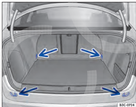
Fig. 102 No compartimento de bagagem: olhais de amarração.
