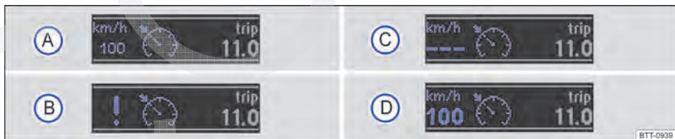
Fig. 166 No display do instrumento combinado: indicadores de status do GRA.
