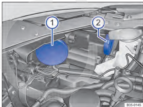
Fig. 240 No compartimento do motor: cobertura para lâmpadas com descarga de gás ❶, farol de conversão, farol de rodagem diurna, luz de posição e indicador de direção ❷.
