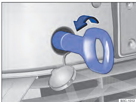
Fig. 256 No para-choque dianteiro à direita: rosquear a argola de reboque.
