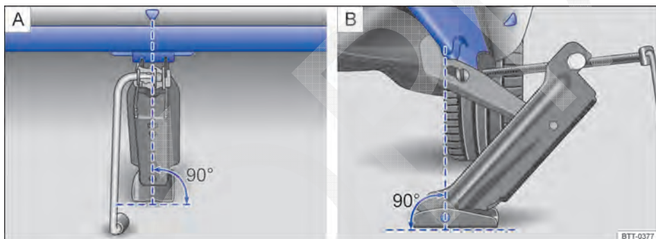
Fig. 231 Macaco posicionado no lado esquerdo traseiro do veículo.
