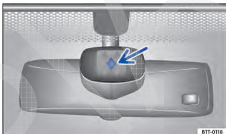
Fig. 93 No lado interno do para-brisa, na parte superior do espelho interno: superfície sensível do sensor de chuva e de luz.
