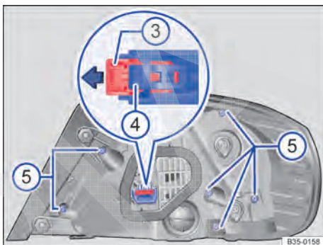
Fig. 249 desinstalar o suporte das lâmpadas.
