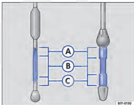
Fig. 195 No compartimento do motor: vareta de medição do óleo com marca de nível do óleo do motor.
