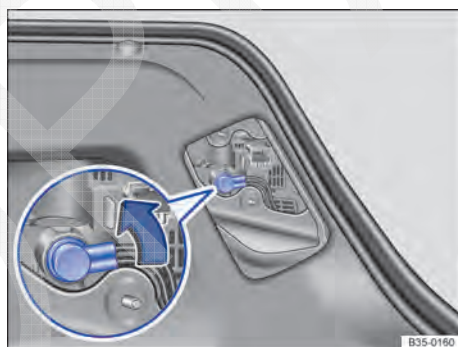
Fig. 247 Na tampa do compartimento de bagagem: desinstalar o suporte da lâmpada.
