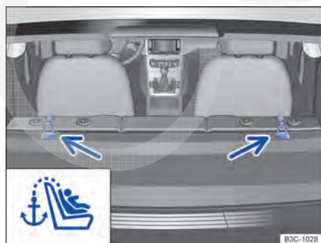
Fig. 82 Olhais de fixação para o assento externo na superfície atrás do banco traseiro.
