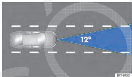
Fig. 172 Área de cobertura do sensor do radar.
