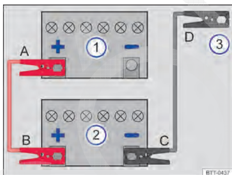
Fig. 253 Esquema para a conexão dos cabos auxiliares de partida em veículos auxiliares de partida sem sistema Start-Stop ou função de retorno de energia: bateria do veículo descarregado ① e bateria do veículo fornecedora de corrente ②.
