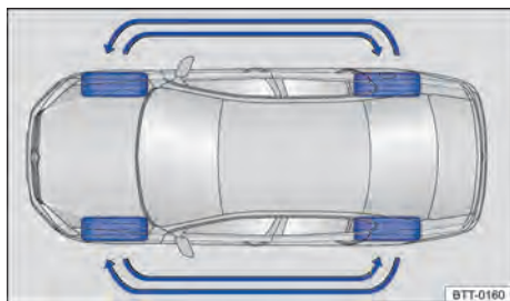
Fig. 204 Esquema para a troca das rodas.
