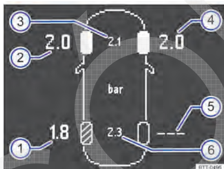
Fig. 182 Representação esquemática da exibição do display do instrumento combinado: pressões dos pneus atuais.
