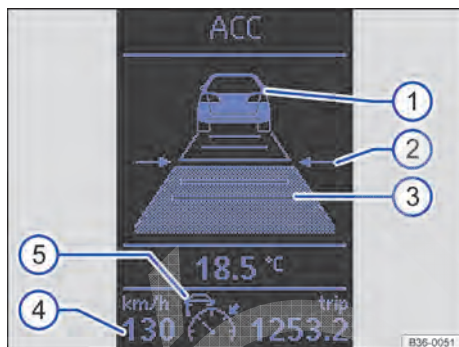
Fig. 168 No display do instrumento combinado: ACC ativo, veículo à frente reconhecido, distância regulada.
