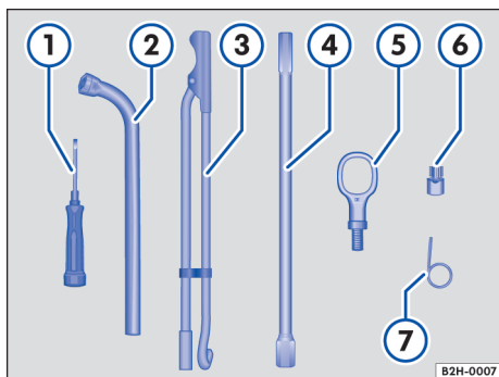
Fig. 144 Componentes das ferramentas de bordo.
