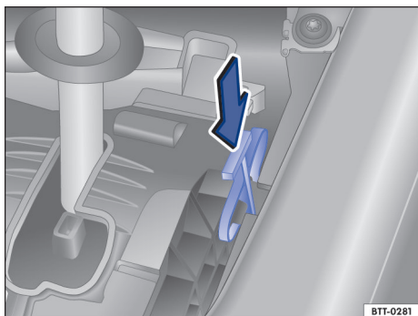
Fig. 106 destravar emergencialmente o bloqueio da alavanca seletora.
