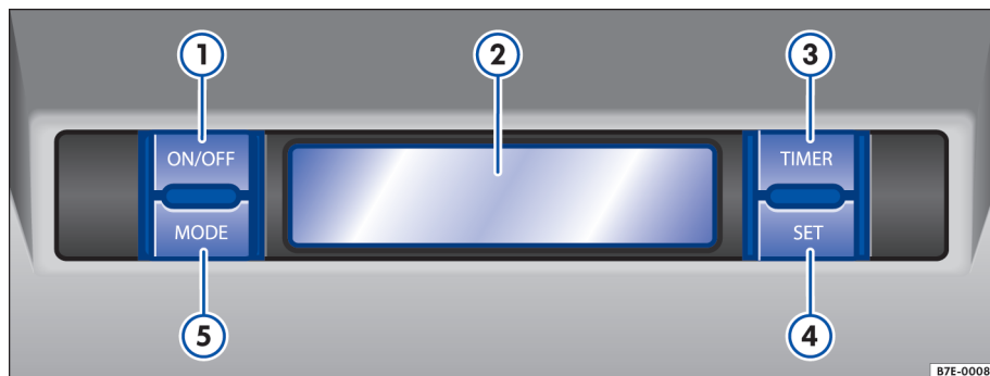
Fig. 93 No revestimento do teto: elementos de comando do aquecimento estacionário.
