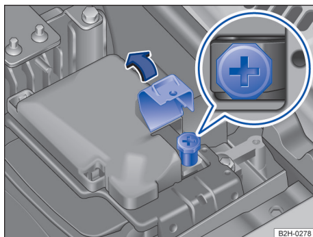
Fig. 164 No compartimento do motor: polo positivo do ponto de auxílio à partida.
