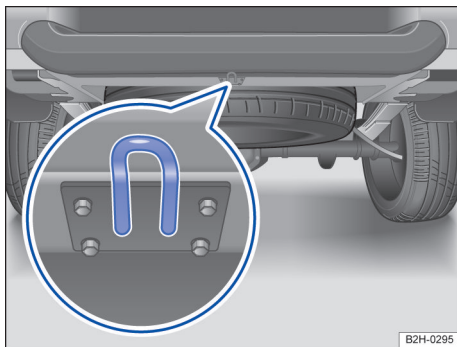
Fig. 166 Abaixo do para-choque: argola de reboque em veículos sem dispositivo de reboque de fábrica.
