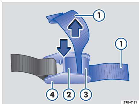
Fig. 133 Apertar o cinto de retenção.
