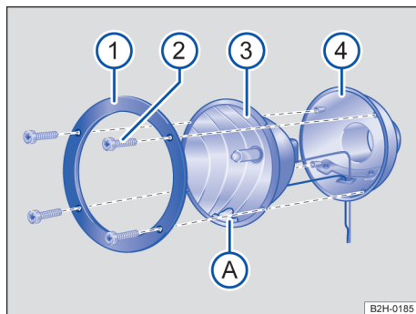
Fig. 157 Iluminação adicional no teto do veículo: desinstalar o vidro da lâmpada.
