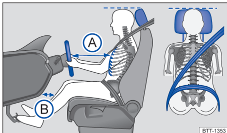
Fig. 18 Representação esquemática: distância correta do condutor em relação ao volante, posição correta do caderço do cinto de segurança e ajuste correto do apoio para cabeça.
