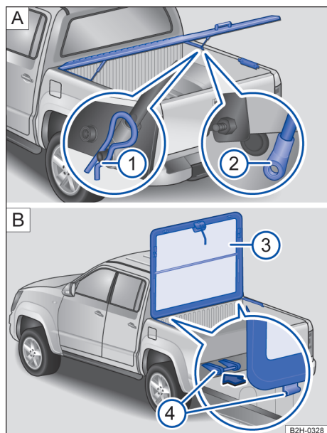
Fig. 54 Instalar e desinstalar a cobertura do compartimento de carga de alumínio.
