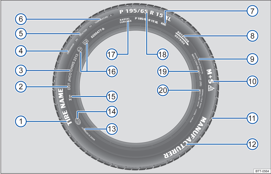
Fig. 193 Inscrição internacional dos pneus.
