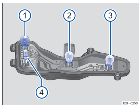
Fig. 152 Suporte da lâmpada: ① indicadores de direção, ②, lanterna traseira, ③ lanterna de freio, ④ Dependendo da versão, lanterna de marcha a ré ou suporte da lâmpada à direita lanterna de marcha a ré e suporte da lâmpada à esquerda lanterna de neblina.
