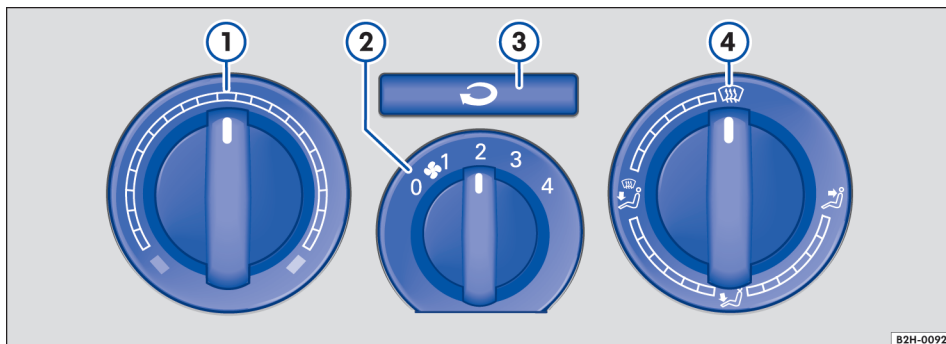
Fig. 91 No painel de instrumentos: elementos de comando do sistema de ventilação e aquecimento.
