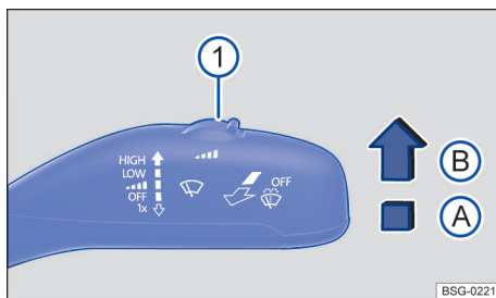
Fig. 84 À direita da coluna de direção: alavanca dos limpadores do para-brisa.
