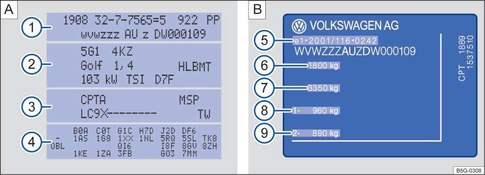
Fig. 206 (A) Etiqueta de dados do veículo: na figura de exemplo com o código do motor CPTA (3). (B): plaqueta de identificação.
