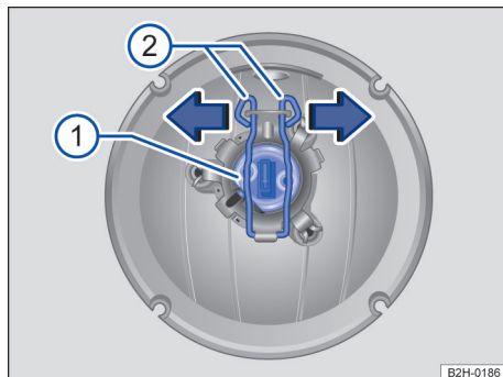
Fig. 158 Iluminação adicional no teto do veículo: trocar a lâmpada incandescente.
