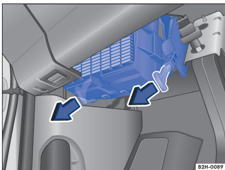
Fig. 159 Caixa de fusíveis abaixo do painel de instrumentos.
