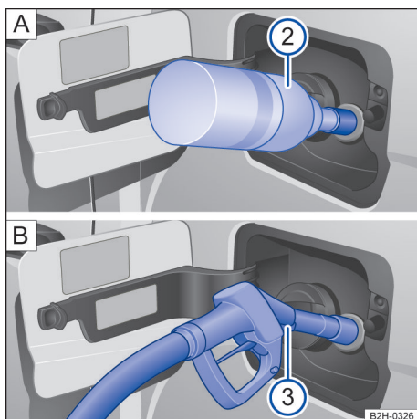
Fig. 143 Atrás da portinhola do tanque: abastecer AdBlue com o frasco de reabastecimento ou [A] com a bomba de combustível [B].
