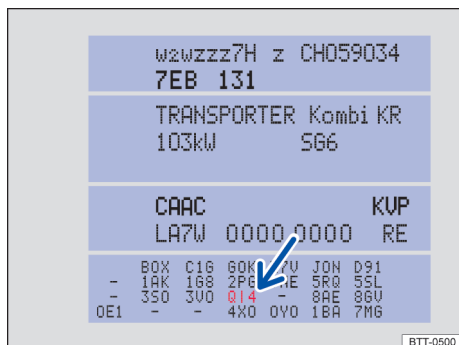
Fig. 204 Etiqueta de dados do veículo com número PR do respectivo serviço (Representação esquemática).
