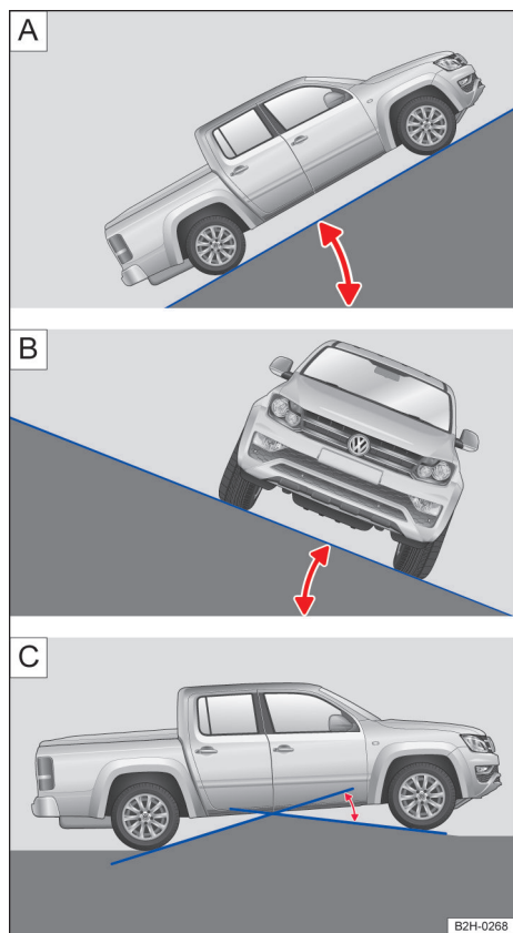
Fig. 109 Representação da rampa máxima [A], ângulo de inclinação [B] e ângulo de rampa [C].
