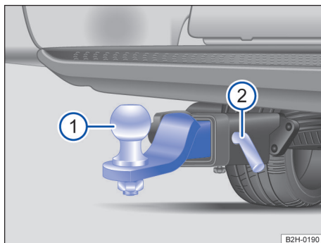
Fig. 137 Sob o para-choque traseiro: montar a rótula de engate.
