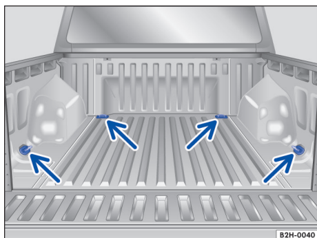
Fig. 130 No compartimento de carga: olhais de amarração.
