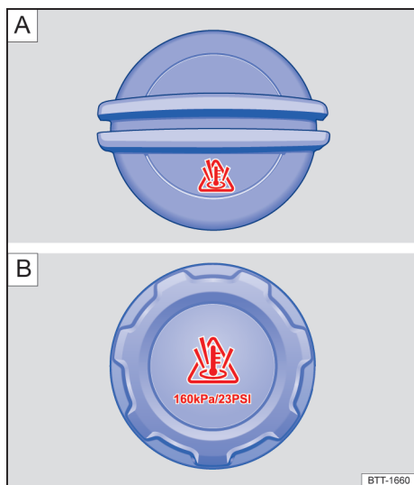
Fig. 178 No compartimento do motor: tampa do reservatório de expansão do líquido de arrefecimento (variante (A) ou (B)).
