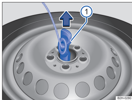
Fig. 191 Roda sobressalente ou roda de emergência: soltar o suporte dos aros.
