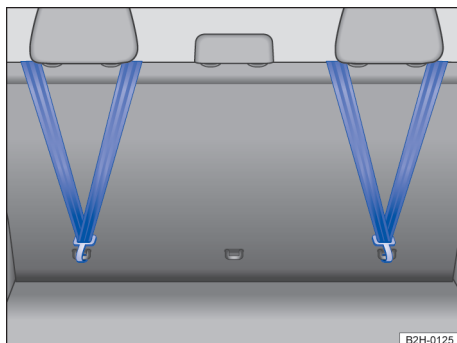
Fig. 45 Na parte traseira do encosto do banco traseiro: cinto de fixação superior preso.
