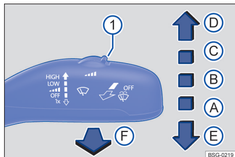
Fig. 83 À direita da coluna de direção: comandar os limpadores do para-brisa.
