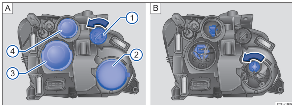
Fig. 147 No compartimento do motor: coberturas no farol esquerdo frontal. 1 Indicadores de direção, 2 farol alto e farol de rodagem diurna, 3 farol baixo, 4 luz de posição.
