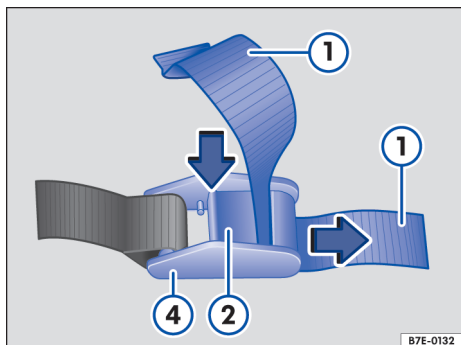
Fig. 134 Soltar o cinto de retenção.
