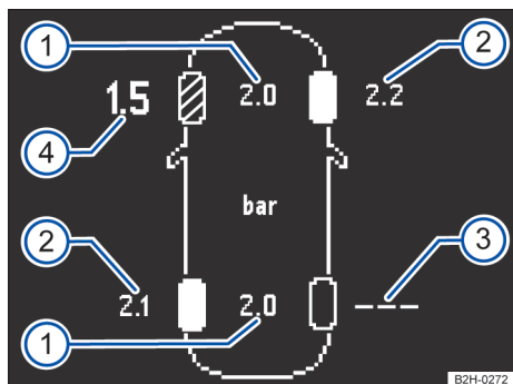
Fig. 182 Representação esquemática do indicador do display do instrumento combinado: pressões dos pneus atuais.
