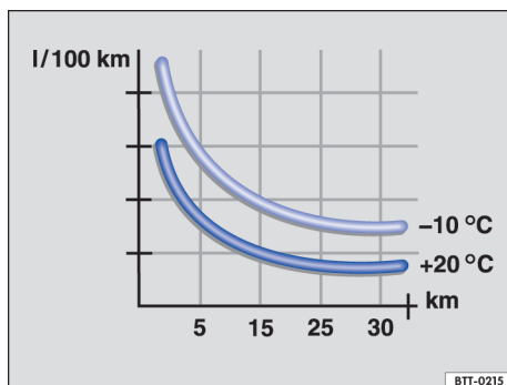
Fig. 98 Consumo de combustível em l/100 km em duas temperaturas ambiente diferentes.
