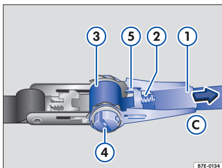
Fig. 136 Apertar o cinto de catraca.
