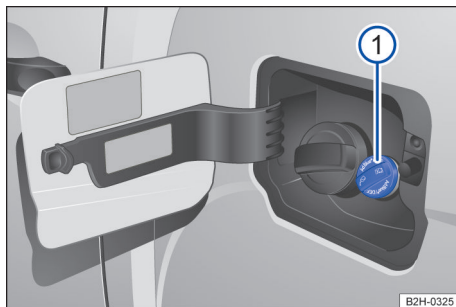
Fig. 142 Atrás da portinhola do tanque: tampa do tanque para AdBlue.
