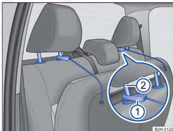
Fig. 44 Banco traseiro: fixar a superfície do banco nos apoios para cabeça.
