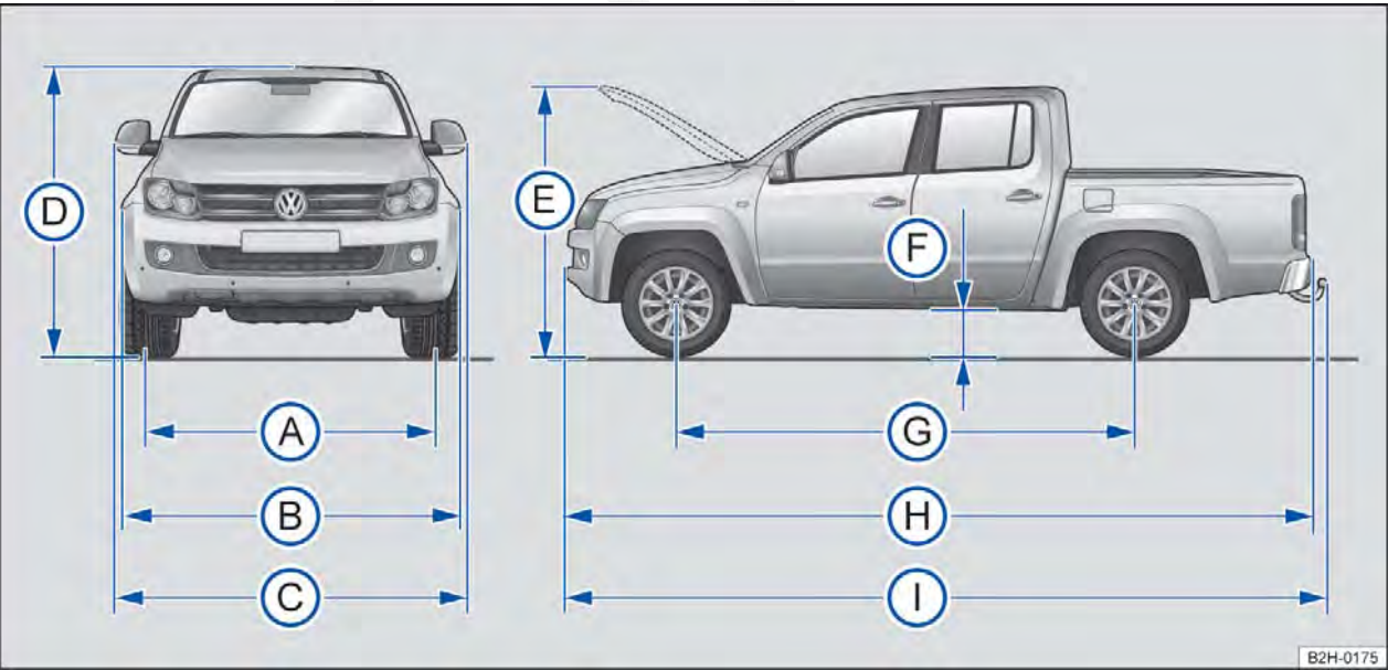
Fig. 18 Dimensões.
