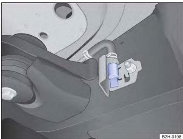
Fig. 129 Drenar o filtro de combustível: bujão de drenagem na parte inferior do veículo, na longitudinal no lado esquerdo do veículo.
